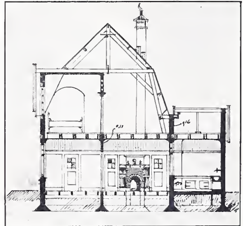
DWARSDOORSNEDE.
