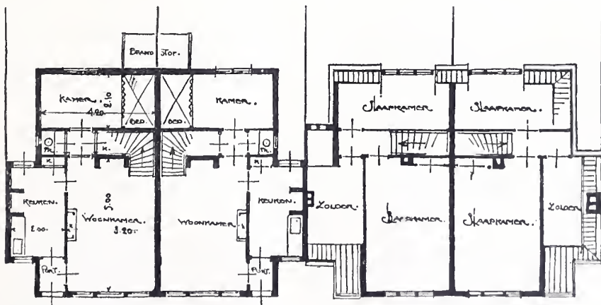
BEGANE GROND.
