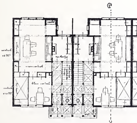
BEGANEGROND.
