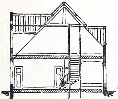
DWARSDOORSNEDE.
