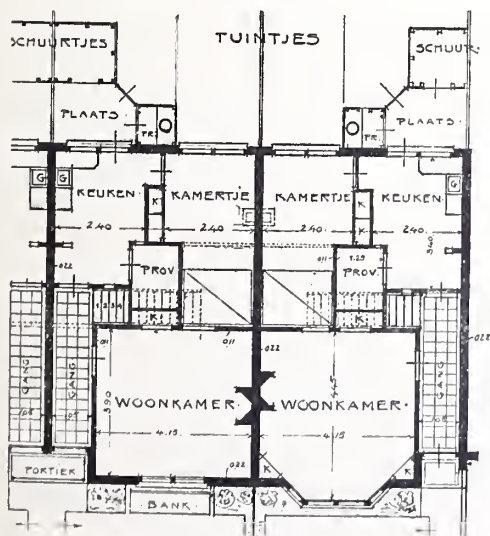
BEGANEGROND.
