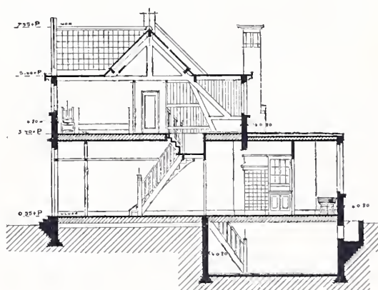
DWARSDOORSNEDE.
