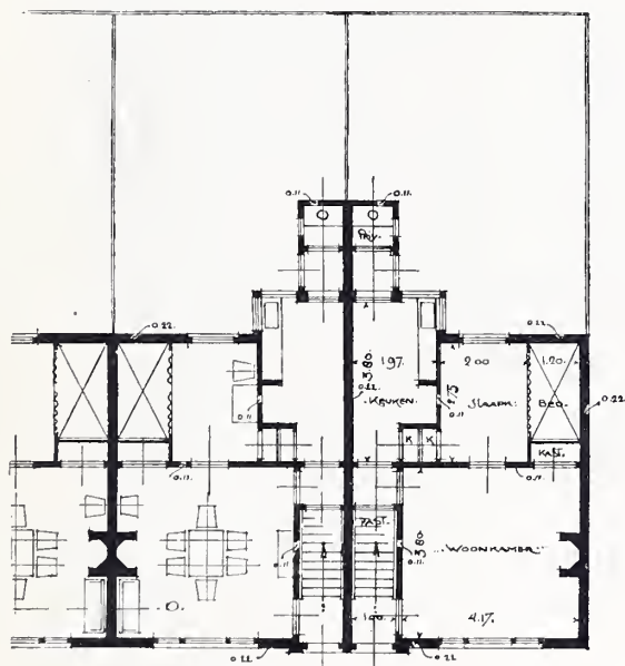
BEGANE GROND.
