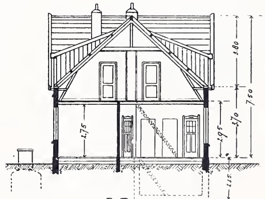
DOORSNED E A-B.
