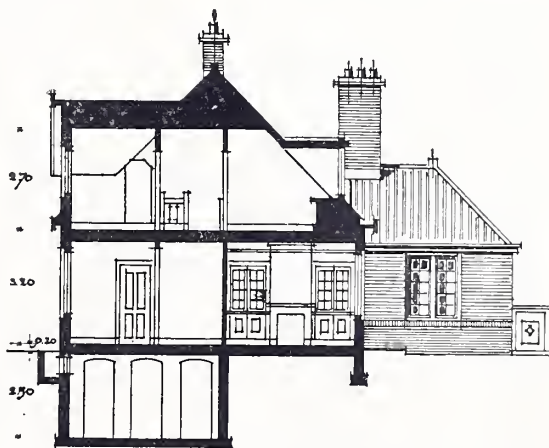
DWARS DOORSNEDE.
