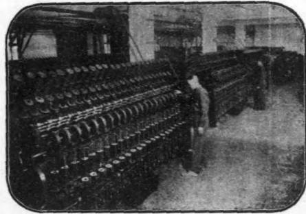
本公司第一分廠又錠機之一
