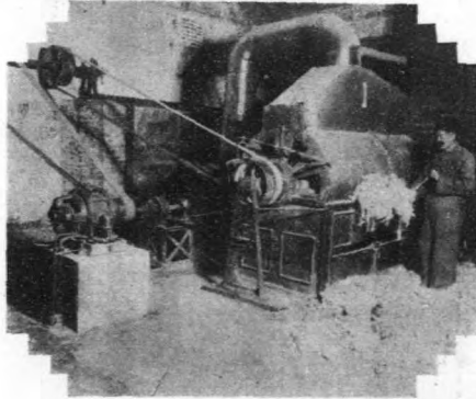
● 打土 ● 將毛所含壹部分 塵沙等不潔之物 除去備易於洗滌
