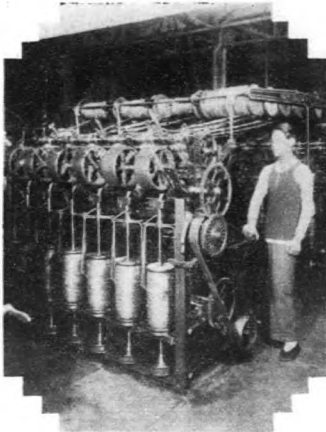
● 二道煉 條機 ● 併數毛條 為一條使 之成為更 進一步之 相當重量 與細度
