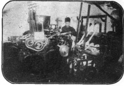
雙筒機之一部分
