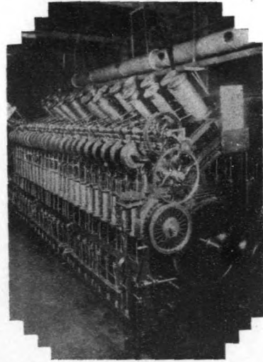
● 精煉機 ● 精煉毛條為線 胚以備紡績用
