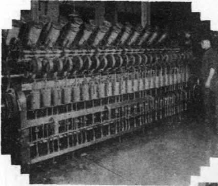
● 叉錠機 ● 將線胚紡績成紗 以供手工針織及 織嗶嘰等用
