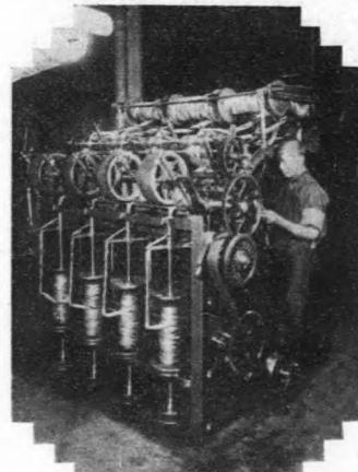
● 頭道煉 條機 ● 併數毛條 為一條並 使至相當 之重量與 細度
