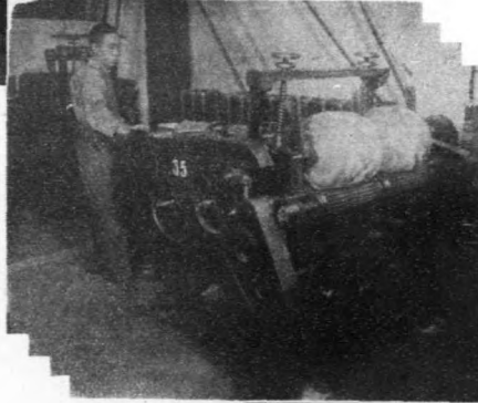
●整理雙球機● 此乃第五次重梳愈 使毛條平行正直並 將毛條作成球狀為 完成之毛條 ↩
