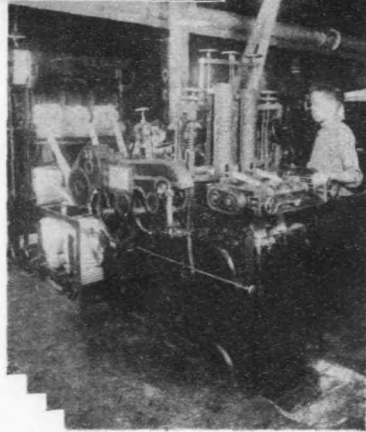
●雙筒機● 此機將毛條作第 六次重梳愈使毛 條平行正直 ↩
