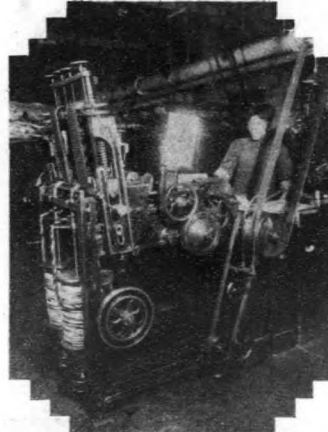
● 雙錠 機 ● 此為第七 次(即末 次)重梳 並為第一 次機器加 撚度於毛 條
