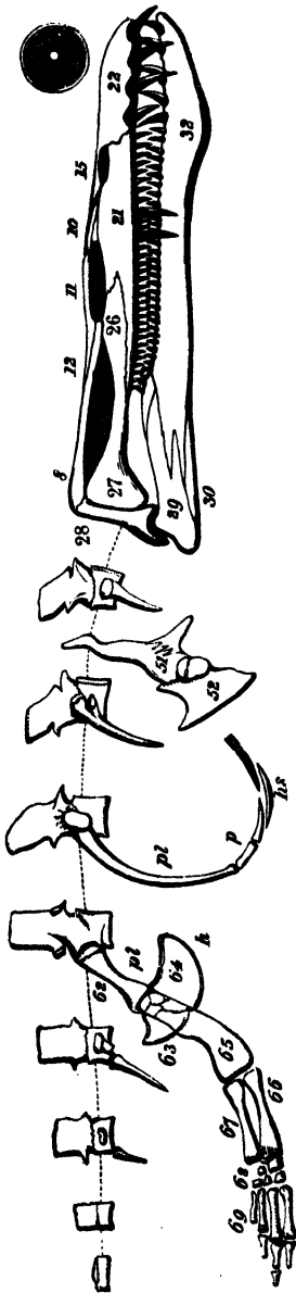
Fig. 90. Nothosaurus (Trias).
