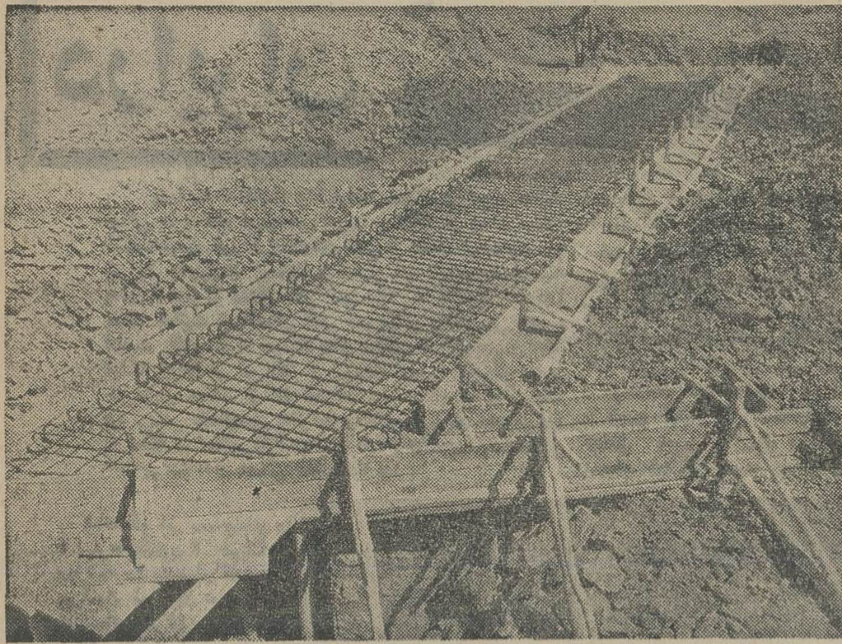
یک بل متوسط در منطقه کوههای الوند که در مسیر راه فرعی توسط شرکت پیروز ساخته میشود
