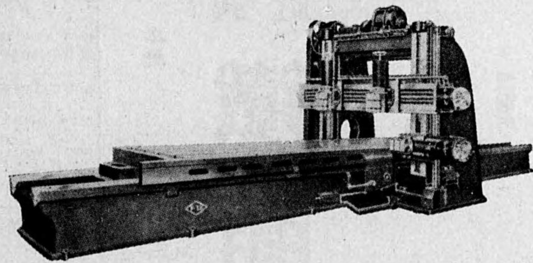
10呎 24呎 電動機直結大形平削盤
