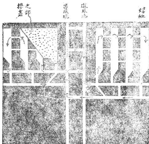
第五圖 房柱法
