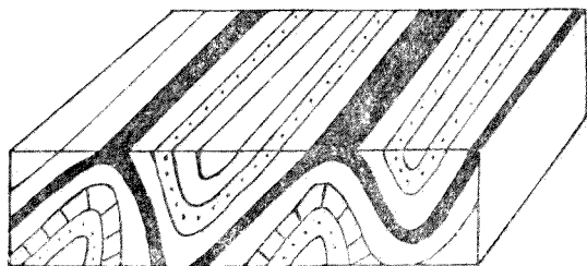
第二圖 地層之褶皺
