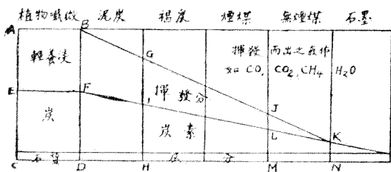
第一圖 碳化作用成分之變遷
