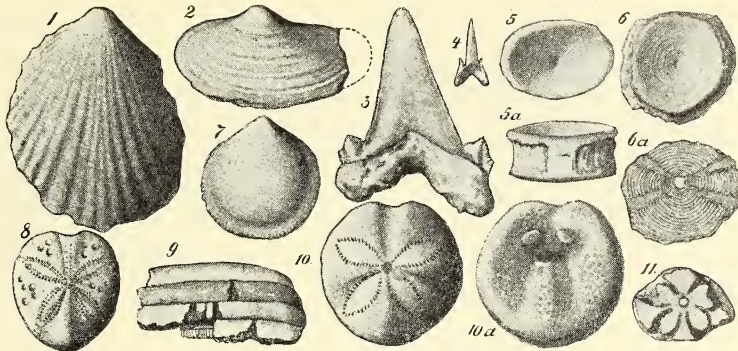
Abb. 5. 1. Ostrea ventilarum Goldf. 2. Panopaea Woodwardi v. Koen. 3. Zahn von Carcharodon angustidens Ag. 4. Zahn von Lamna elegans Ag. 5. Wirbel von Squatina sp. 6. Wirbel von Selache sp. 7. Pectunculus sp. 8. Maretia Grignonensis Desm. 9. Zahnplatten von Aetobates irregularis Ag. 10. Laevipatagus bigibbus Beyr. 11. Wirbel von Torpedo sp.
