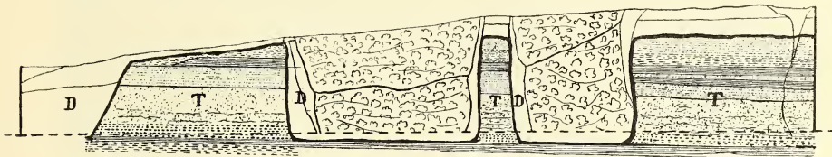
Abb. 9. Profil der Küste bei Sassau nach ZADDACH.
