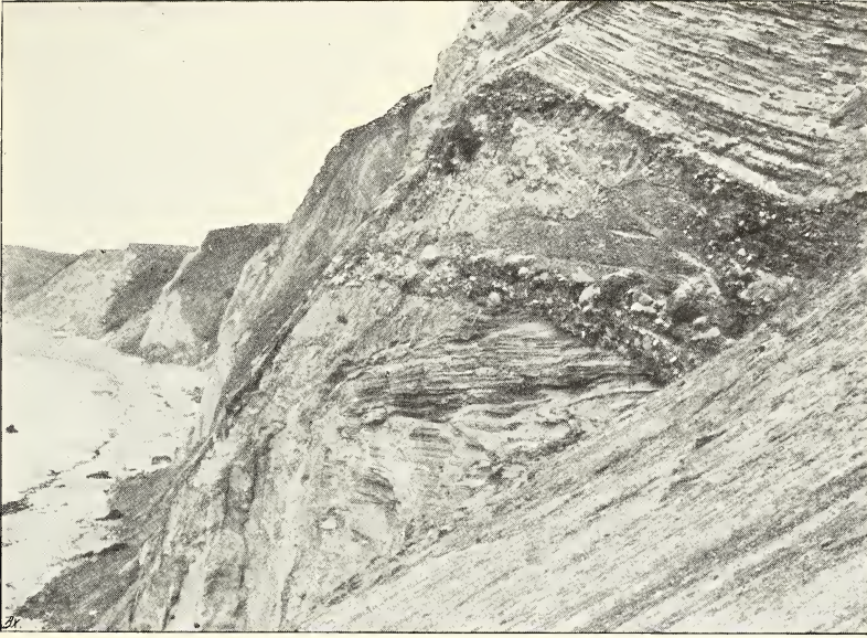
Abb. 13. Diluvialer Sand und Kies an der Marscheiter Spitze. Aufgen. im April 1905.
