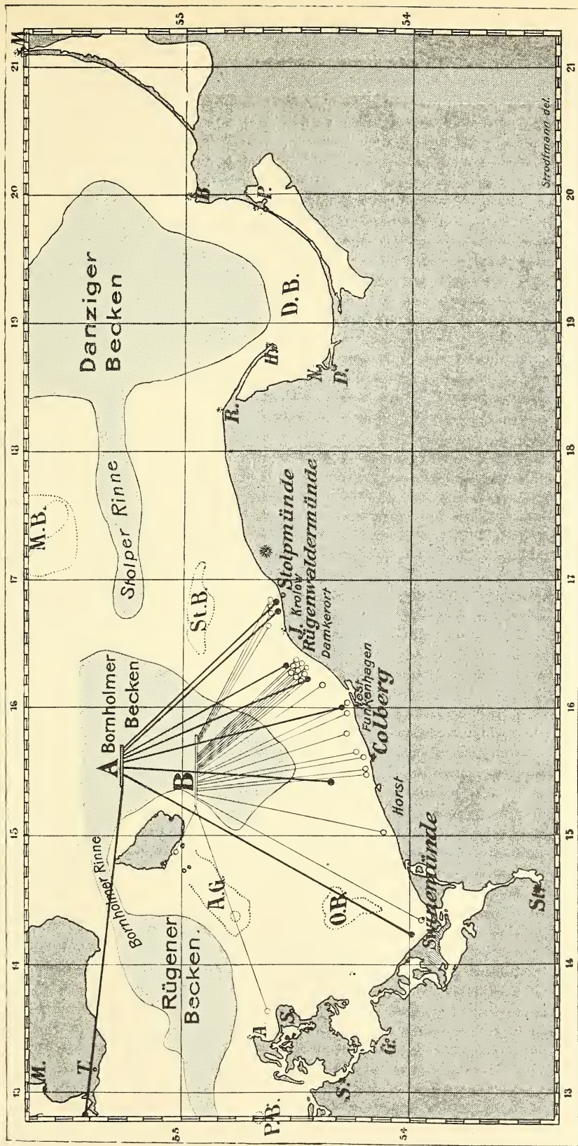
A und B sind die Aussetzstellen markierter Fische im Bornholmer Becken, die Fangorte (Punkte resp. Kreise) sind durch gerade Linien mit den Aussetzstellen verbunden.
