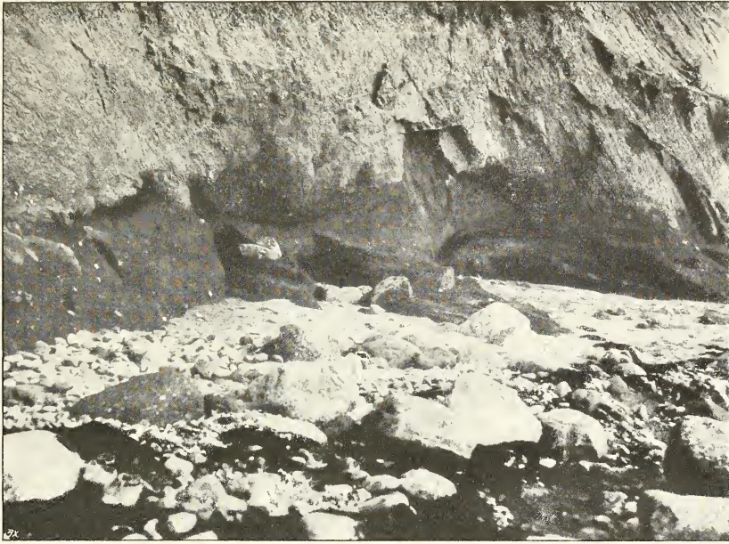
Abb. 40. Durch die Brandung ausgehöhlte Partien am Fuße einer Geschiebemergelwand bei Kreislacken (Strand nur wenige Meter breit). Aufgen. im September 1904.
