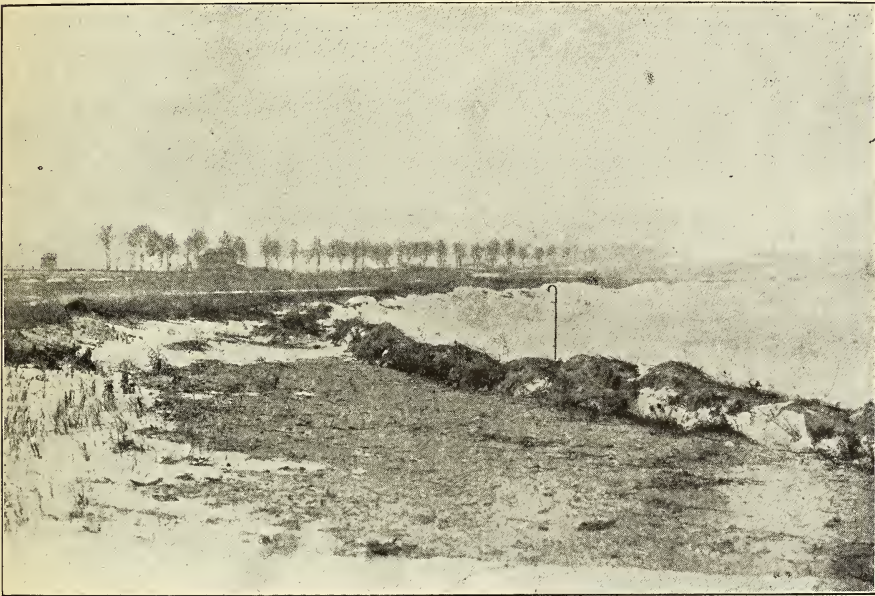
Abb. 1. Durch Eisdruck aufgeschobener Sandwall am Löwentin-See.
