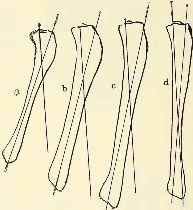
Fig. 8. Umriß-Schemata verschiedener Schienbeine, von innen gesehen a) von einem erwachsenen weiblichen Gorilla, b) von Spy, c) von einem Neolithiker, d) von einem modernen Lütticher. (Nach FRAIPONT, aus Ergebnisse d. Anatomie und Entwicklungsgeschichte. Bd. IX. Wiesbaden 1899.)
