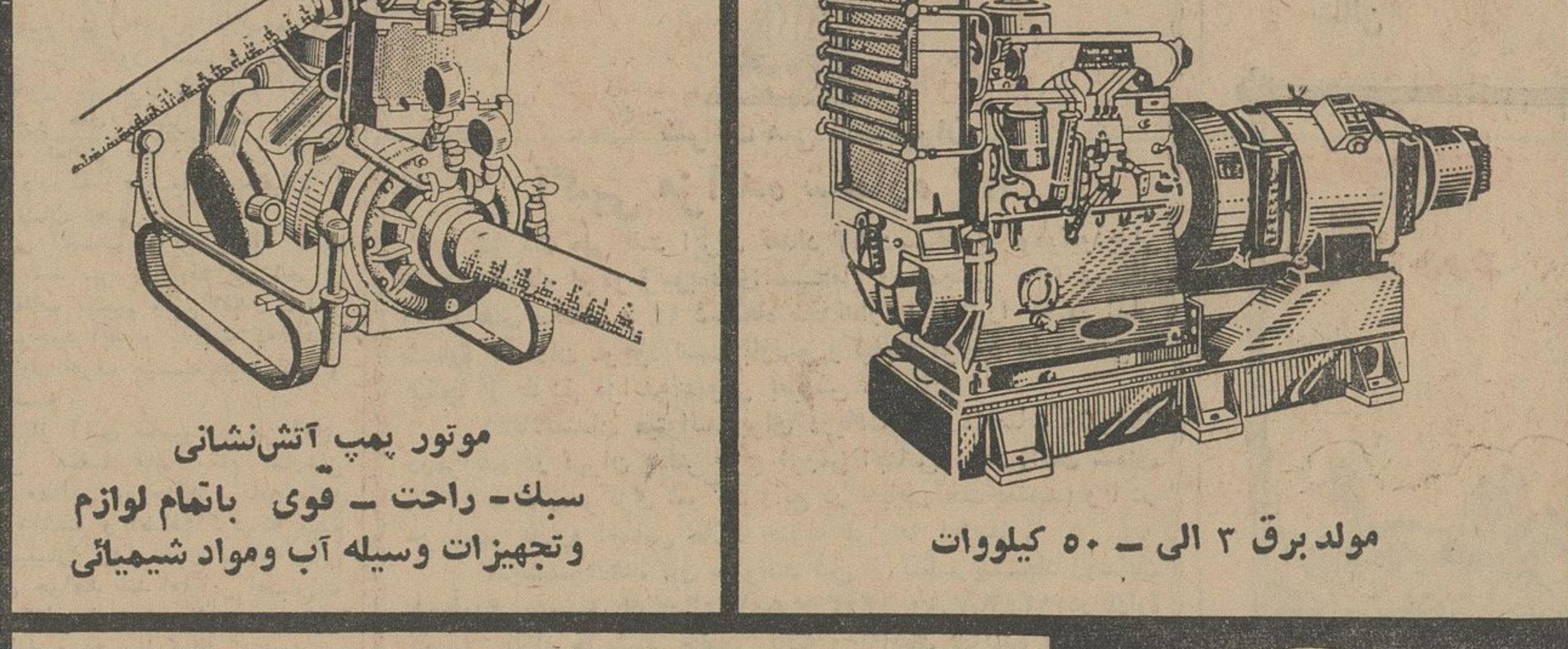
موتور بپ آتش نشانی سبک - راحت - قوی بانام لوازم و تجهیزات وسیله آب و مواد شیمیائی مولد برق ۲ الی - ۵۰ کیلووات
