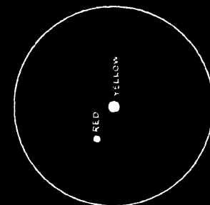
\alpha CASSIOPEIAE
