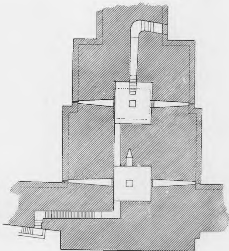
Рис. 172. Верхний подвал.
