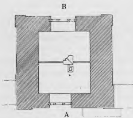
Рис. 272. 1-й этаж.
