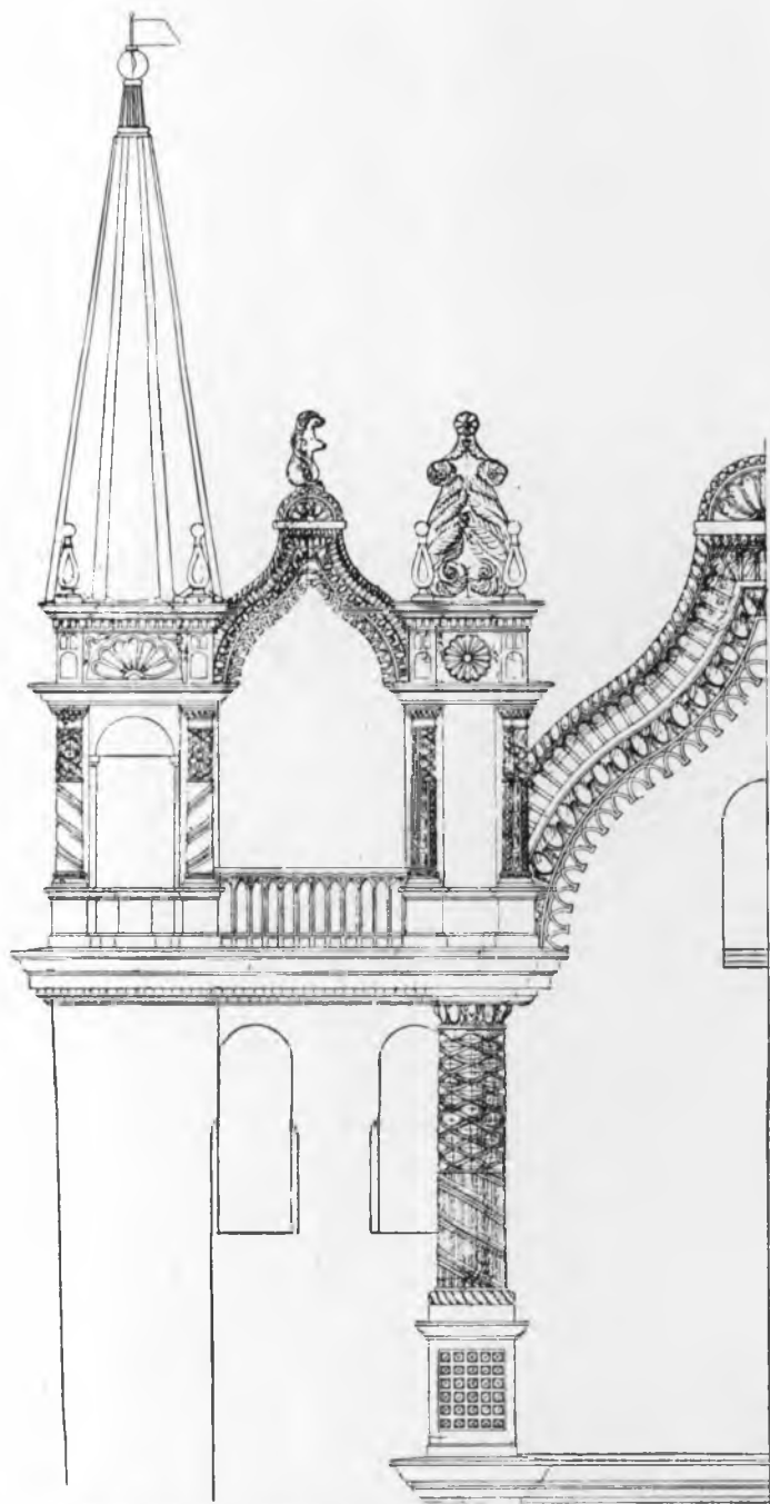
Рис. 133. 6-й этаж. Декоративная обработка лицевых фасадов Спасской башни.
