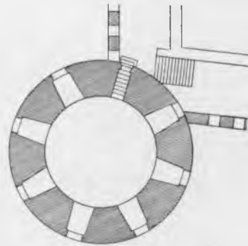
Рис. 254. 2-й этаж.
