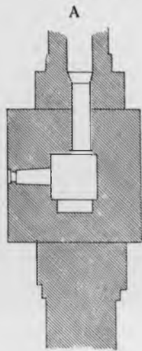
Рис. 286. 1-й этажъ.
