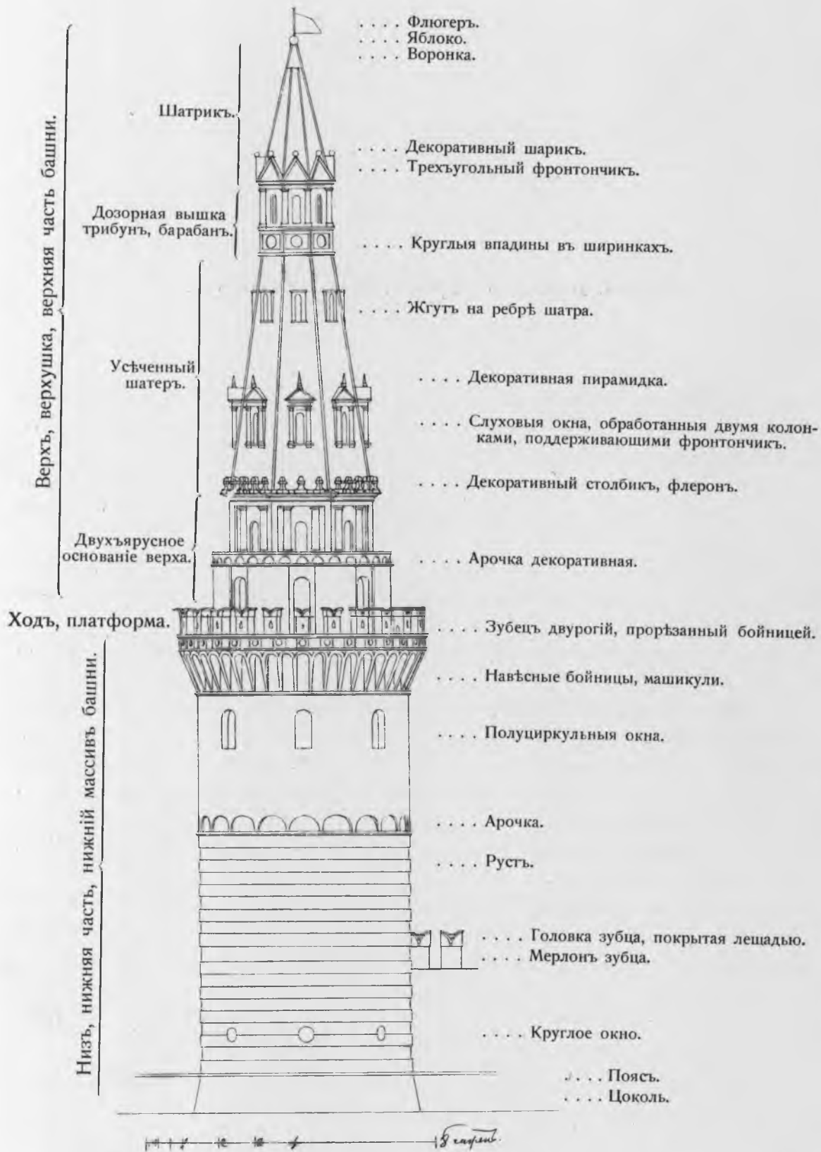
Рис. 114. Названія архитектурныхъ частей башенъ.
