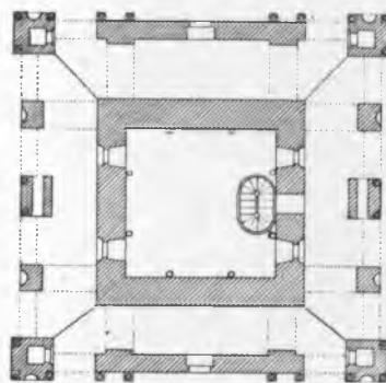
Рис. 127. 7-й этаж.
