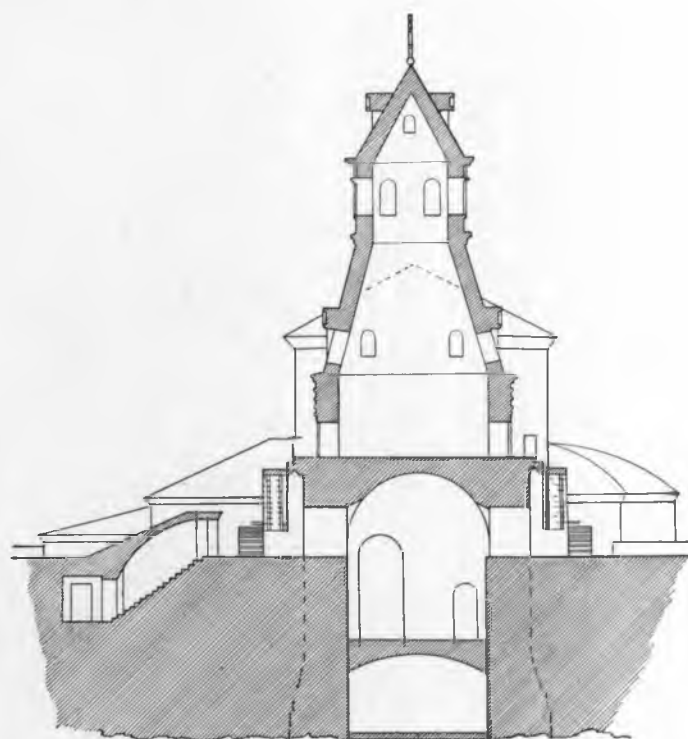
Рис. 341. Разрѣзь по линіи А В.
