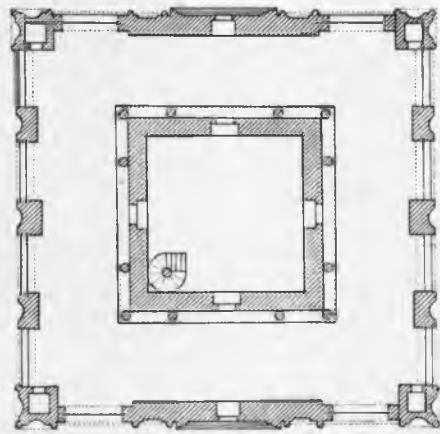
Рис. 177. 5-й этаж.
