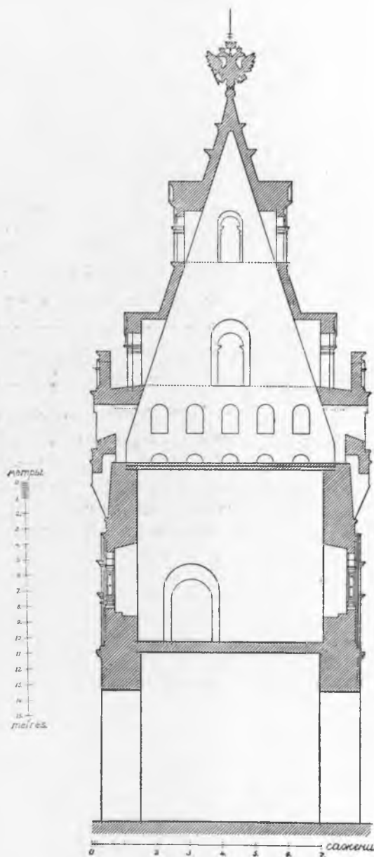
Рис. 72. Гербовая башня.
