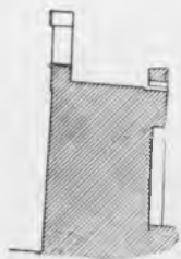
Рис. 84. Разрѣзъ стѣны между 1-й Безымянной и Тайницкой башнями.
