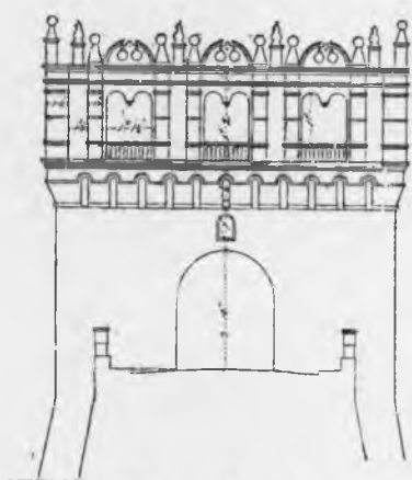
Рис. 181. Фасадъ Кутафьи со стороны моста.
