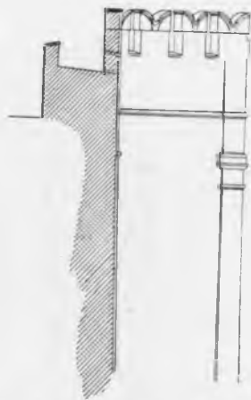
Рис. 89. Разрѣзъ и изломъ стѣны между Оружейной и Боровицкой башнями.
