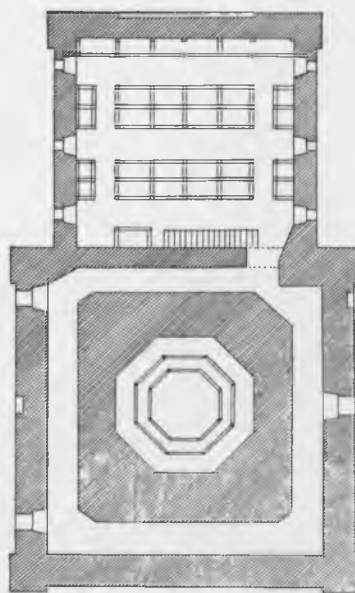
Рис. 191. 3-й этажъ.
