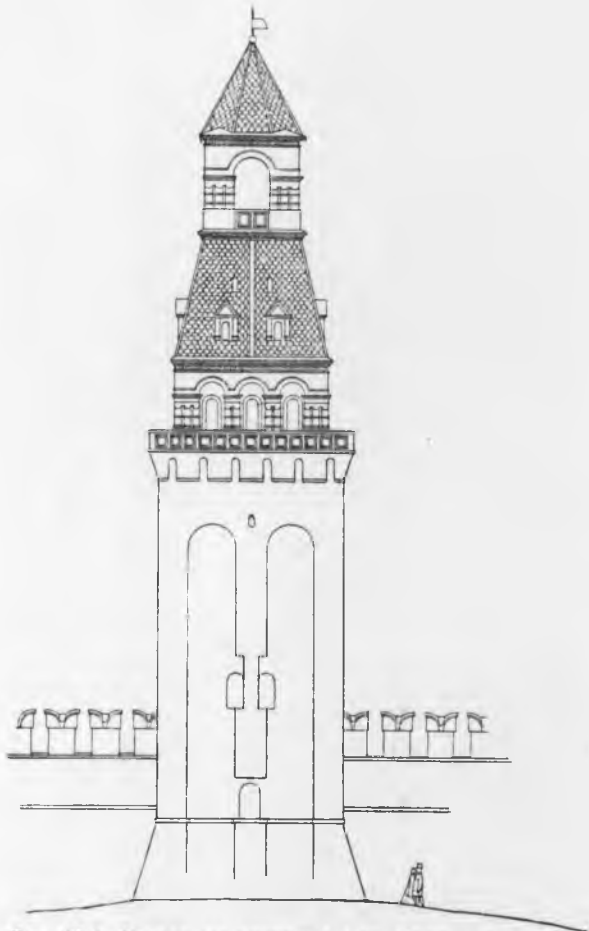
Рис. 294. Фасад со стороны 1-го Кремлевского сада.
