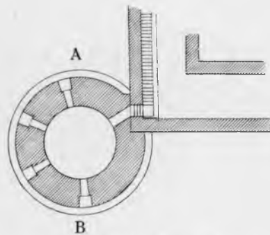
Рис. 241. 1-й этажъ.
