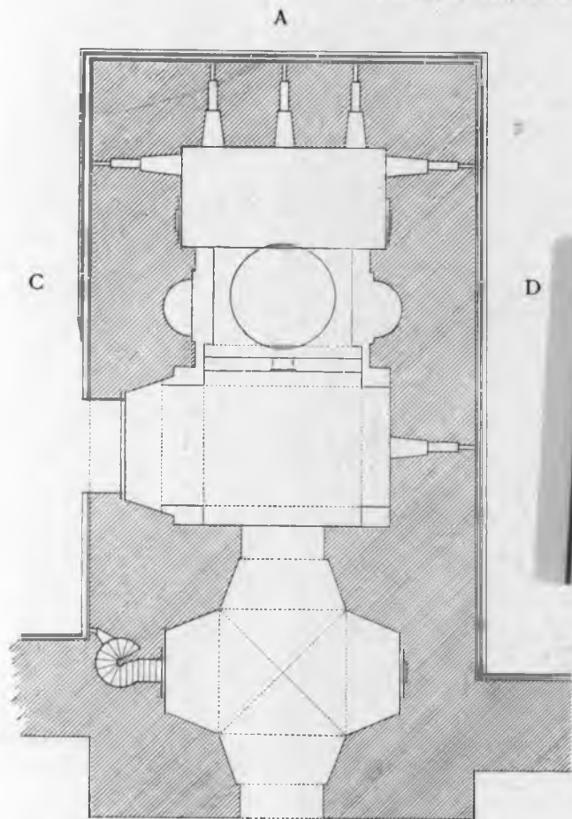
Рис. 230. 1-й этажъ.
