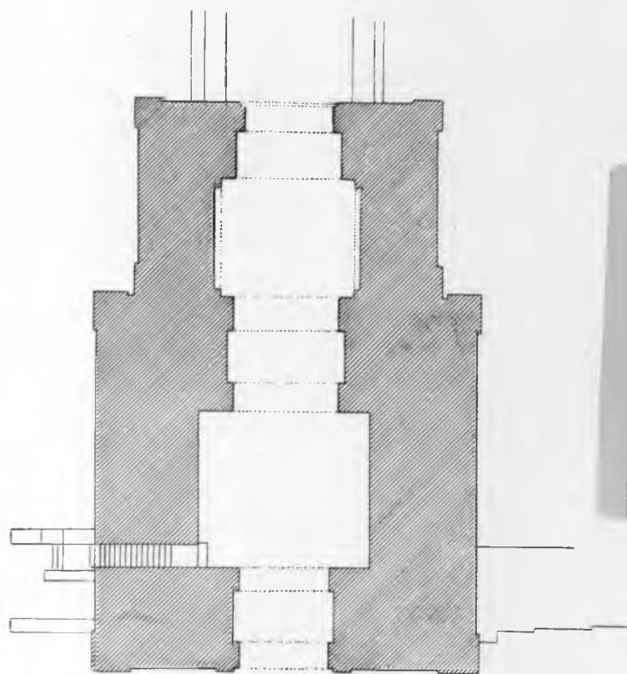
Рис. 173. 1-й этаж.
