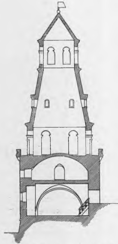
Рис. 325. Разрѣзь по линіи А В.
