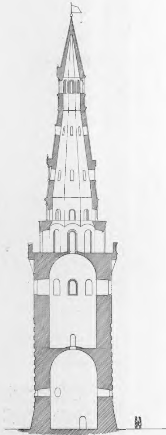
Рис. 252. Разрѣзь по линіи А В.
