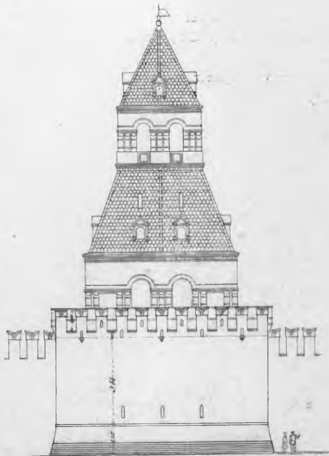
Рис. 226. Фасад Тайницкой башни со стороны Москвы рѣки.
