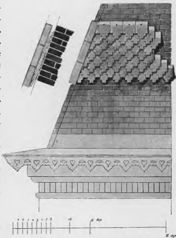
Рис. III. Черепица и подзоры на верхахъ кремлевскихъ башенъ.
