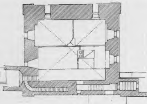
Рис. 274. 3-й этаж.
