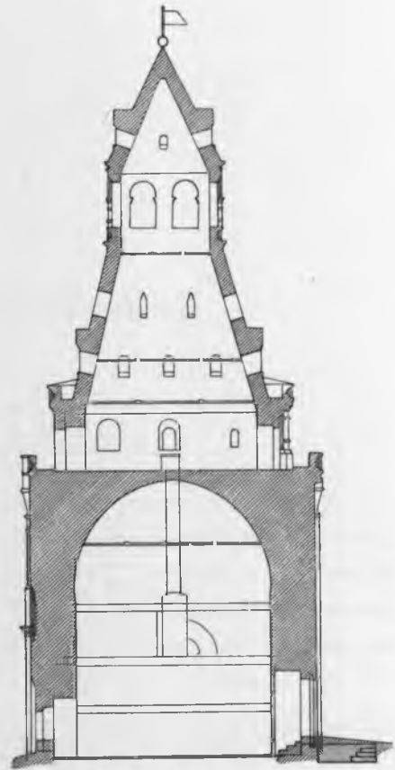
Рис. 271. Разрѣзь по линіи А. В.
