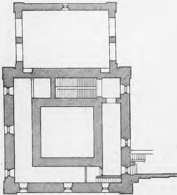
Рис. 175. 3-й этаж.
