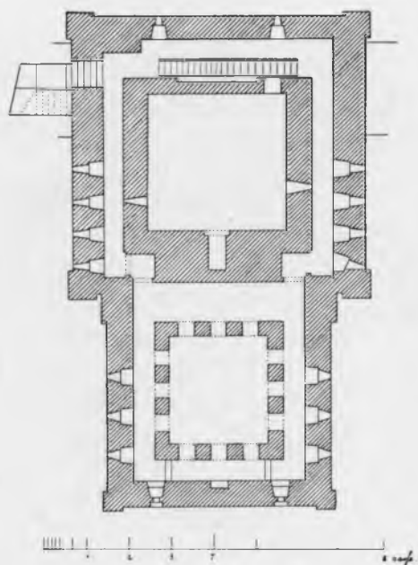
Рис. 122. 2-й этаж.
