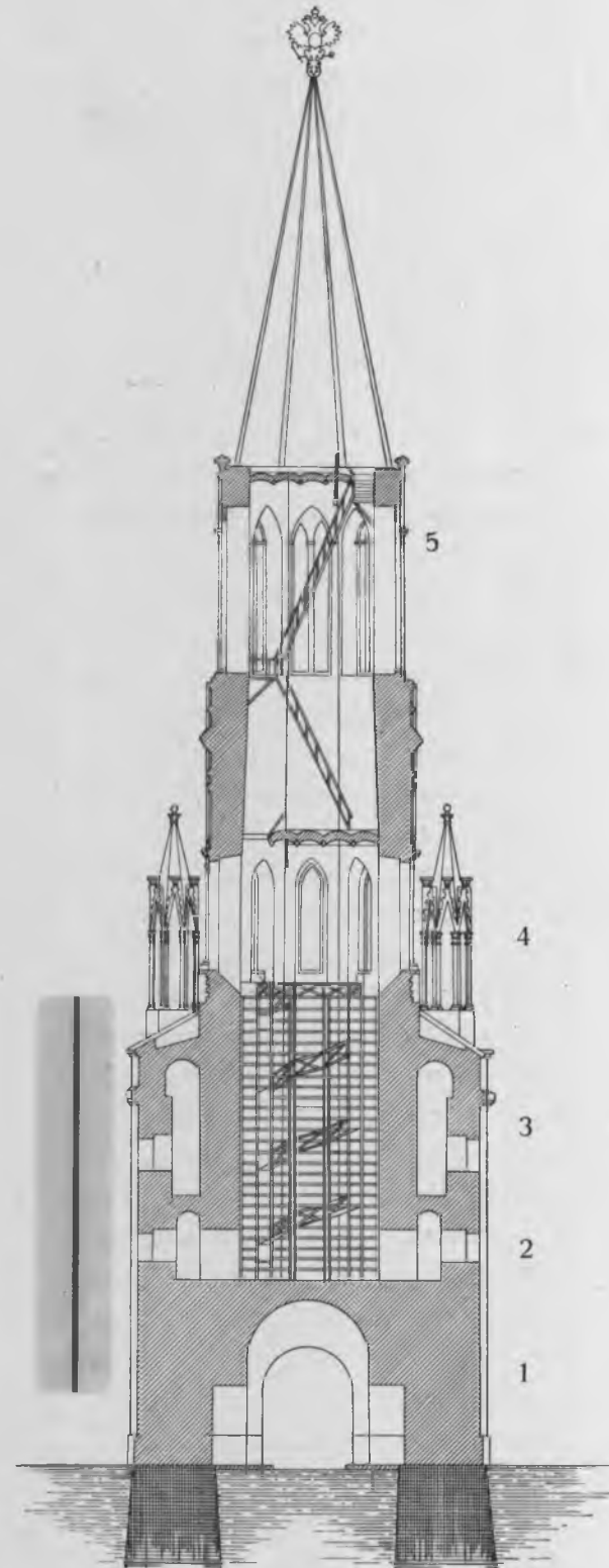
Рис. 187. Разрѣзь по линіи А В.
