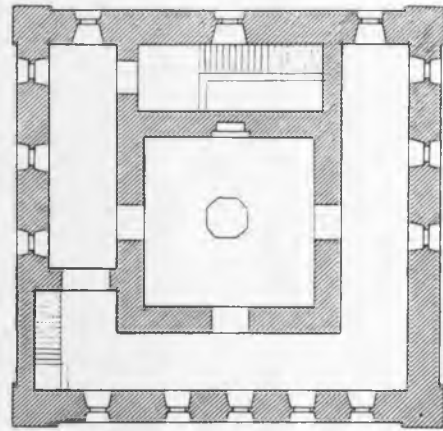
Рис. 176. 4-й этаж.
