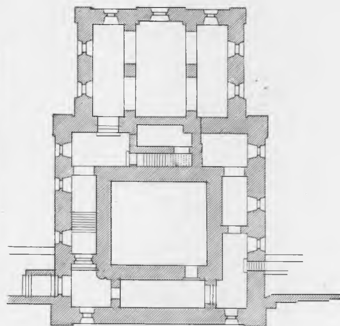
Рис. 174. 2-й этаж.
