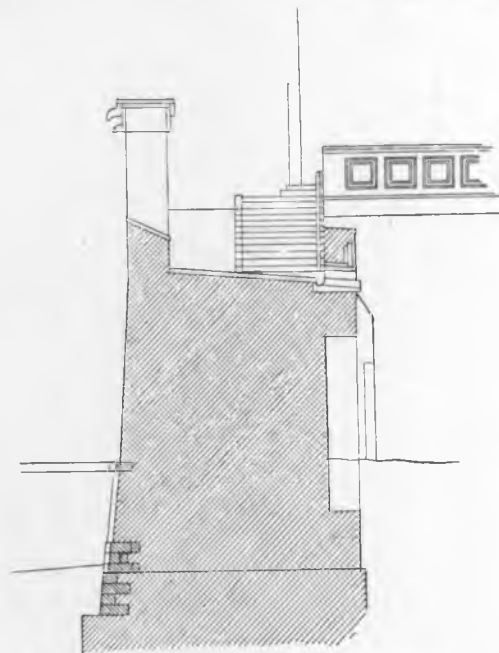
Рис. 86. Разрѣзъ стѣны между Благовѣщенской и Водовзводной башнями. [Масштабъ увелич. вдвое].
