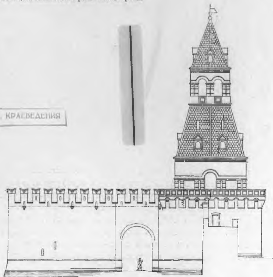
Рис. 227. Боковой, восточный фасад Тайницкой башни.
