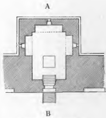
Рис. 348. 1-й этажъ.
