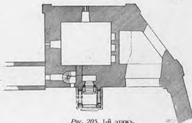
Рис. 205. 1-й этаж.
