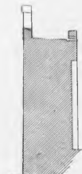
Рис. 96. Разрѣзъ стѣны между Никольской и Спасской башнями.
