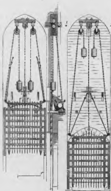
Рис. 38. Герсы въ Porte Narbonnaise въ г. Carcassonne.
