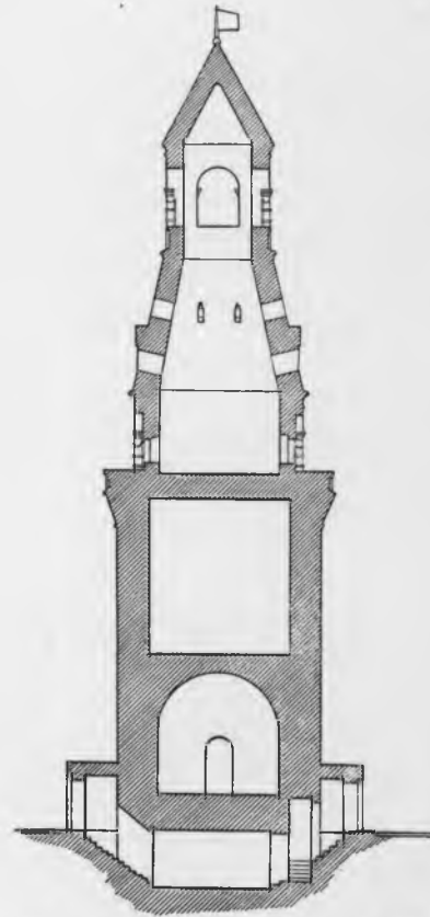
Рис. 295. Разрѣзъ по линіи А В.
