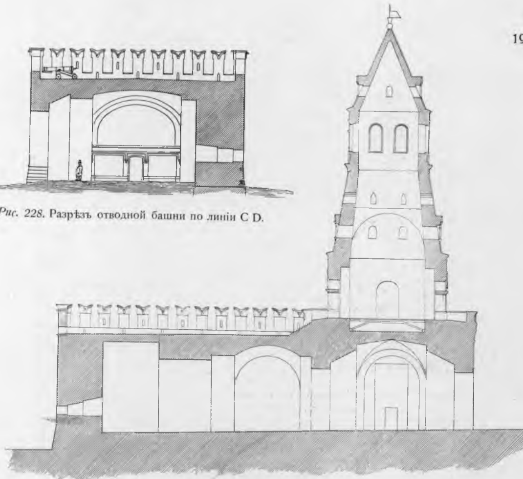
Рис. 229. Разрѣзь по линіи А. В.
