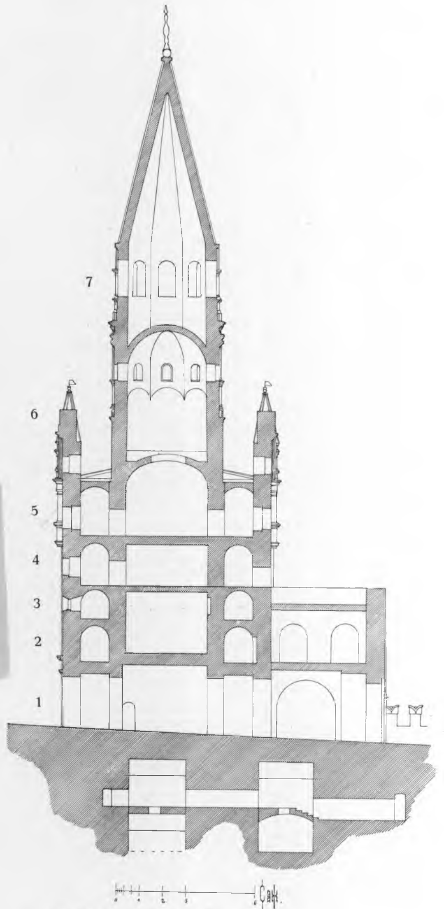
Рис. 170. Боковой разрез Троицкой башни.
