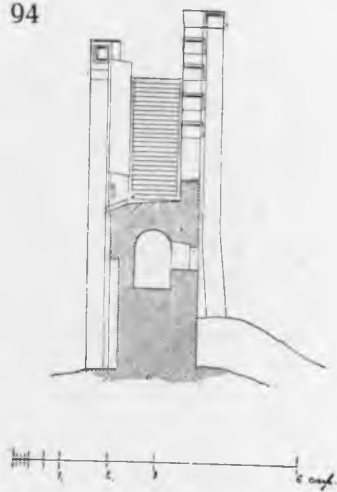
Рис. 81. Разрѣзъ стѣны между Набатной и Константиновской башнями.
