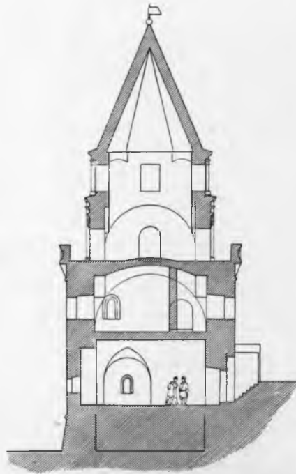
Рис. 347. Разрѣзь по линіи А В.
