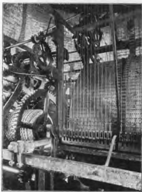
Рис. 145. Валъ для курантовъ. Часть часового механизма.
