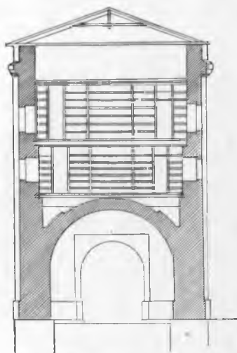
Рис. 188. Разрѣзь отводной стрельницы.
