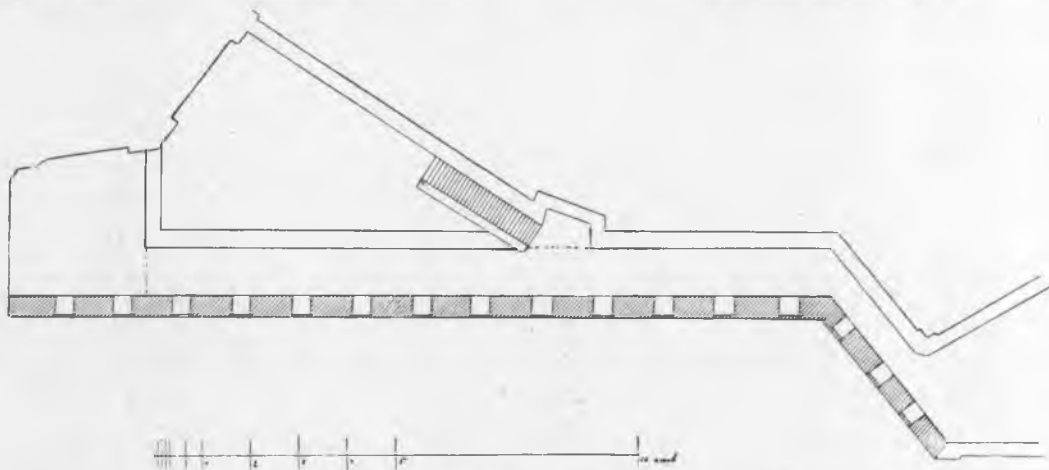
Рис. 87. Планъ стѣны между Оружейной и Боровицкой башнями. Фасадъ показаннаго на этомъ планѣ излома стѣны см. на рис. 89.
