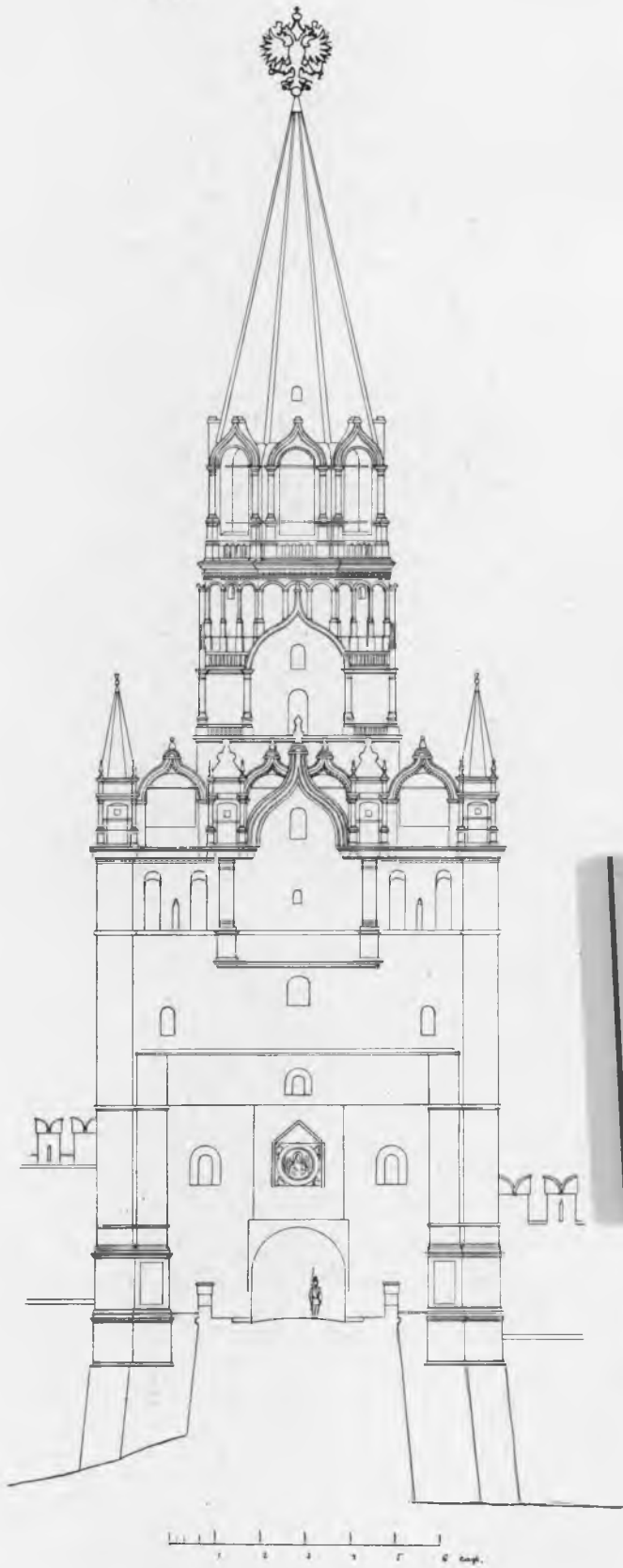
Рис. 169. Лицевой фасад Троицкой башни.
