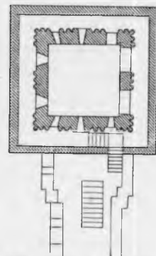
Рис. 289. 4-й этажъ.
