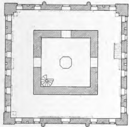
Рис. 178. 6-й этаж.
