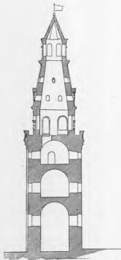
Рис. 303. Разрѣзъ по линіи А В.
