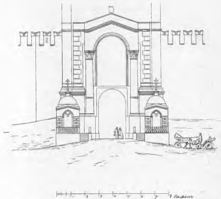
Рис. 165. Порталь Спасской башни и двѣ часовни, существовавшія до реставраціи 1866 года.
