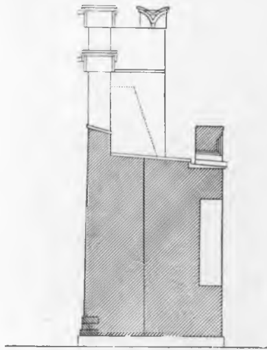
Рис. 88. Разрѣзъ стѣны между Водовзводной и Боровицкой башнями и боковой фасадъ бойницы.
