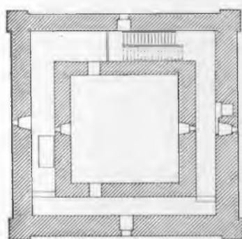
Рис. 124. 4-й этаж.
