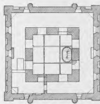
Рис. 126. 6-й этаж.
