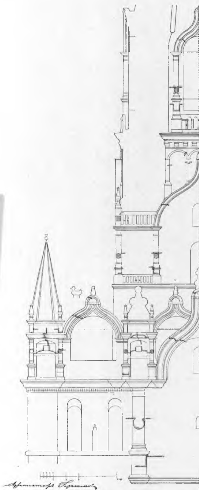
Рис. 179. Архитектурная обработка верха Троицкой башни.
