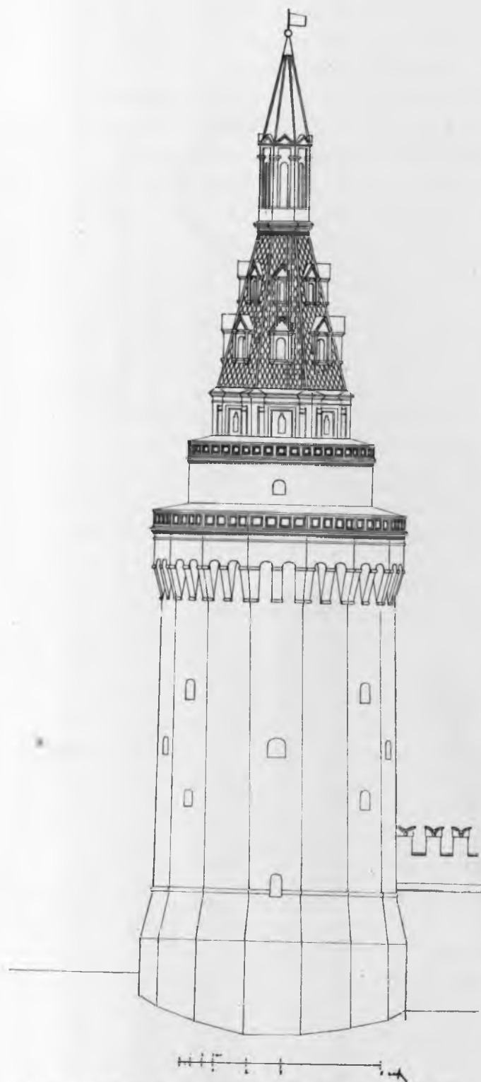
Рис. 260. Фасад со стороны 1-го Кремлевского Сада.
