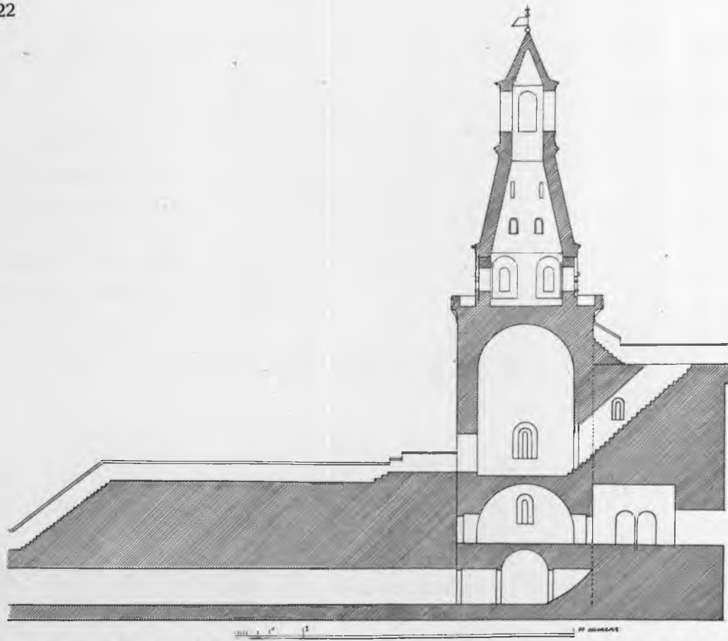
Рис. 285. Разрѣзь Набатной башни и стѣны, къ ней прилегающей по линіи А В.
