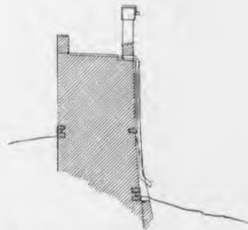
Рис. 90. Разрѣзъ стѣны между Комендантской и Оружейной башнями.
