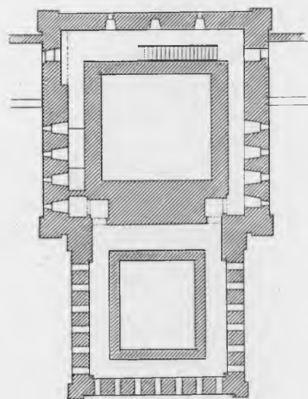
Рис. 123. 3-й этаж.
