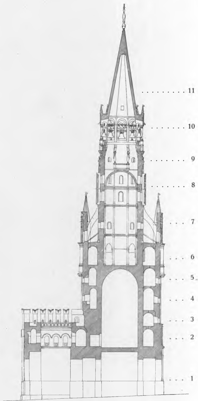
Рис. 120. Боковой разрезъ.
