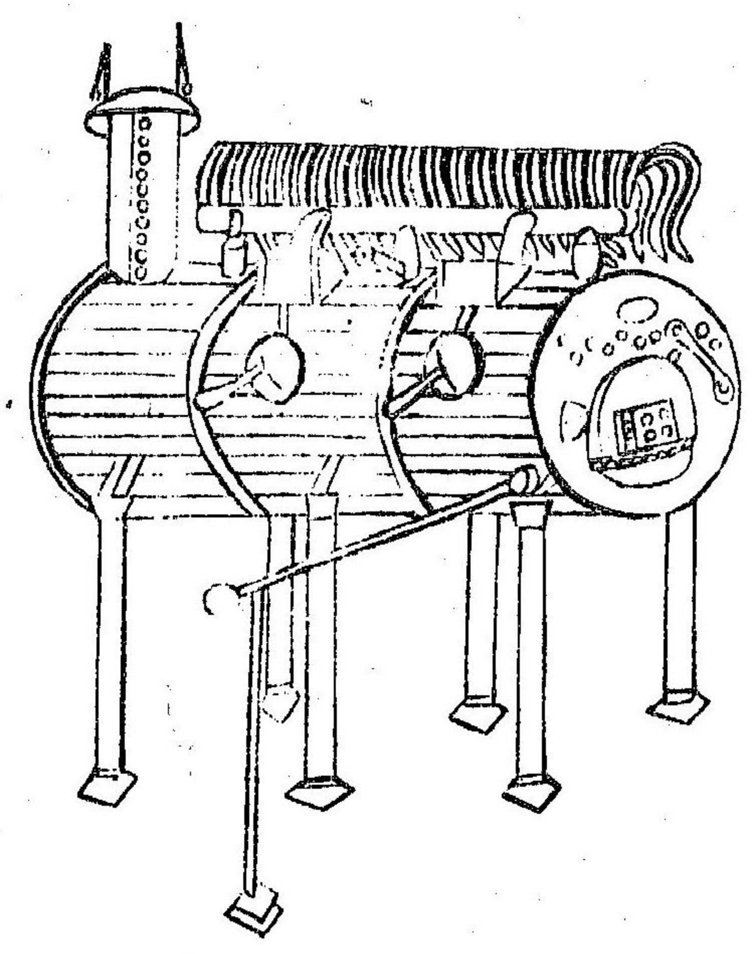
三十六 蒸汽電機
