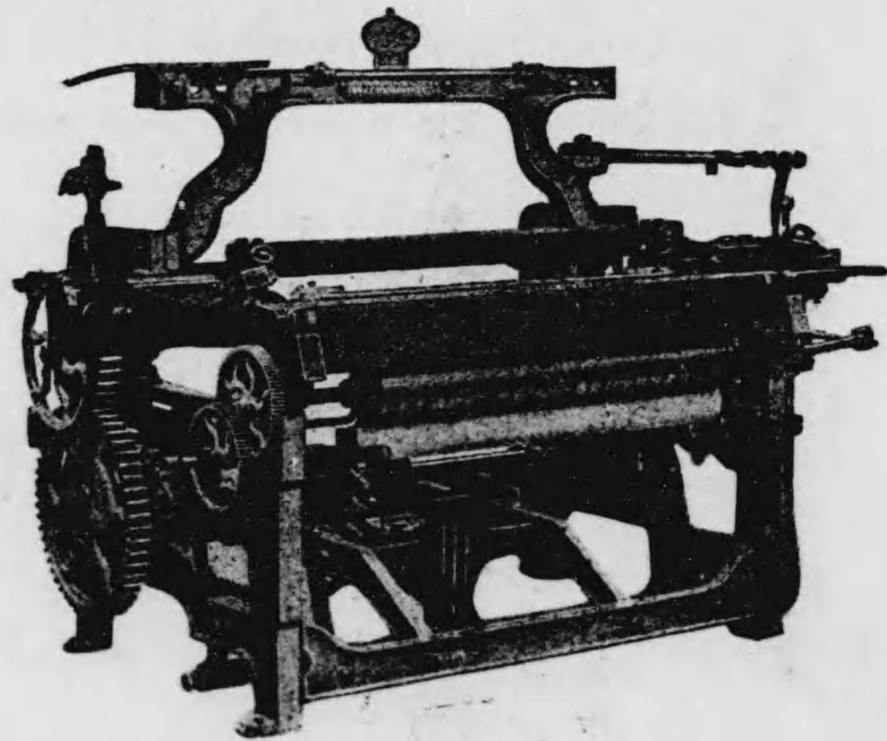
渡邊式力織機
