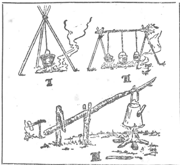
吊 灶 圖
