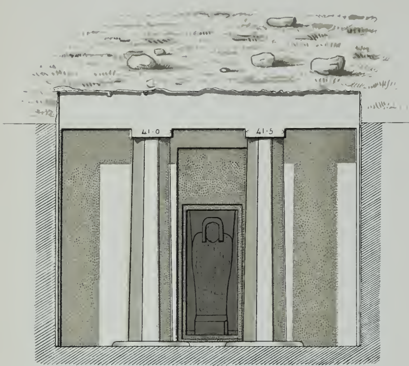
Y ELEVATION OF PORTICO.
