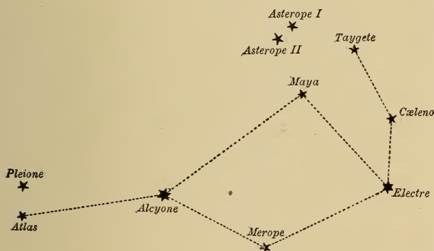
FIG. 25.—The Pleiades.
