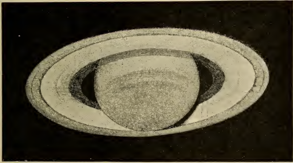
FIG. 47.—Saturn.
