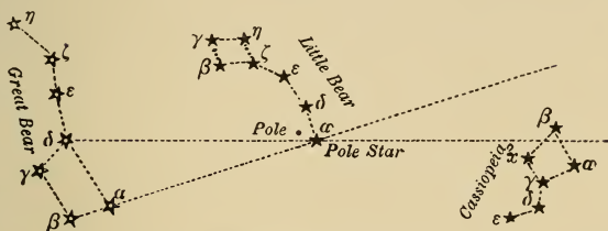
FIG. 5.—To find Cassiopeia.
