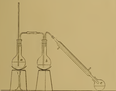
a Kolben zur Gewinnung von Wasserdampf. b Reduktionsgefäß. c Vorlage.
