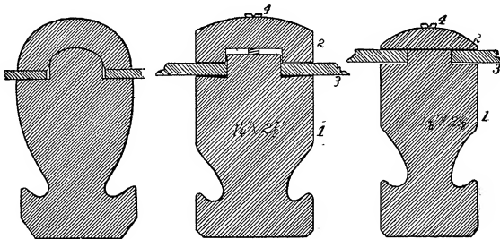
FIG. 20. FIG. 21. FIG. 22. SASH BARS FOR BUTTED GLASS.
