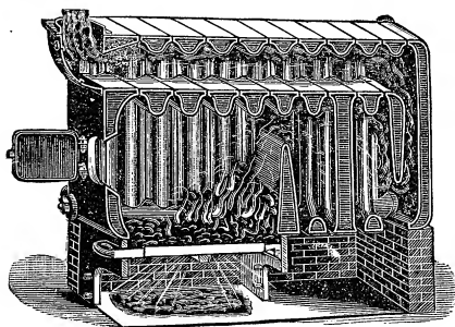
FIG. 65. CARMODY HEATER.
