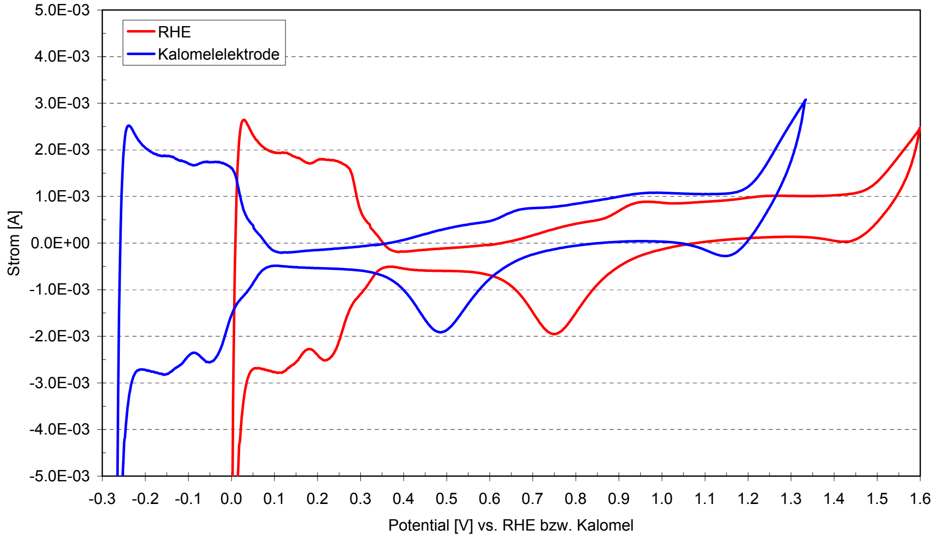
Platin in 1 N Schwefelsäure, 20°C, 100 mV/s
