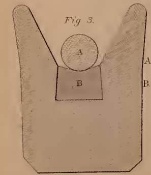
Transverse section of the pulley groove, actual size
