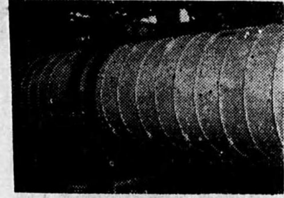
化学用ドライヤー (内径三米、長さ三〇米)
