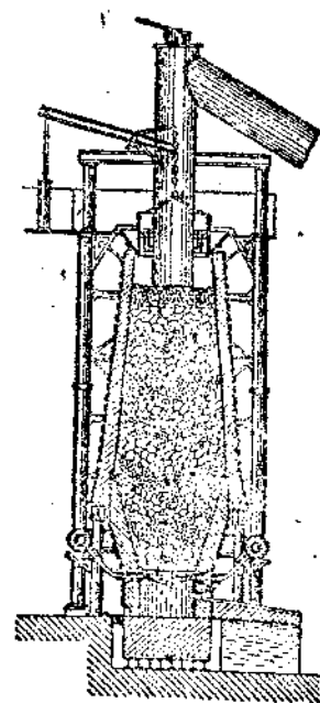
鼓風爐的內部
