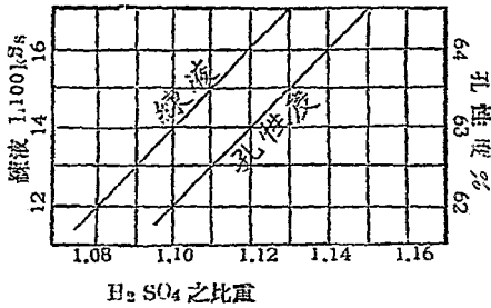
陰極板練液使用之平衡曲線
