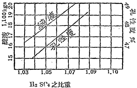
陽極板練液使用之平衡曲線
