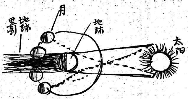
太陽 地球 月球
