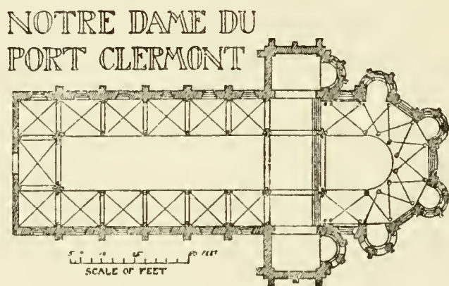
Fig. 104 (V.-le-Duc).
