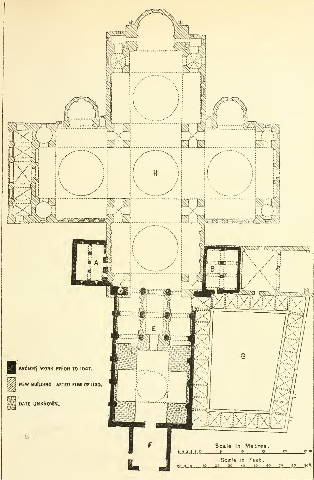
Fig. 75. PLAN OF S. FRONT, PÉRIGUEUX (Spiers)
