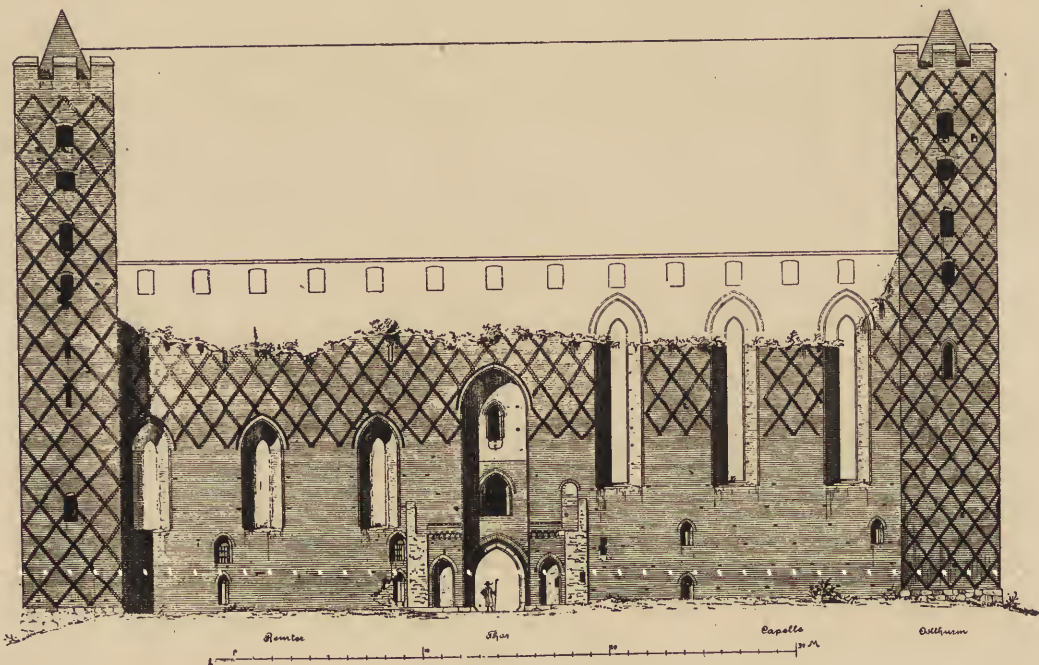
Längenschnitt
