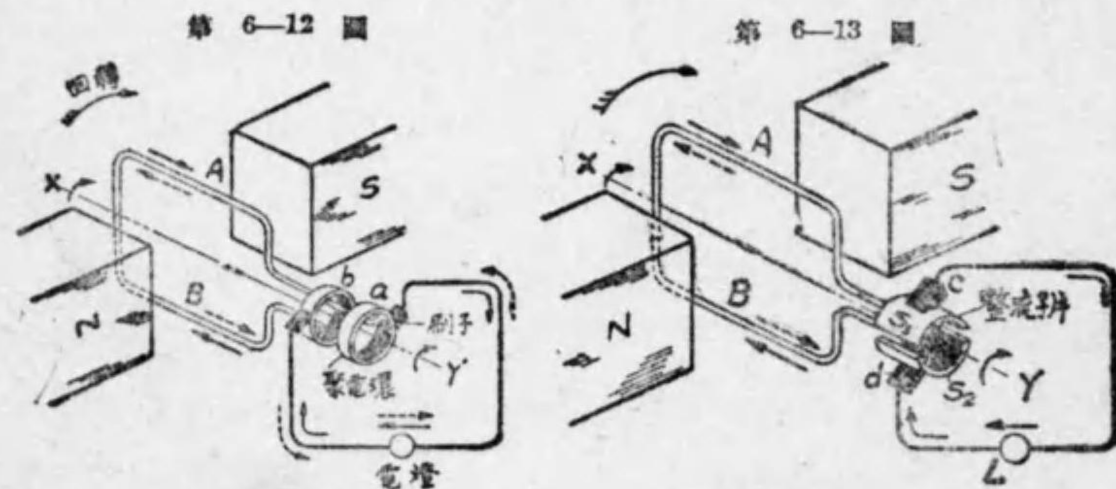
第 6—12 圖 交流發電機の原理 點線の矢印は A と B との位置が反對になつた時の電流の方向
