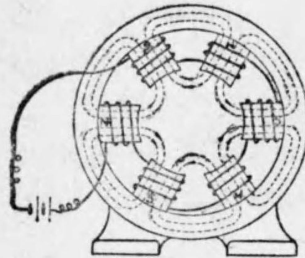
磁極が六つある發電機の界磁
