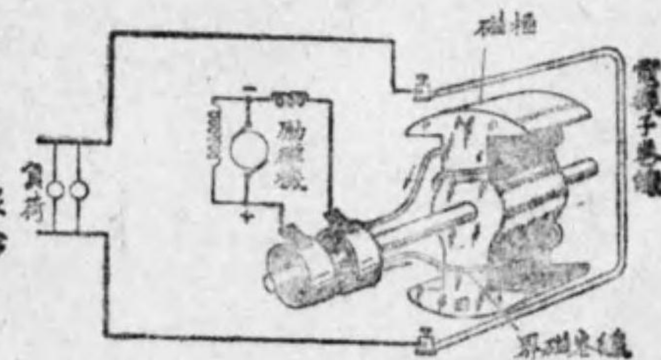
四轉界磁型交流發電機の接続圖
