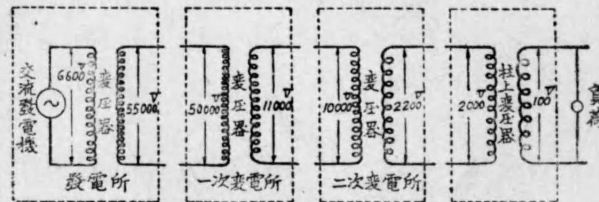
送電及び配電の有様
