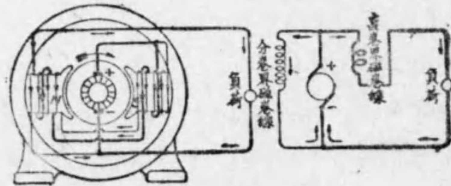
複巻発電機
