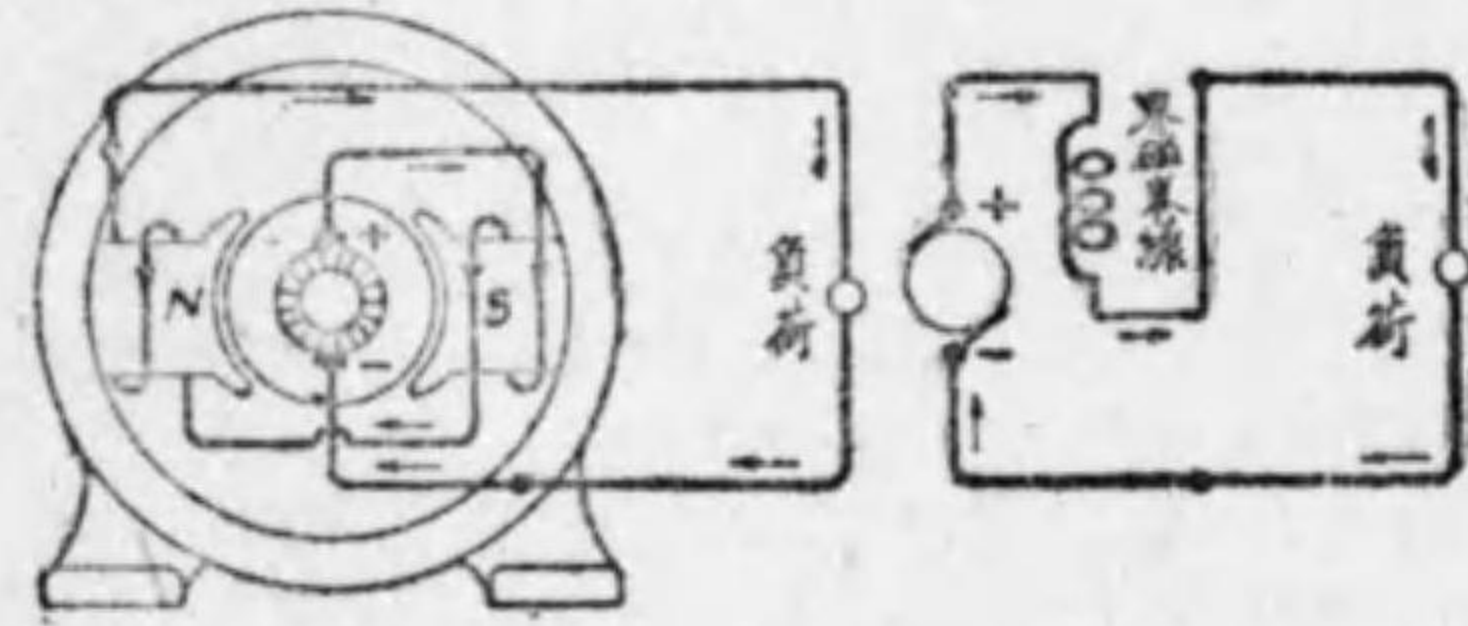
直巻発電機
