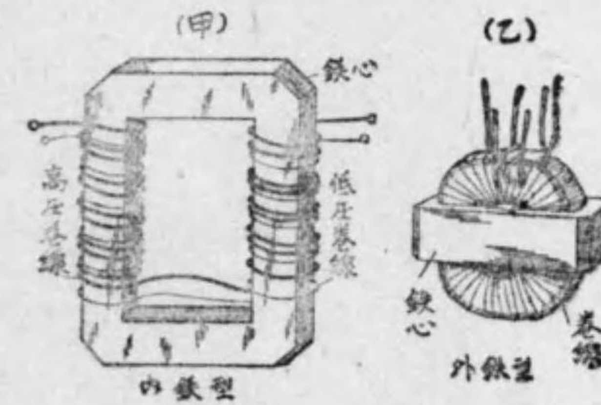
變壓器の主體
