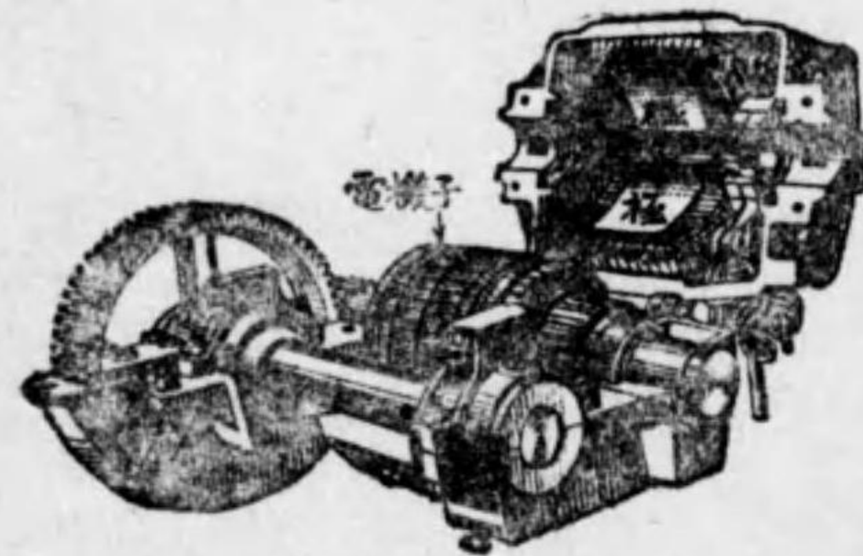
電车用直流直巻電動機の内部
