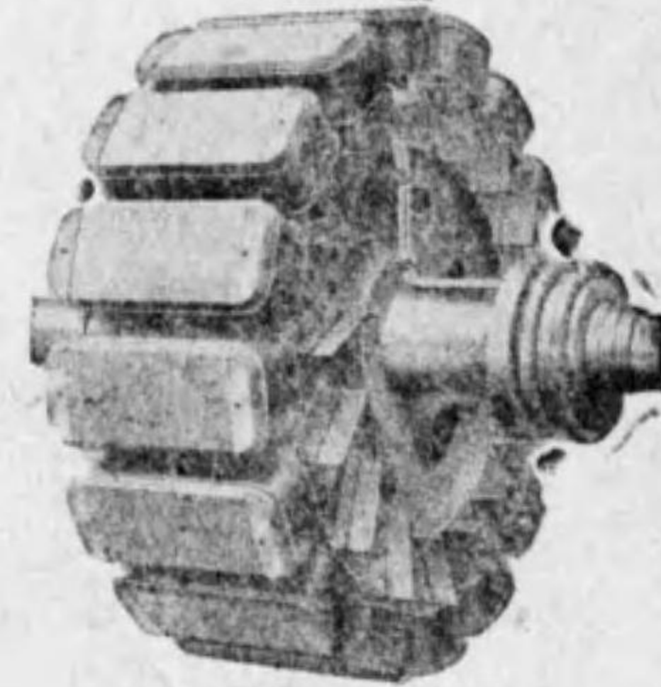
交流發電機の界磁
