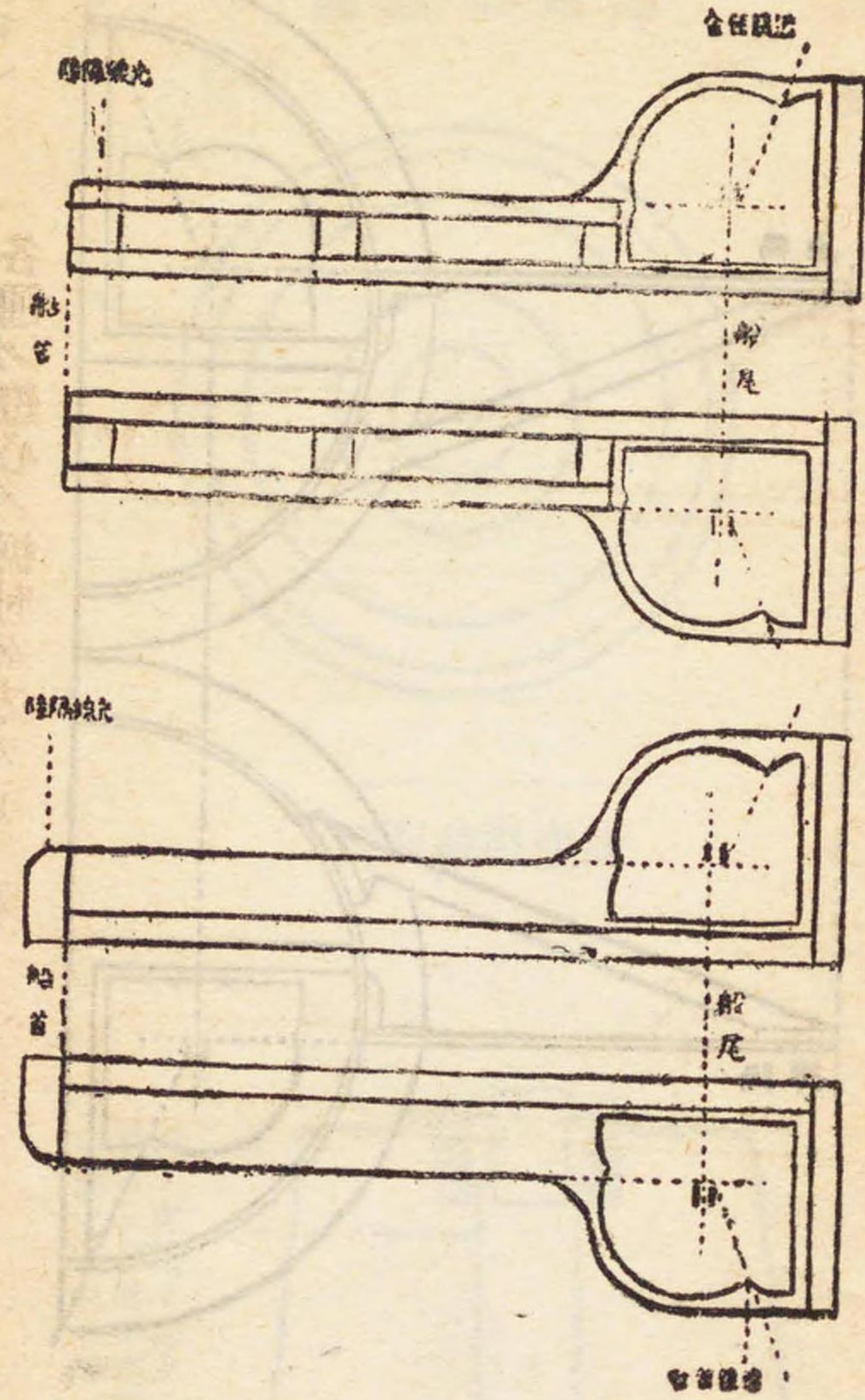
第四圖(乙) 舷燈ノ各種燈心ノ据付ケ方ヲ示ス圖
