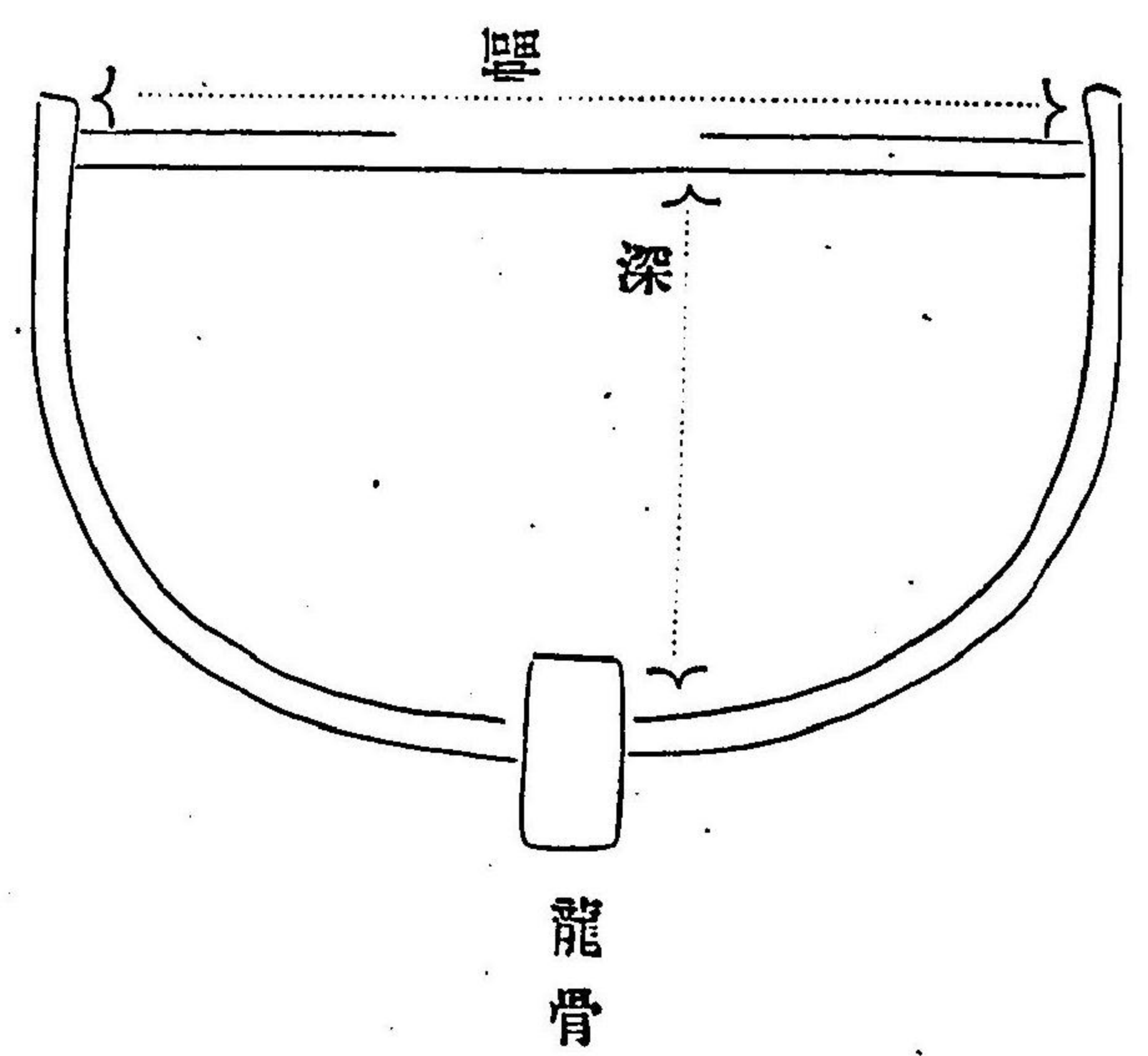
船ノ胴正面
