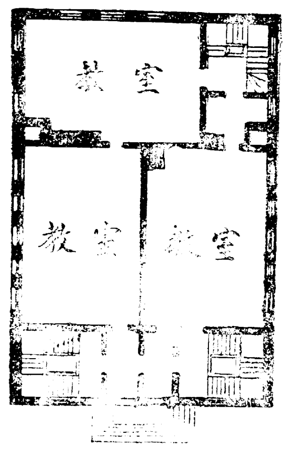
縮尺 10 5 50 英尺 阿拉白馬學校底層之平面圖
