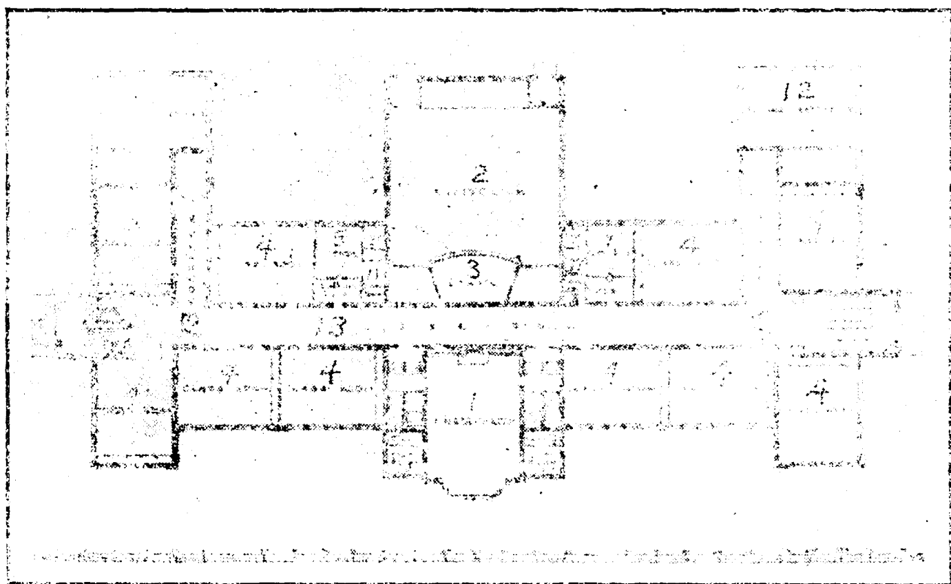
恩派埃學校之底層平面圖
