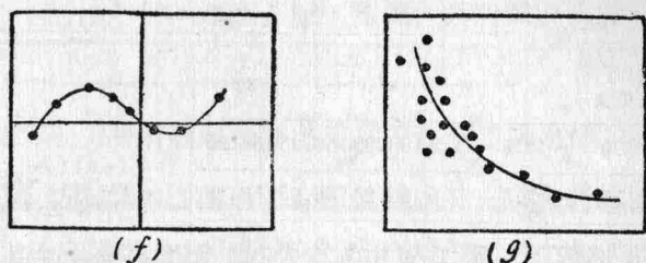
圖七十 非直線相關的表示
