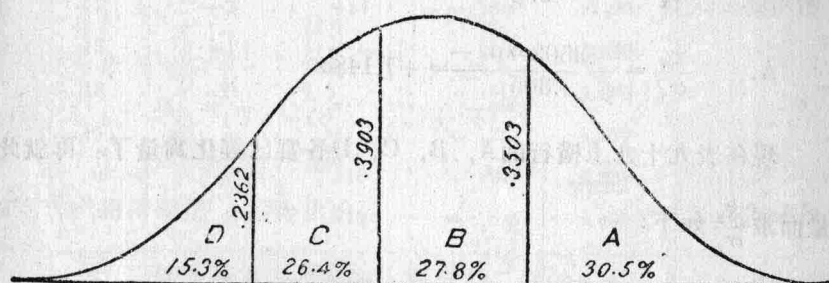
圖八十一 常態面積在相關係數計算上的應用
