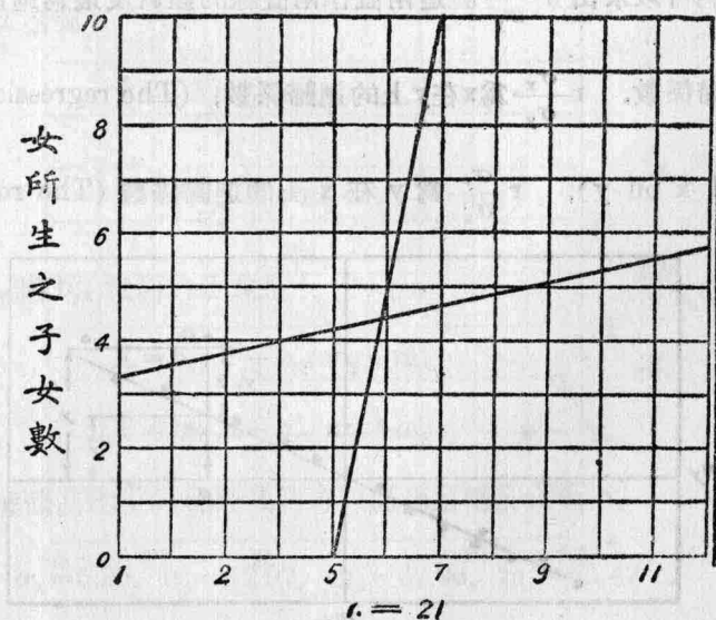
圖七十七 其三 兩線更分得開
