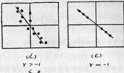
圖六十九 相關的遠近的表示
