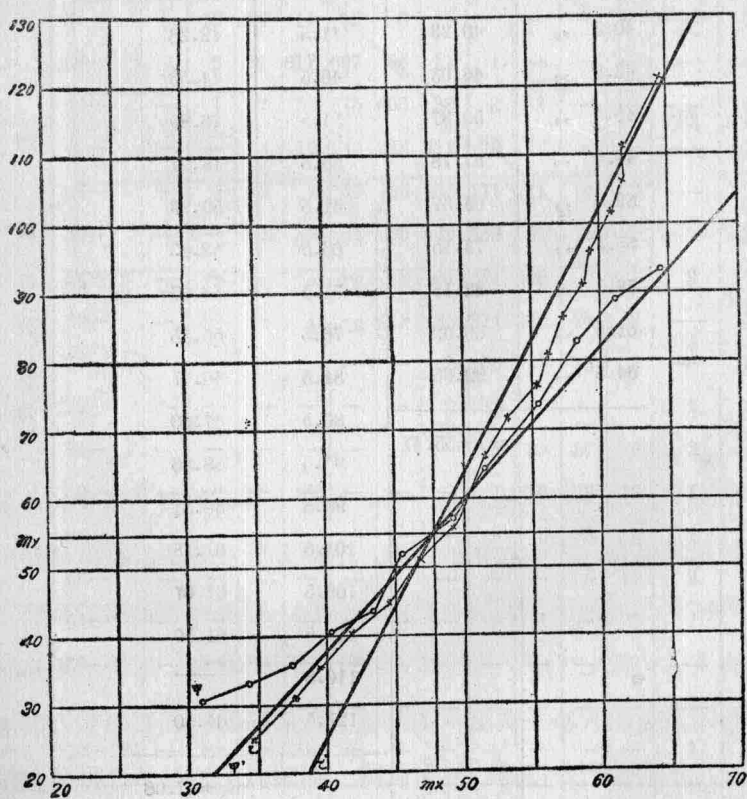
圖七十四 迴歸線之表示 (其二)
