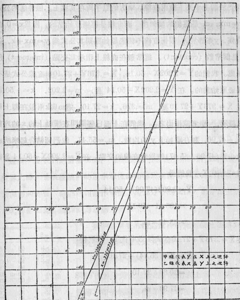
圖七十九 根據迴歸方程所繪之直線
