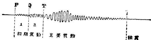
第十圖 地震波之範圍形
