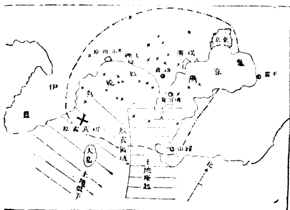
最近日本地震區圖 第五圖
