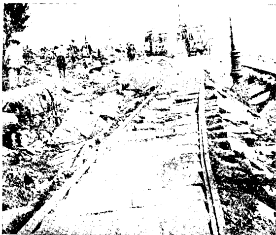
道軌車電後震地宮橫本日 圖三第
