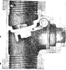
阻隔活門圖
