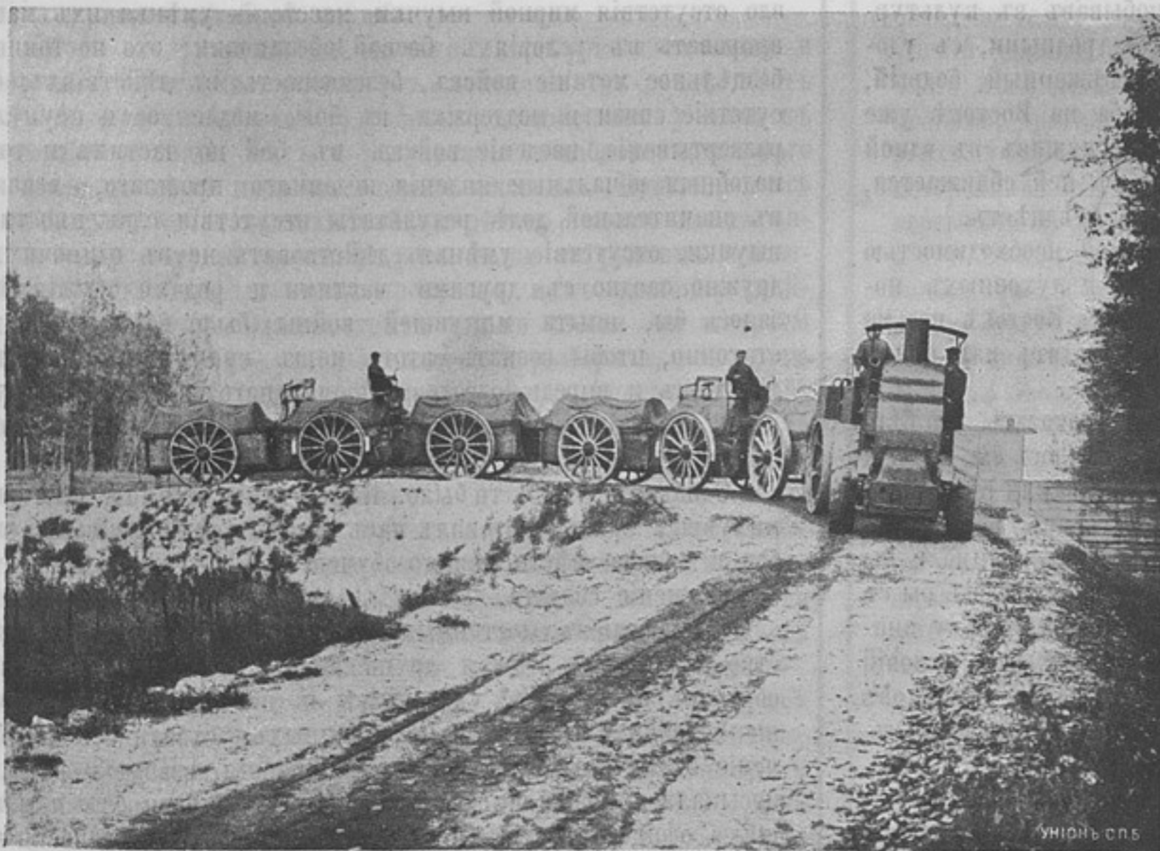
Автомобильные поѣзда въ германской арміи. Погруженный поѣздъ. Видъ спереди.
