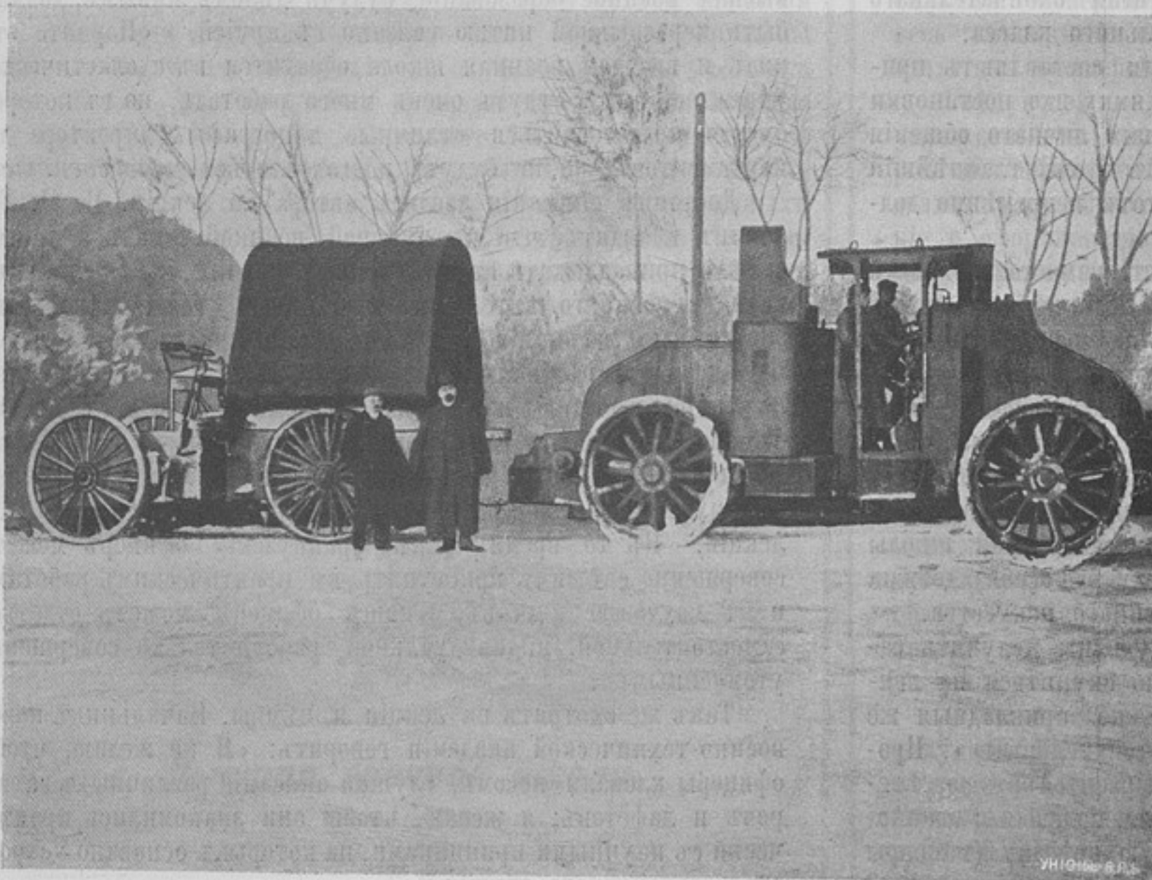
Автомобильные поѣзда въ германской арміи. При движеніи по снѣгу ободы колесъ обматываются цѣпью.
