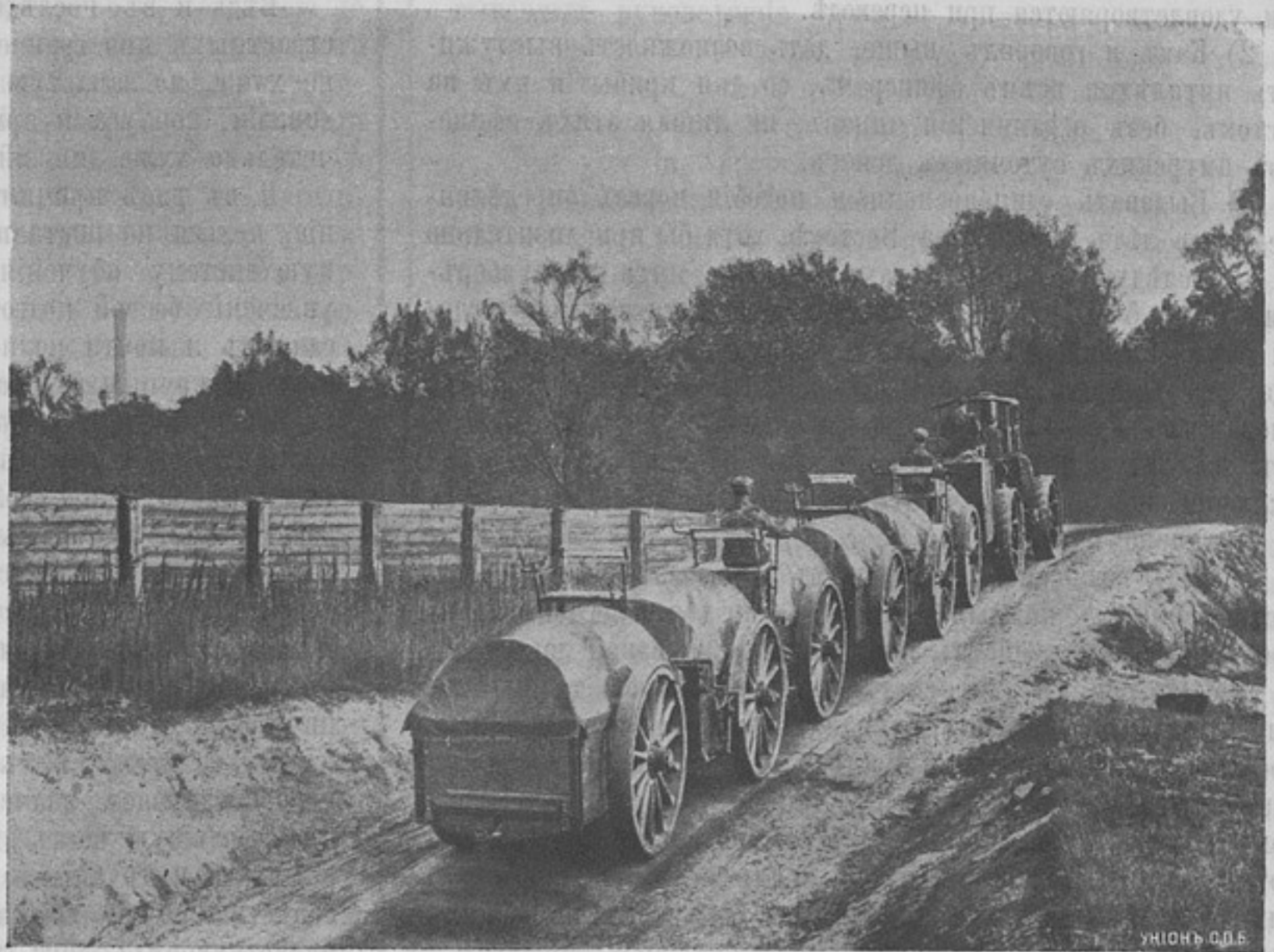
Автомобильные поѣзда въ германской арміи. Погруженный поѣздъ на сильномъ подъемѣ.
