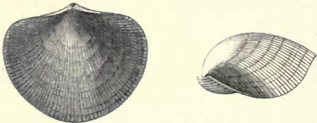
Fig. 149.— Atrypa ( Spirigera ) reticularis , Silurian.
