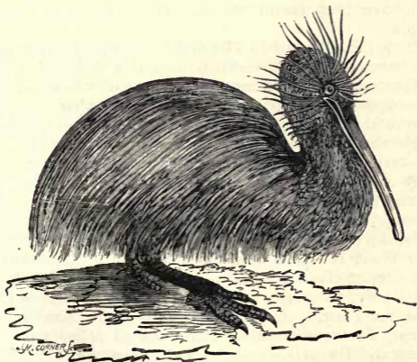
Fig. 332.— Apteryx Australis . (Gould.)
