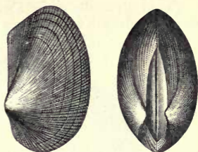
Fig. 183.— Arca antiqua . Permian.
