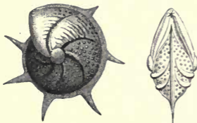
Fig. 8.— Robulina echinata , a "nautiloid" Foraminifer. D'Orbigny.
