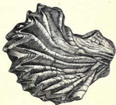
Fig. 171.— Ostrea Marshii , Oxford Clay (Middle Oolites).
