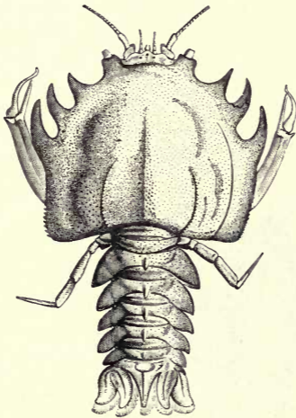
Fig. 122.— Eryon arctiformis , Middle Oolites (Solenhofen Slates).
