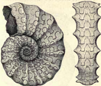
Fig. 259.— Ceratites nodosus . Muschelkalk (Middle Trias).
