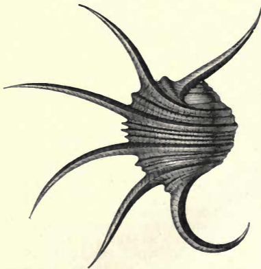
Fig. 207.— Pteroceras oceani . Neocomian.
