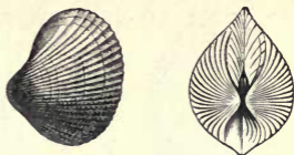
Fig. 201.— Pholadomya aequivalvis . Chalk.
