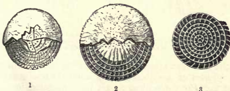
Fig. 13.— Nummulites laevigatus . Eocene.
