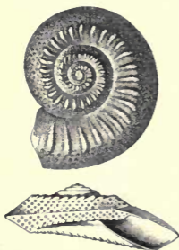
Fig. 218.— Solarium ornatum . Gault (Upper Cretaceous).
