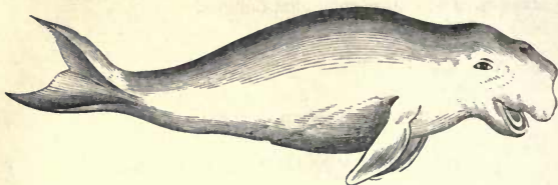
Fig. 346.— Sirenia . Dugong ( Halicore ).
