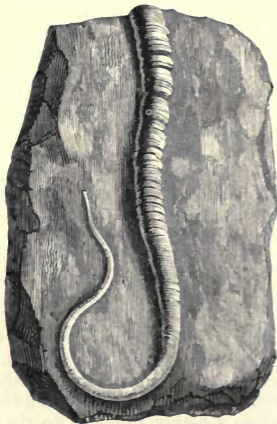
Fig. 90.— Serpula flagellum . Oxford Clay. (Jurassic.)
