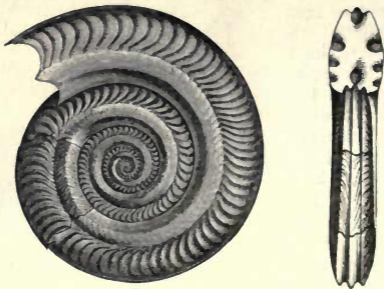
Fig. 261.— Ammonites bifrons . Lias.
