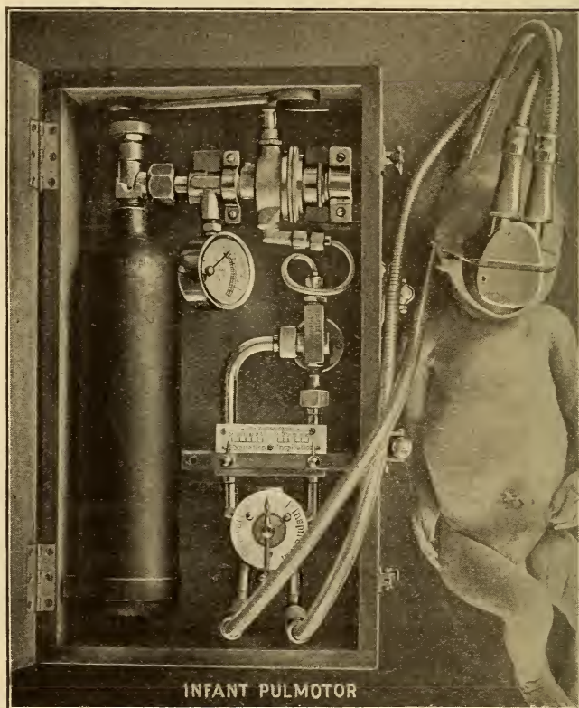
Fig. 16.—Infant Pulmotor.
