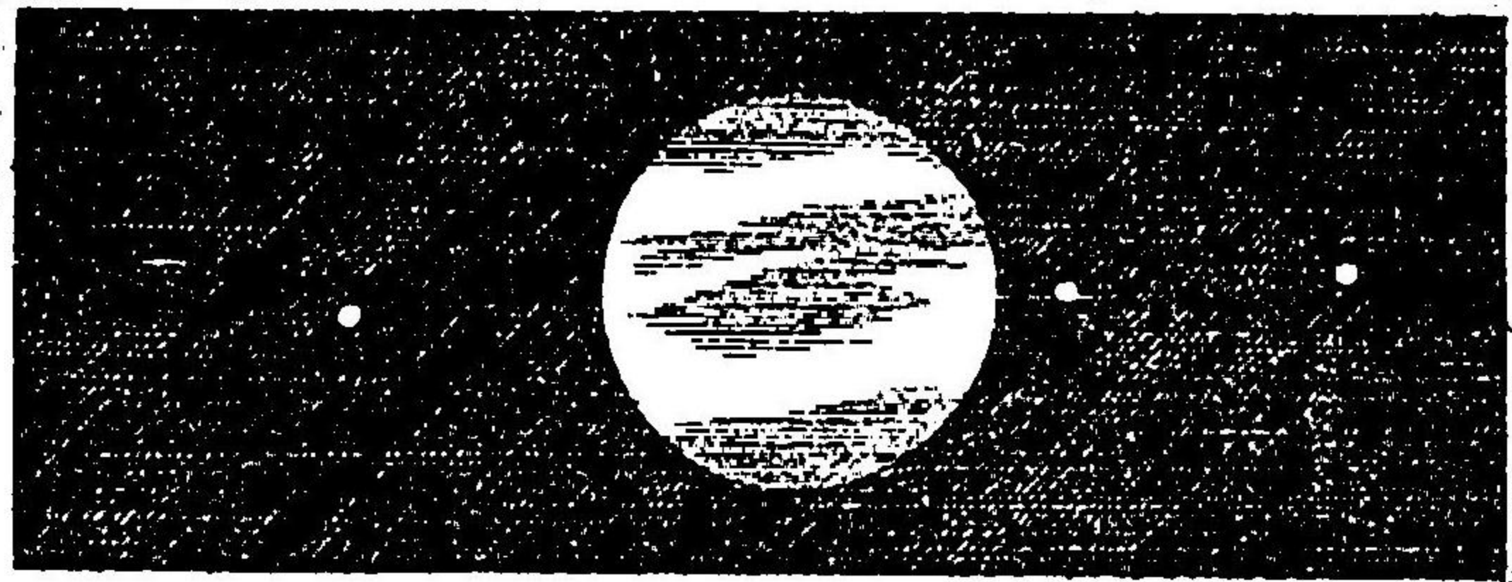
圖之星行小四及体形星木
