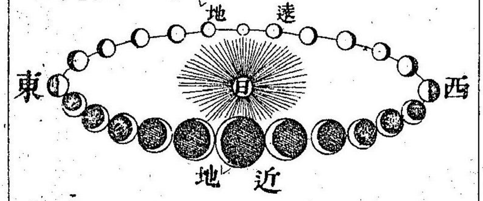
金星日行盈缺之圖
