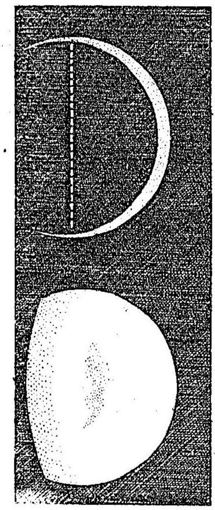
火星將盈之圖
