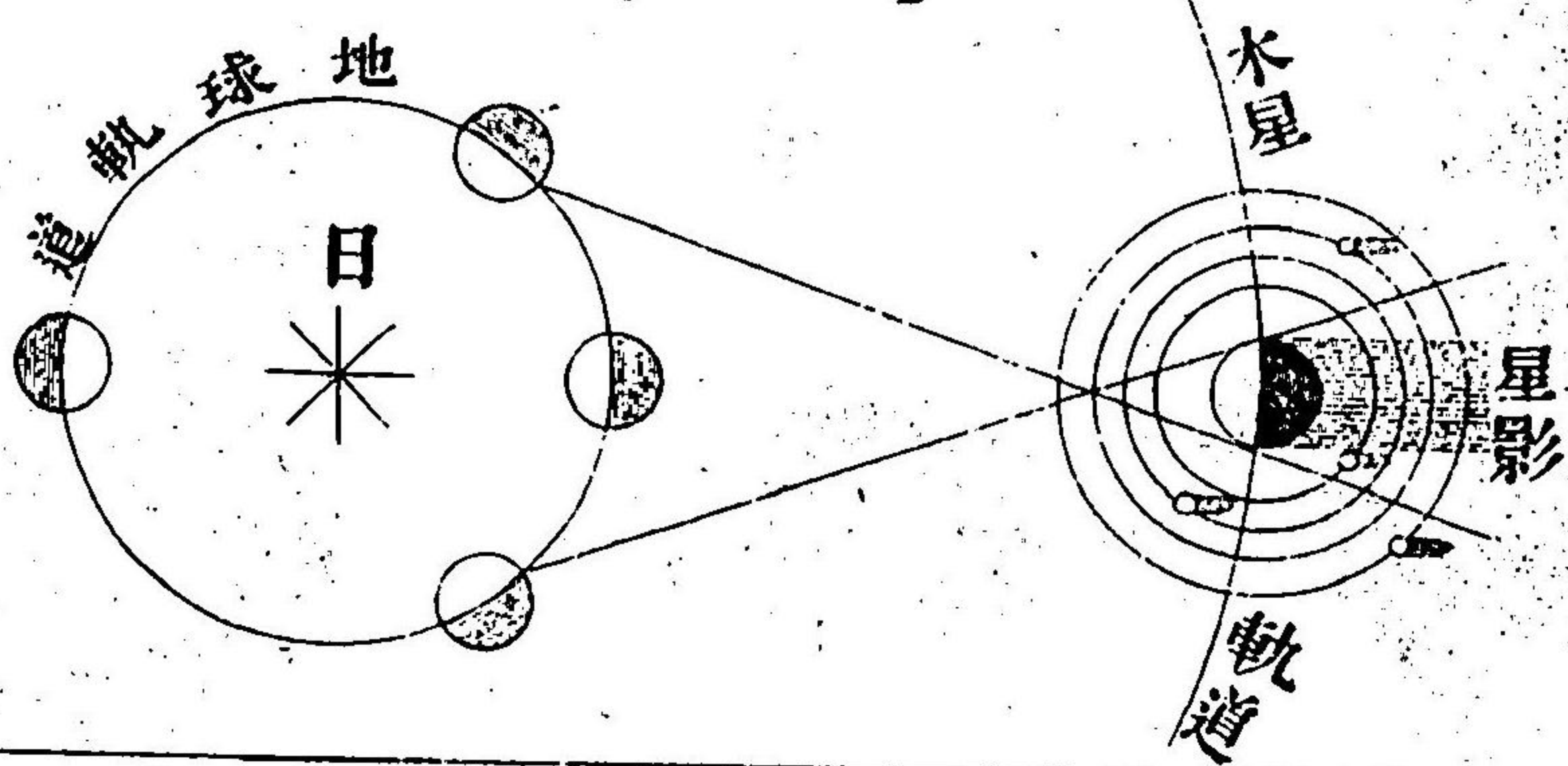
四小行星行木星之圖
