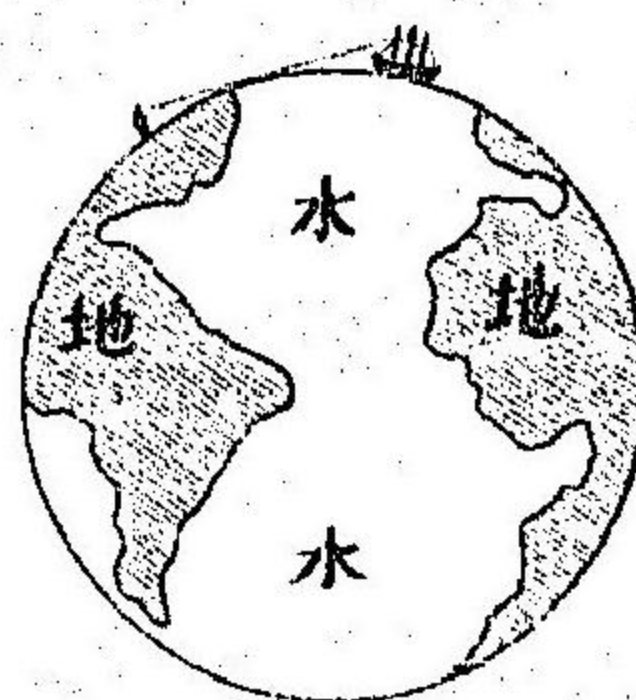
地球圓體憑據圖
