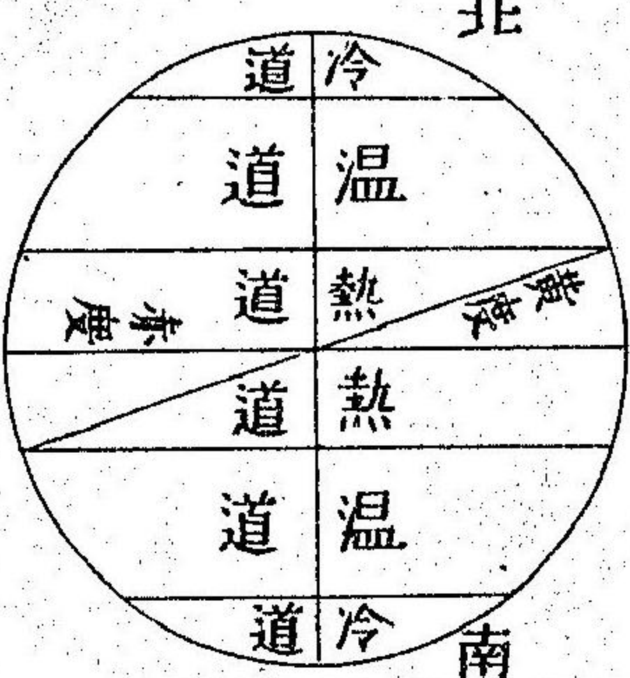
日行黃度分冷熱圖
