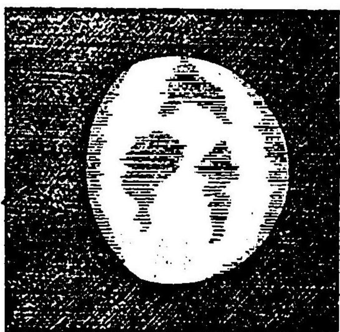
圖之盈將星火
