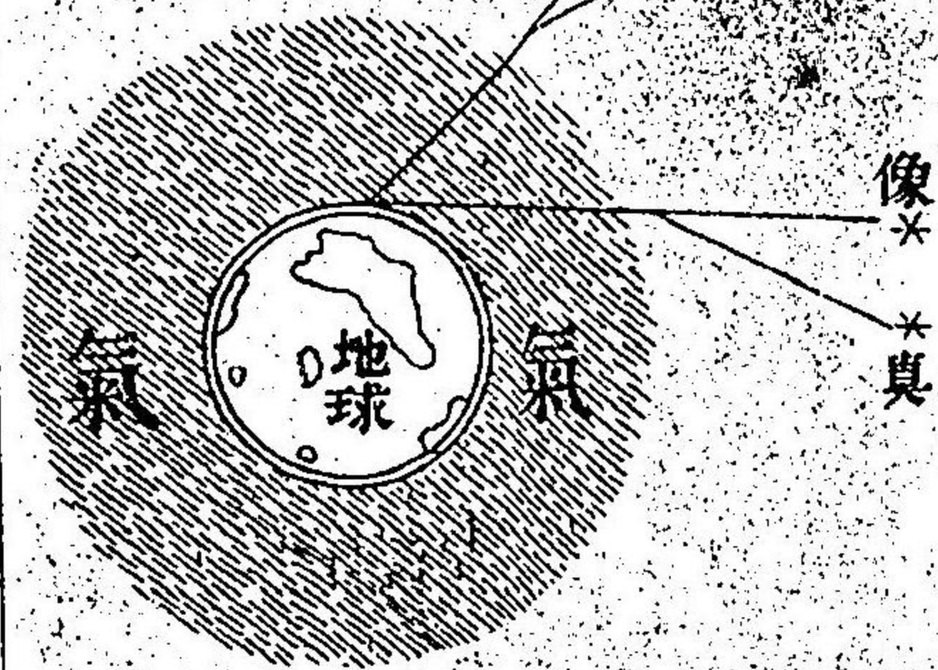
日光入氣斜射圖
