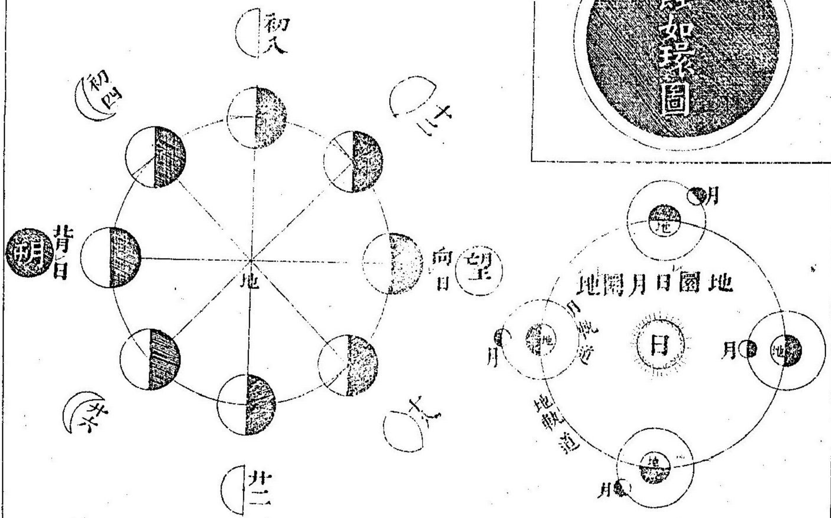
月輪地成湖望圖
