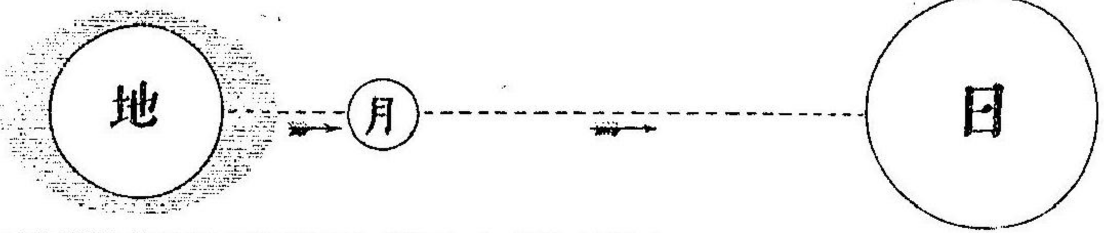
行星與日較大小圖
