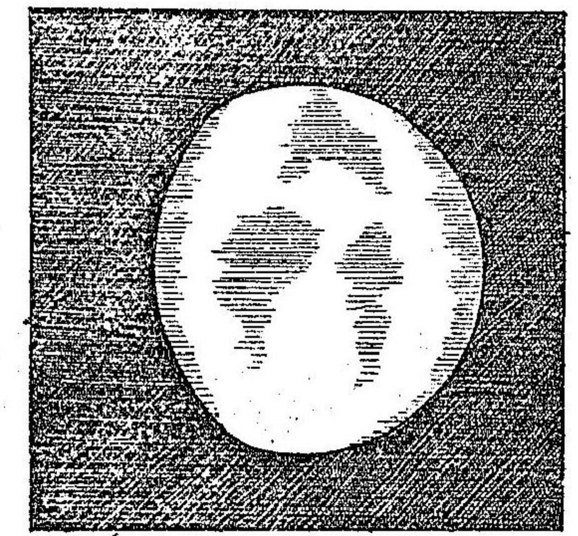
火星將盈之圖
