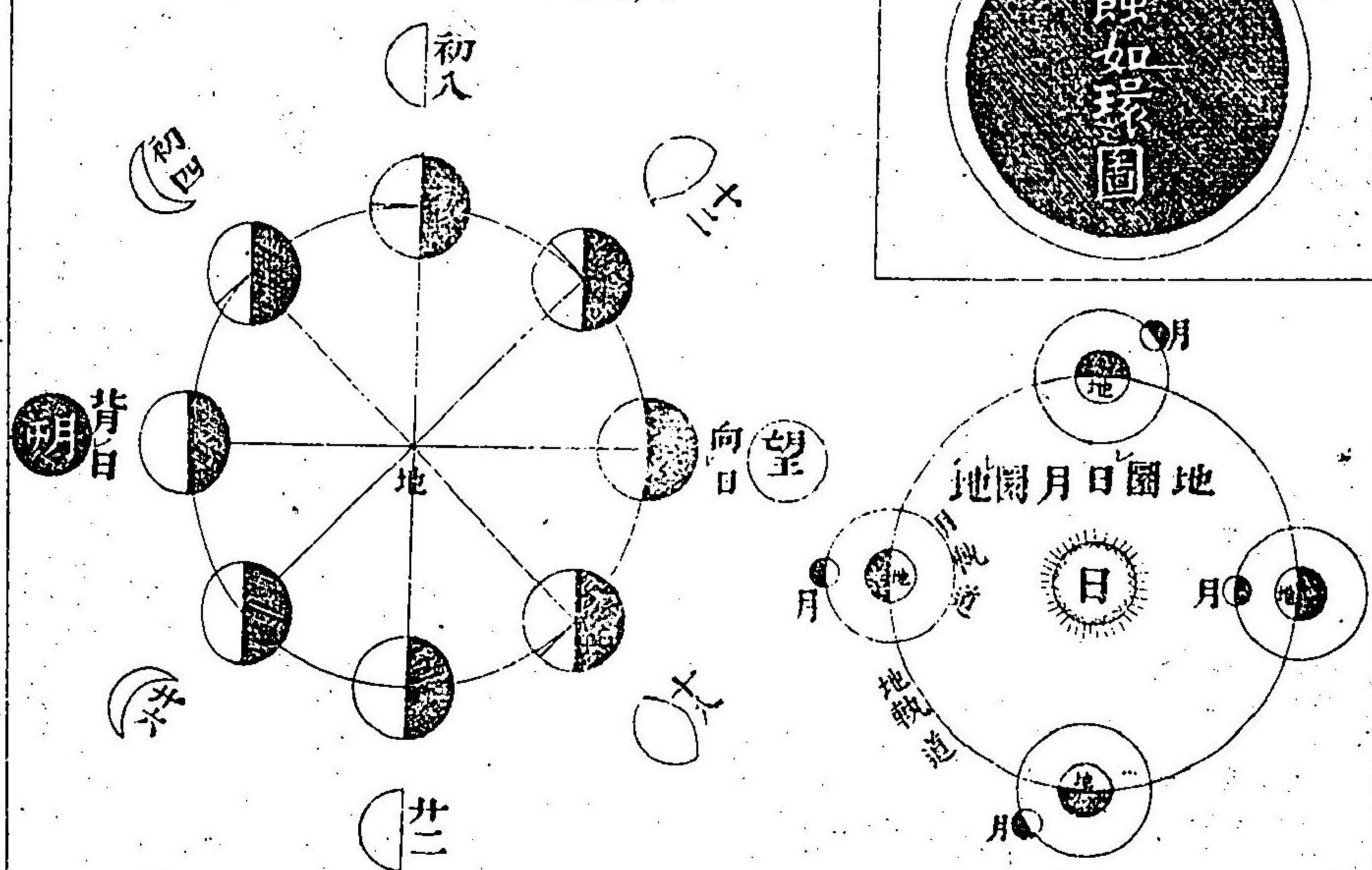
月輪地成朔望圖
