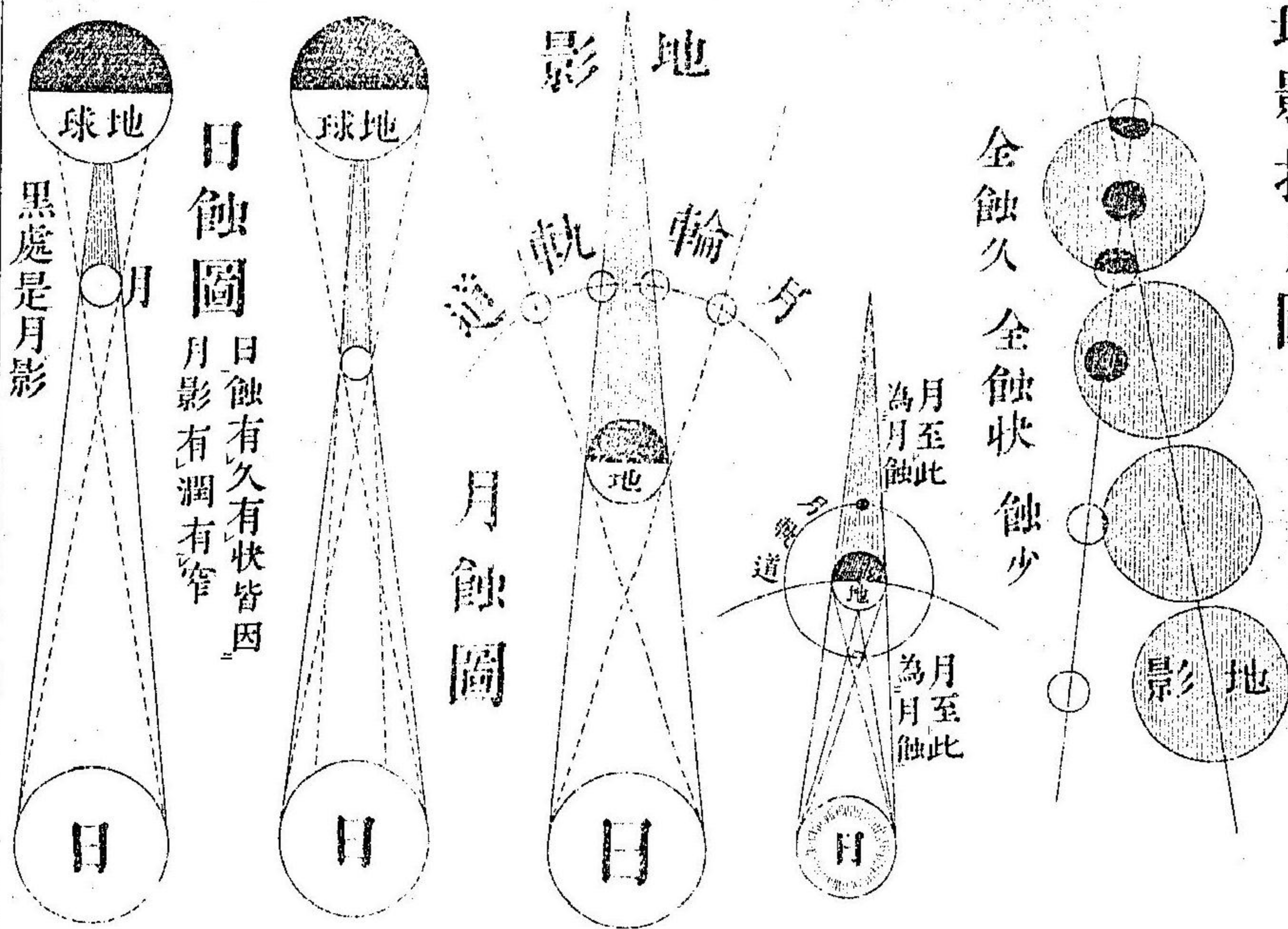
月輪地成湖望圖
