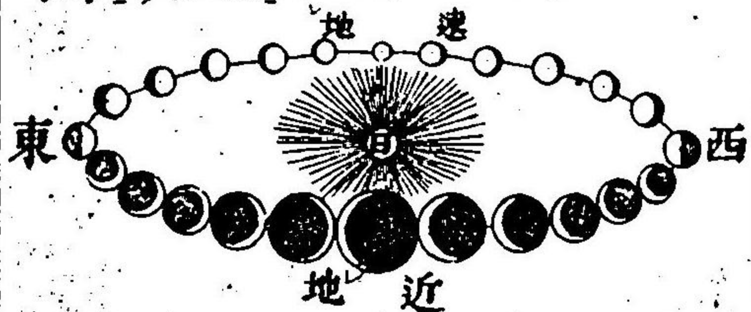
圖缺盈成行日圍星金
