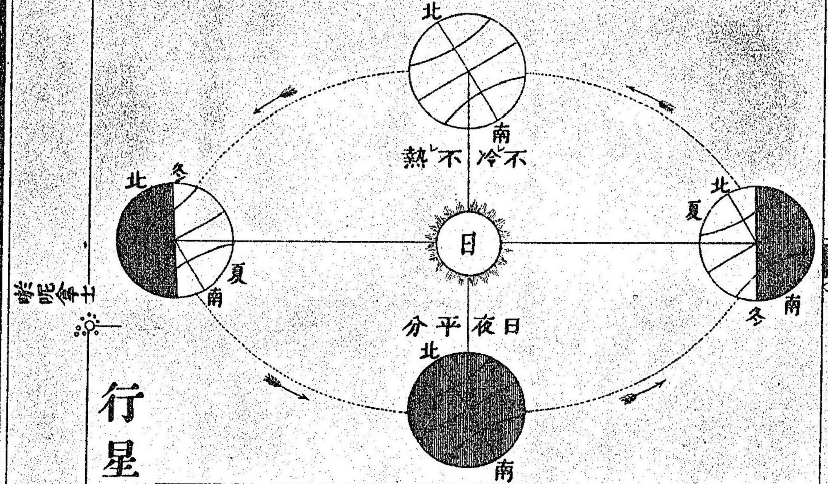
地球側倚圖成四季圖
