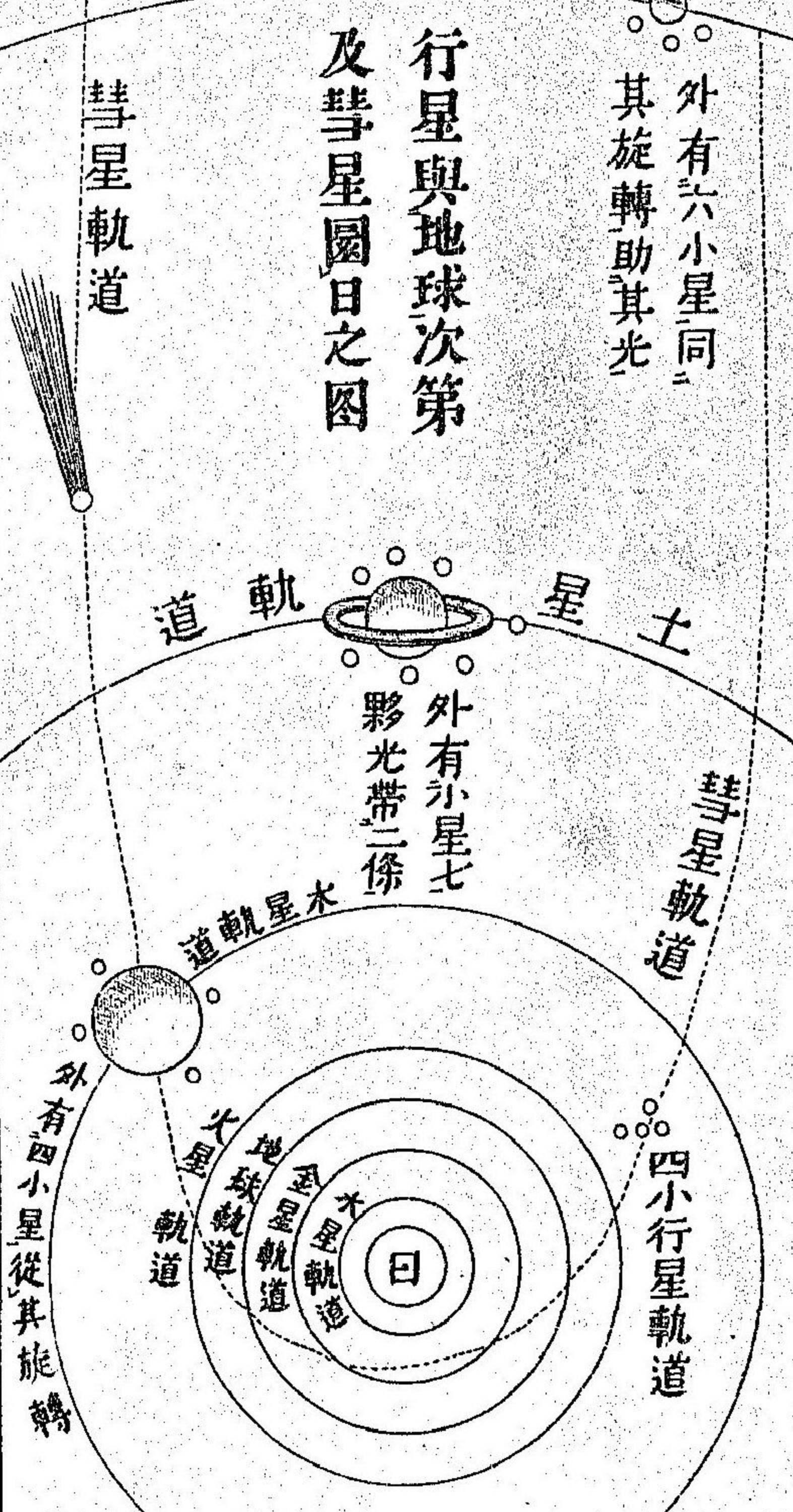
於呢拿士行星軌道
