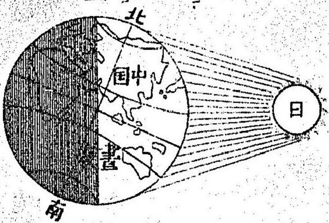
地球分日夜圖
