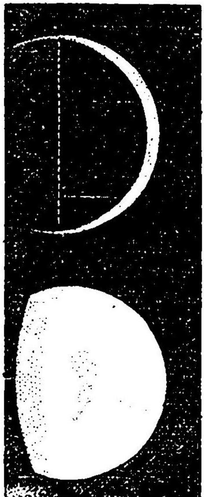
圖之盈將星火
