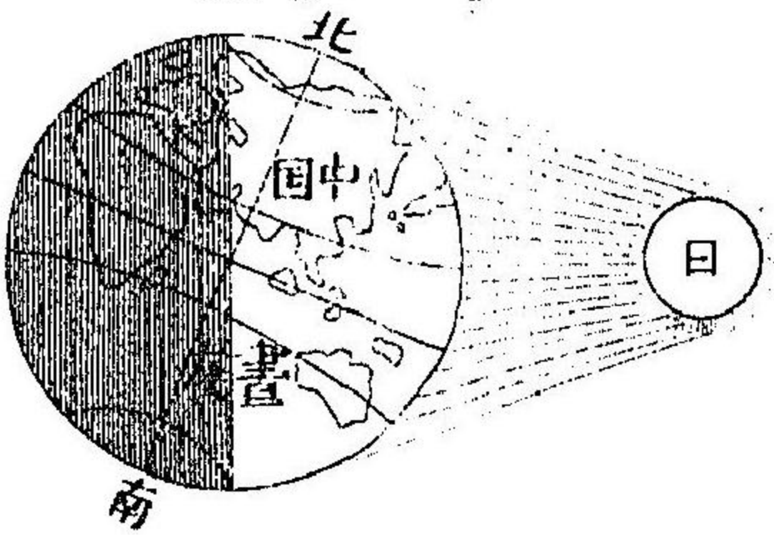
地球分日夜圖
