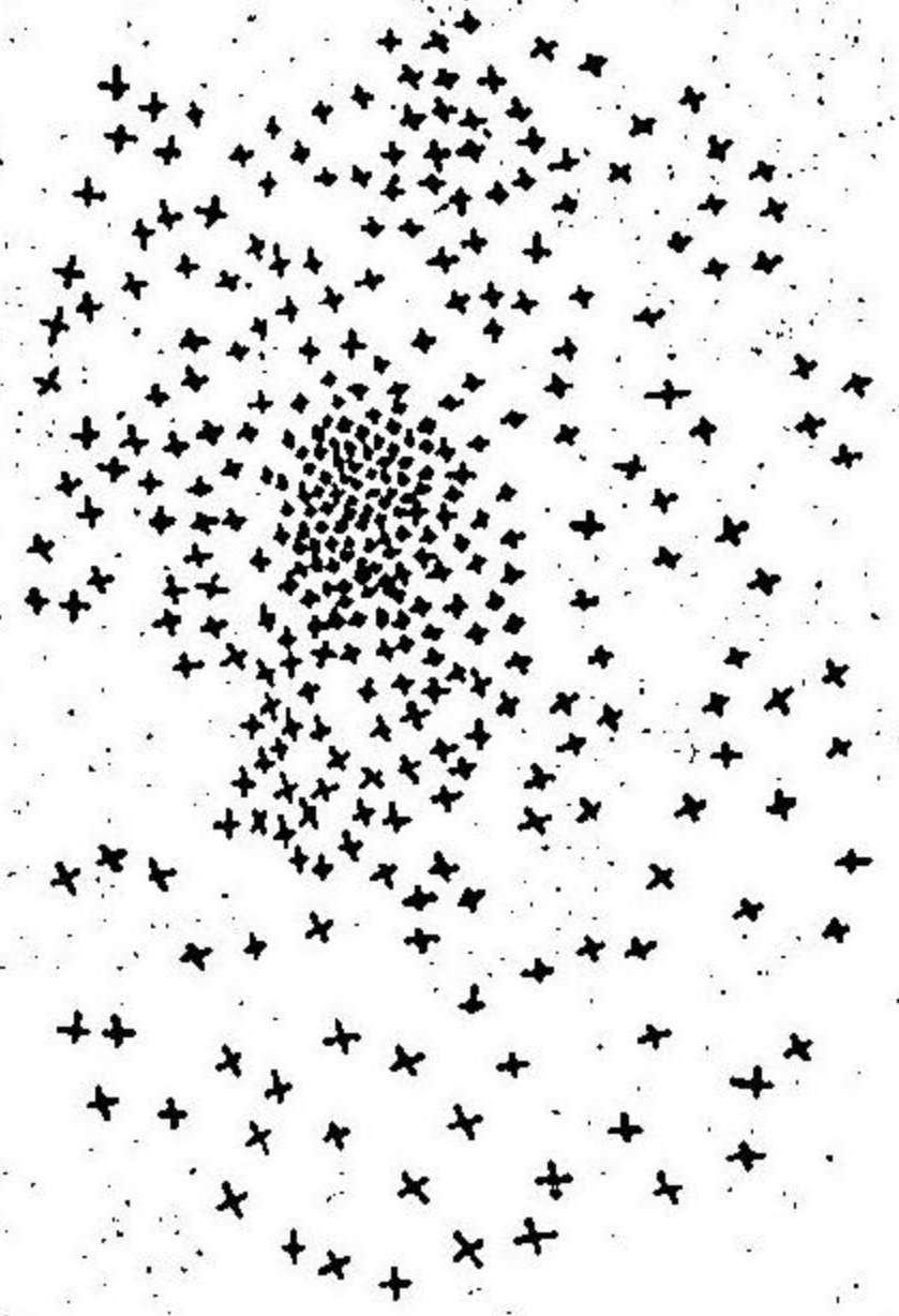
天河眾星圖 用千里鏡所見如此
