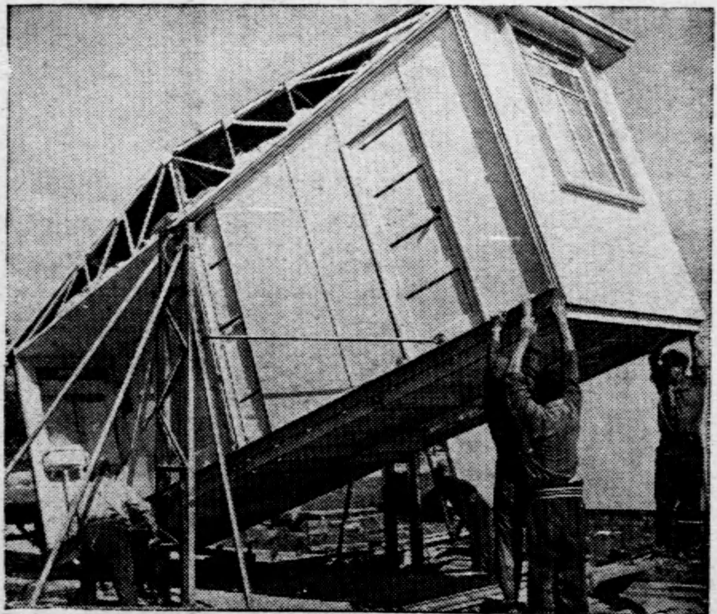
在英國大量建築的鋁質家屋。先部分的裝好了，再運到目的地。其壽命可達四五十年。包括一個起居室二間臥室，澡房及廁所。面積六二〇立方尺。圖上所示是廚房和浴室正在裝置中。
