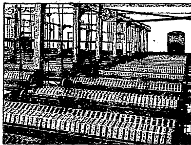
中國棉紗廠
