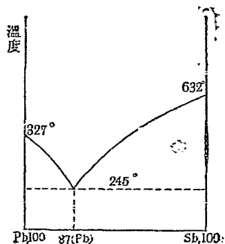
圖 54. 鉛錫系之融點曲線
