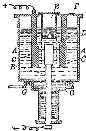
圖 51. 鈉之製法
