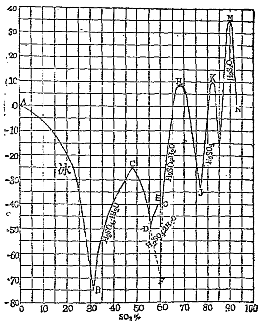
圖 56. 三氧化硫水系之融點曲線
