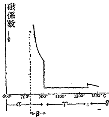
圖 68. 純鐵之磁分析
