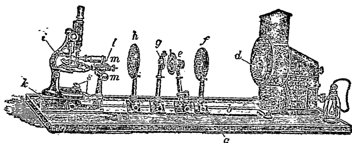
圖 49. 度外顯微鏡
