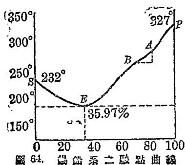
圖 61. 錫鉛系之融點曲線
