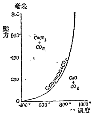
圖 60. 碳酸鈣之離解壓
