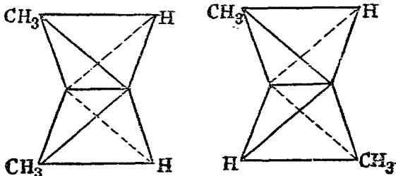
圖 42. 雙鍵結合
