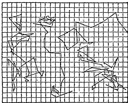
圖 50. 勃朗 運動
