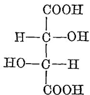
右旋酒石酸 d-tartaric acid
