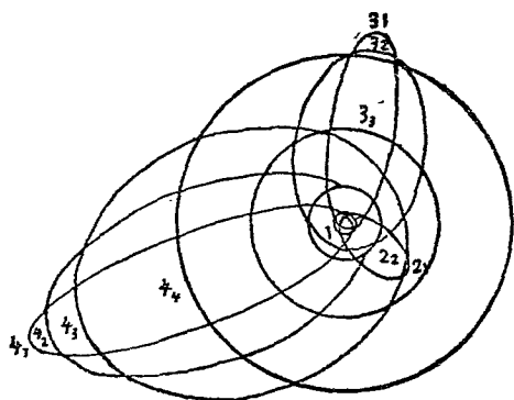
圖7B. 核外電子
