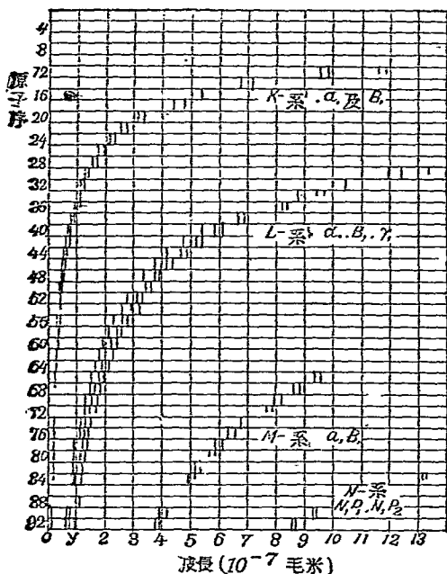
圖 70 波長
