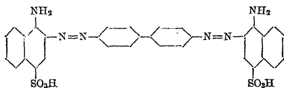
剛果紅之結構式
