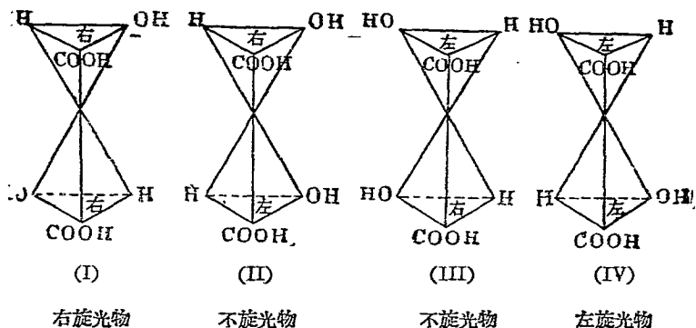
圖 44. 酒石酸異構物之立體結構
