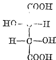
左旋酒石酸 l-tartaric acid
