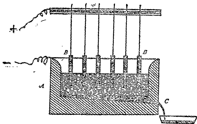
圖 62. 鋁之製法
