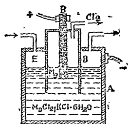
圖 61. 鎂之製法
