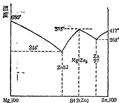
圖 55. 鎂鋅系之融點曲線
