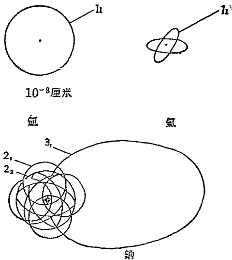
圖71. 原子之結構
