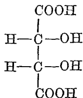
消旋酒石酸 meso-tartaric acid
