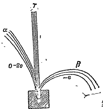
圖 69. 放射線
