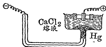
圖 59. 製鈣
