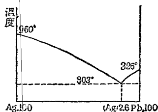
圖 58. 銀鉛系合金
