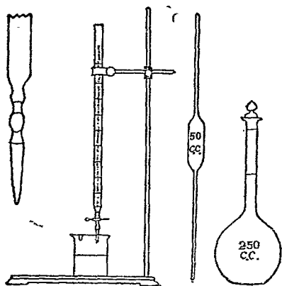
圖 53. 滴管 移液管 量瓶 時用滴管 (burette). 又
