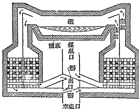
圖 66. 平 爐
