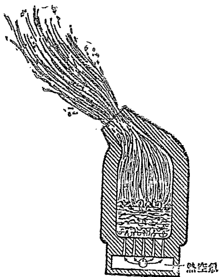
圖 65. 迴轉爐
