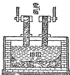
圖 67. 電製鋼法 置銑鐵於電爐，通強電流而熱之，鐵中所含之硫、磷等，與滲於爐內之碳酸鎂等化合，成礦滓而淨。
