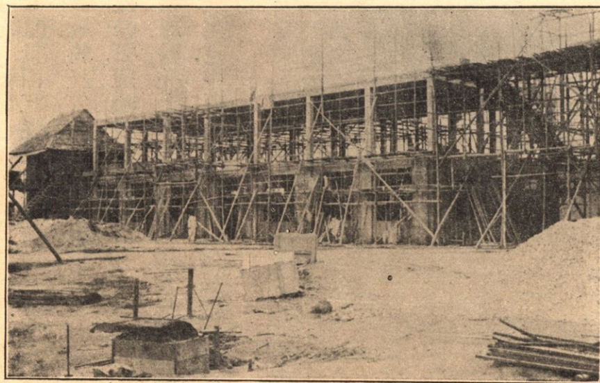
建築中之工學院機械系製圖室及材料實驗所
