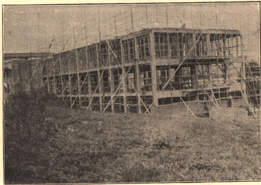
舍宿生女之中築建
