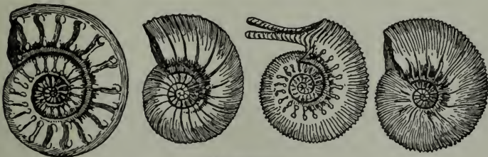
AMMONITES.
