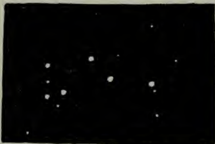
FIG. 8. THE PLEIADES.
