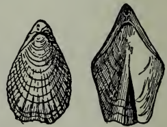
TEREBRATULINA.
