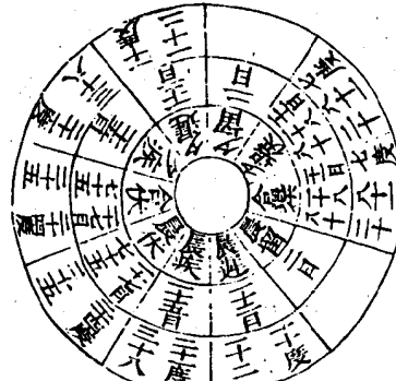
辰星伏見終圖
