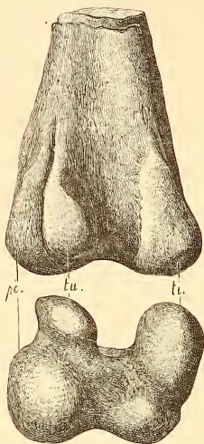
FIG. 555. — Portion inférieure du fémur d'un dinosaurien, vu par derrière, et sur la face distale, au 1/4 de grandeur : tu. tubérosité qui sépare la facette tibiale ti. de la facette péronienne pc. — Donné par le petit séminaire de Beauvais. Gisement inconnu.
