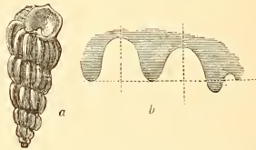
FIG. 201. — Cochloceras Fischevi : a. coquille; b. cloison (M. Fischer, d'après de Hauser). — Keuper d'Aussee.
