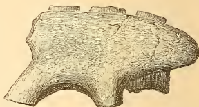
FIG. 510. — Sacrum composé de trois vertèbres; il est en grande partie caché par l'ilion, au 1/10 de grandeur. — Même gisement.
