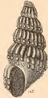
FIG. 188. — Turritites costatus aux 2/5 grandeur. — Cénomaniens de Rouen. Collection d'Orbigny.
