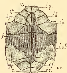
FIG. 550. — Plastron de jeune Testudo tabulata , gr. nat. : en. ento-plastron ; ép. épi-plastron ; hypo. hypo-plastron ; xi. xiphi-plastron ; é.g. écaille gulaire ; é.p. éc. pectorale ; é.h. éc. humérale ; é.ab. éc. abdominale ; é.f. éc. fémorale ; é.c. éc. caudale ; f. grande fontanelle. — Époque actuelle. Collect. d'anat. comparée.
