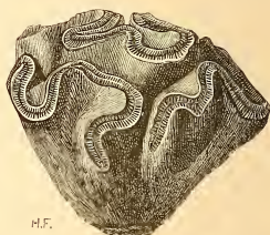
FIG. 55. — Lobophyllia ( Pachygyra ) labyrinthica , au 1/5 de gr. (d'après Michelin). — Turonien des Corbières.
