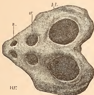
FIG. 289. — Crâne du Cyamodus rostratus , vu en dessus, à 1/4 de grandeur. Il doit être incomplet antérieurement. Mêmes lettres. — D'après le moulage d'un échantillon du Muschelkalk de Bayreuth.
