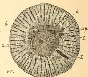
FIG. 155. — Coupe de Barrettia monilifera , au 1/5 de grand; b. b'. fosses dentaires; E. S. piliers correspondant aux oscules; m. a. muscle antérieur; m. p. muscle postérieur. — Craie de la Jamaïque. Collection de l'École des Mines 5 .
