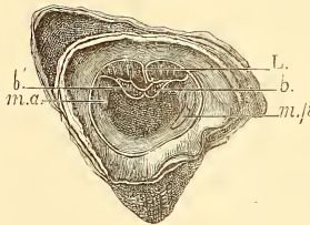
FIG. 150. — Valve droite (inférieure) de Sphaerulites Haeninghausi , au \frac{1}{5} de grandeur (d'après M. Douvillé). — Sénonien de Saint-Mammet. Coll. de l'École des Mines.
