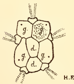
FIG. 74. — Hyboctypus caudatus (d'après Wright). — Bajocien.
