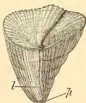
FIG. 154. — Monopleura imbricata , à 1/2 gr.; l. sillon ligamentaire de la valve inférieure; p. point d'attache de cette valve. (M. Fischer, d'après d'Orbigny.) — Urgonien d'Orgon.
