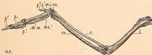
FIG. 548. — Aile gauche d'un aigle au 1/6 de grandeur. m. i. métacarpien interne; m. m. métacarpien médian; m. e. métacarpien externe; p. premières phalanges; p''. secondes phalanges; les autres lettres comme dans les figures précédentes.
