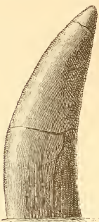
FIG. 519. — Dent de Megalosaurus superbis , grandeur naturelle. — Albien de Bar-le-Duc. Coll. de M. Pierson.
