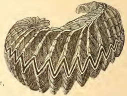
FIG. 114. — Ostrea (Alectryonia) frons , à 1/2 grandeur. — Sénonien de Saintes, Char.-Inf. Collection d'Orbigny.
