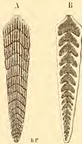
FIG. 5. — Fronicularia pulchra . A. vue extérieure; B. coupe verticale. (Dessin de M. Schlumberger.) — Lias moyen de Nancy.
