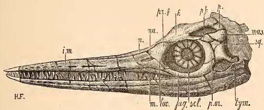
FIG. 271. — Tête de l' Ichthyosaurus communis , vue de profil à 1/10 de grandeur : i.m. inter-maxillaire; m. maxillaire; jug. jugal; n. os nasaux; na. ouverture externe des narines; lac. lacrymal; pr.f. préfrontal; f. frontal; p.f. post-frontal; p.or. post-orbitaire; p. pariétal; scl. pièces osseuses de la sclérotique; sq. squameux; mas. mastoïde; tym. tympanique. — Lias de Lyme Regis. — Collection du Museum.
