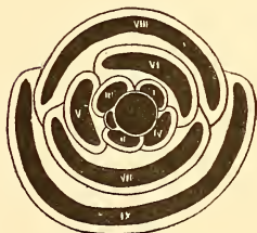
FIG. 17. — Section transverse d'une autre Idalina antiqua , forme A, grandie 28 fois (d'après MM. Munier-Chalmas et Schlumberger).
