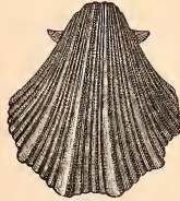
FIG. 116. — Pecten quinquecostatus , grandeur nat. — Craie cénonmienne de Rouen. Collection d'Orbigny.
