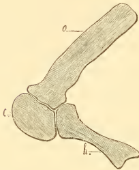
FIG. 552. — Arc thoracique de Megalosaurus , restauré au trait d'après des échantillons du Musée d'Oxford, à 1/20 de grand. : o. omoplate, c. coracoïde, h. humérus (d'après Phillips). — Bathonien de Stonesfield.
