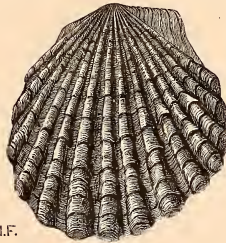
FIG. 117. — Lima 2 proboscidea , au 1/3 de grandeur. — Bajocien de Moutiers. Collection d'Orbigny.
