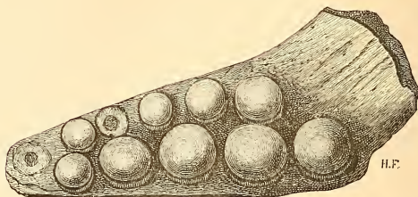
FIG. 261. — Mandibule droite du Lepidotus neocomiensis aux \frac{2}{5} de grandeur, vue sur la face supérieure. — Néocomien de Ville-sur-Saulx, Meuse. Donné au Museum par Cornuel.
