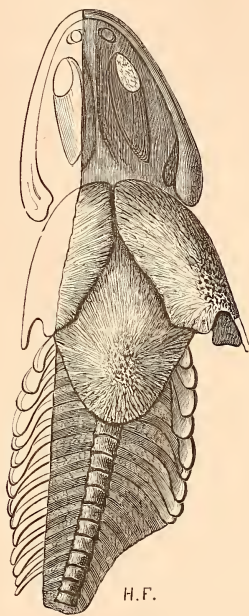
FIG. 265. — Metopias diagnosticus , H. von Meyer, à 1/10 de grandeur, vu sur la face ventrale (d'après un dessin de M. Eberhard Fraas). — Grès du Keuper d'Harweiler. Musée de Stuttgart.
