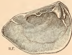
FIG. 121. — Valve de Trigonia Bronni , vue en dedans pour montrer ses dents striées, aux \frac{4}{5} de grand. — Corallien de Glos, Calvados. Coll. d'Oebigny.
