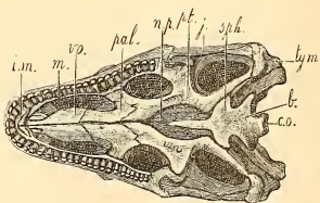
FIG. 565. — Tête d'iguane, vue en dessous, aux 2/5 de grandeur. — Époque actuelle. Collection d'anatomie comparée.
