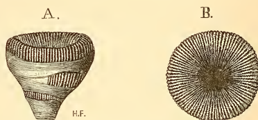
FIG. 50. — Montlivaultia sarthacensis , grandeur nat. A. vu de profil; B. vu en dessus. — Bathonien de Conlie, Sarthe. Coll. d'Orbigny.
