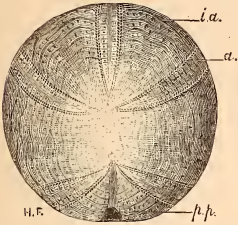
FIG. 83. — Collyrites elliptica , aux \frac{2}{5} de grand., vu en dessus. Les trois ambulacres antérieurs forment le trivium; les deux postérieurs forment le bivium; a. ambulacres; i.a. inter-amb.; p.p. périprocte. — Callovien de Chaumont. Coll. d'Orb.
