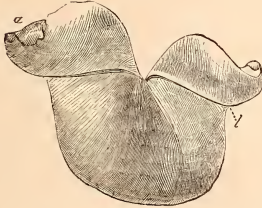
FIG. 156. — Diceras arietinum , à 1/2 grandeur : a. point d'attache de la valve droite, fixée; l. rainure du ligament. (M. Fischer, d'après Woodward.) — Corallien de Saint-Mihiel.
