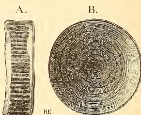
FIG. 242. — Corps d'une vertèbre de Lamna , aux \frac{2}{5} de grandeur. A, vu de profil; B, vu en avant. — Cénomannien du Havre (?). Collection du Museum.
