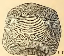
FIG. 245. Dent de Ptychodus decurrens , vue en dessus, grandeur naturelle. — Craie du comté de Kent. Collection du Museum.
