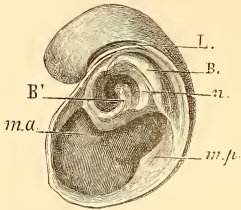
FIG. 142. — Valve droite de Diceras arietinum , à 1/2 grand. (d'après M. Douvillé). — Corallien de Saint-Mihiel. Coll. de l'École des Mines.
