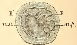
FIG. 153. — Valve droite (inférieure) d' Hippurites bioculatus , aux \frac{5}{4} de grandeur (d'après M. Douvillé). — Sénonien des Bains de Rennes. Collection de l'École des Mines.
