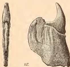
FIG. 265. — Dent pharyngienne d' Ancistrodon splendens , grandeur naturelle, vue de côté et de face pour montrer combien elle est comprimée. — Crête d'Arvert (Charente-Inférieure). Donné au Muséum par le docteur D. Chevallier.
