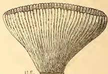
FIG. 53. — Rhipidogyra flabellum , au 1/5 de grandeur. — Corallien de Châtel-Censoir. Collection d'Orbigny.
