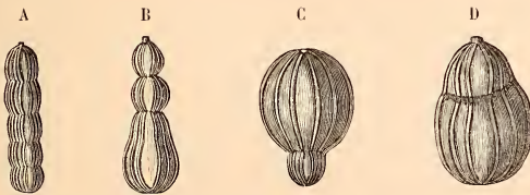
FIG. 11. — Variations de la Nodosaria mutabilis . A. Individu grand 55 fois; B. autre individu grand 50 fois; C. et D. autres individus grands 80 fois (d'après Terquem). — Oolite de Fontoy.
