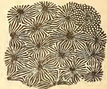
FIG. 40. — Même espèce, calices un peu usés, grandis (d'après Edwards et Haime). — Bajocien de Dundry.
