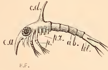
Fig. 240. — Zoé du Carcinus menas 2 , grandi 40 fois : c.a. corne antérieure; c.d. corne dorsale; p. grandes pattes munies de cirrhes; p.r. pattes rudimentaires; ab. abdomen; tel. telson. — Vivant dans la mer à Concarneau.
