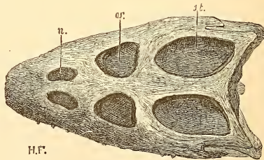
FIG. 288. — Crâne du Simosaurus Guilielmi , vu en dessus, à 1/4 de grandeur : n. narines; or. orbite; s.t. fosse sus-temporale. — Muschelkalk de Lunéville. Collection du Museum.
