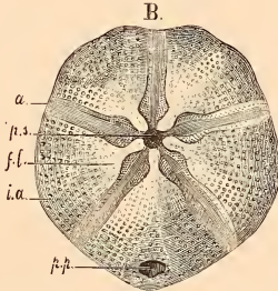
FIG. 85. — Pygurus rostratus , à \frac{1}{2} grandeur. A. vu en dessus; B. vu en dessous; p.p. périprocte; p.s. péristome; a. ambulacres; i.a. inter-ambulacres; fl. rosace appelée floscelle, formée par les dilatations des ambulacres appelées phylloides; g. trous génitaux. — Néocomien de Sainte-Croix. Coll. d'Orbigny.
