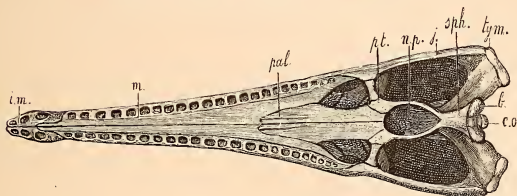
FIG. 565. — Tête du Metriorhynchus Blainvillei , vue en dessous, à 1/8 de grandeur. — Oxfordien du Calvados.
