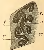
FIG. 169. — Nerinea Clio , aux 2/5 de grandeur (d'après d'Orbigny). — Corallien de Saint-Mihiel.
