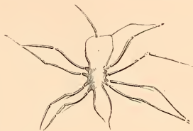
FIG. 258. — Larve d'un crustacé décapode décrite sous le nom de Phyllosoma priscum (d'après Seebach). — Pierre lithographique de Solenhofen
