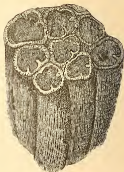
FIG. 129. — Groupe d' Hippurites organisans , aux \frac{2}{5} de grandeur. — Turonien du Beausset. Collection d'Orbigny.
