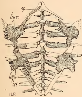
FIG. 552. — Restauration de la Proto-sphargis veronensis au 1/24 de grandeur. On voit le plastron et au-dessous de lui les pièces dorsales, le squelette étant dessiné sur la face ventrale : ép. épipastron; hyc. hypo-plastron; hypo. hypo-plastron; xi. xiphi-plastron (d'après M. Capellini). — Scaglia de Valpolicella, Véronais.
