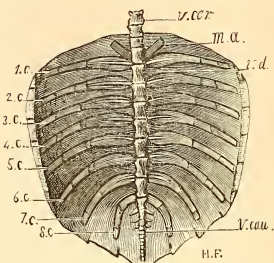
FIG. 549. — Carapace d'une jeune Chelone vue en dessous, grandeur naturelle : v.cer. vertèbres cervicales ; v.d. vertèbres dorsales ; v.cau. vertèbres caudales ; 1.c. , 2.c. , 5.c. , 4.c. , 5.c. , 6.c. , 7.c. , 8.c. les huit paires de côtes qui sont encore bien distinctes les unes des autres ; m.a. pièces de l'arc thoracique. On observe des rudiments des pièces marginales. — Époque actuelle. Collection d'anatomie comparée.
