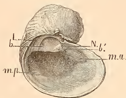
FIG. 159. — Valve gauche de Matheronia Virginia , au \frac{1}{4} de grandeur (d'après M. Munier-Chalmas). — Urganien de Navacelle, Gard. Collection de la Sorbonne.
