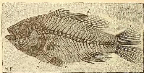
FIG. 260. — Lates Heberti , aux \frac{4}{5} de grandeur. p. pectorales; v. ventrales; d. dorsale; a. anale; c. caudale. — Pisolitique du Mont Aimé. Collection du Museum.
