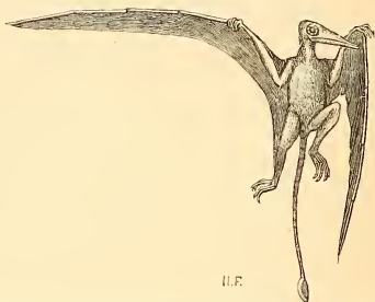
FIG. 544. — Essai de restauration du Rhamphorhynchus Gemmingi , à 1/12 de grandeur. — Pierre lithographique de Solenhofen (d'après M. Zittel).
