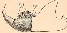
FIG. 597. — Mandibule du Plagiolax Becklesii , grandie \frac{3}{2} (d'après M. Owen). Mêmes lettres. — Étage de Purbeck, près de Swanage.
