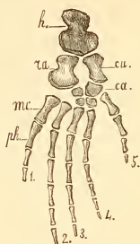
FIG. 504. — Membre de devant gauche du Lestosaurus simus , au 1/16 de gr. : h. humérus ; ra. radius ; cu. cubitus ; ca. carpe ; mc. métacarpiens ; ph. phalanges ; 1. 2. 3. 4. 5. les cinq doigts (d'après M. Marsh). — Craie du Niobrara.
