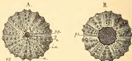
FIG. 50. — Acrocidaris nobilis , aux \frac{4}{5} de grandeur. A. vu en dessus; B. vu en dessous : a. ambulacres; i.a. inter-ambulacres; p.p. périprocte; p.s. péristome; g. pièces génitales; o. pièces ocellaires. — Corallien de la Pointe du Ché. Collection d'Orbigny.
