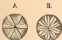
FIG. 105. — Pièces dermiques d' Hemispheeranthos florida , vues en dessus. A. pièce grossie 26 fois; B. autre pièce grossie 47 fois (d'après MM. Terquem et Berthelin). — Lias moyen d'Essey-les-Nancy.
