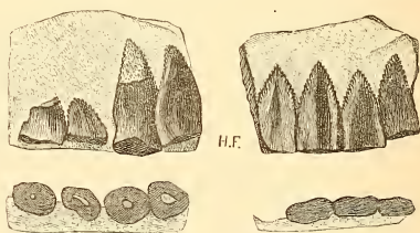
FIG. 518. — Dents de Dimodosaurus , grandeur naturelle, vues de face et en dessous. — Trouvées dans les marnes irisées de la tranchée de Villette, près de Poligny. — Collection du Muséum de Paris.
