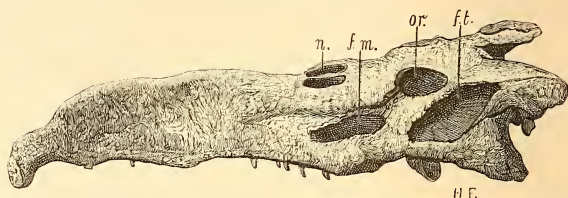
FIG. 568. — Tête du Belodon ( Phytosaurus ) Plueningeri , à 1/8 de grandeur, vu de côté, légèrement de 5/4 pour montrer la position des narines n. ; fosse massétérierne f.m. ; orbite or. ; fosse temporale f.t. — Keuper du Wurtemberg, d'après un moulage envoyé par le Musée de Stuttgart au Museum de Paris.
