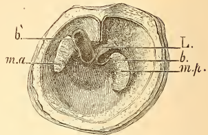
FIG. 149. — Valve droite (inférieure) du Sphaerulites foliaceus , au \frac{1}{4} de grandeur (d'après M. Douvillé). — Cénomaniens de l'île d'Aix. Collection de l'École des Mines.
