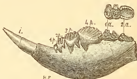
FIG. 591. — Mandibule de Plagiaulax minor , grandie 4 fois : i. incisive ; 1 p. , 2 p. , 5 p. , 4 p. ; les 4 prémolaires ; 1 a. , 2 a. , les arrière-molaires vues de profil et en dessus (d'après Falconer). — Étage de Purbeck, près de Swanage.
