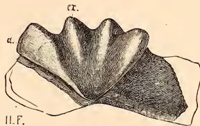
FIG. 251. — Dent inférieure du Ceratodus 2 Kaupi , vue sur la face triturante, aux \frac{2}{5} de grandeur; a. corne antérieure; ex. bord externe. Le dessin de l'os de la mandibule a été complété au trait avec une pièce qui a été recueillie par M. Schlumberger. — Muschelkalk de Mont-sous-Meurthe, Meurthe-et-Moselle. Donné au Museum par M. Roville.
