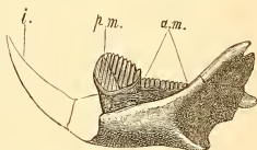
FIG. 592. — Mandibule du Neoplagiaulax cocænus , au double de grandeur : i. incisive ; p.m. prémolaire unique ; a.m. les deux arrière-molaires (d'après M. Lemoine). — Éocène inférieur de Cernay, près Reims.
