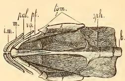
FIG. 560. — Tête de poisson vue en dessous (figure schématique), 1/2 grandeur.
