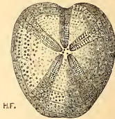
FIG. 100. — Micraster Brongniarti , aux \frac{3}{5} . — Sénonien de Meudon. Donné par moi au Muséum.
