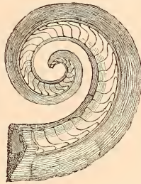
FIG. 151. — Ichthyosarcolites ( Caprinella ) triangularis , valve gauche; la coquille a disparu, laissant visibles les chambres à eau. (M. Fischer, d'après Woodward.) — Cénomaniens de l'île d'Aix.
