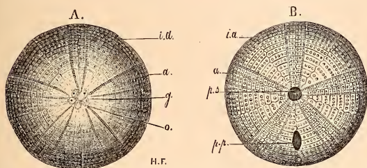
FIG. 51. — Discoidea cylindrica , aux \frac{5}{4} de grand. A. en dessus; B. en dessous. Mêmes lettres. — Cénomaniens du Villard de Laus. Coll. d'Orbigny.
