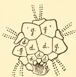
FIG. 71. — Aerosalenia angularis (d'après M. de Loriol). — Jura berinois.
