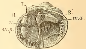
FIG. 145. — Valve gauche de Plagiptychus Aquiloni , aux 2/5 de grandeur (d'après M. Douvillé). — Turonien du Beausset. Var. Collection de l'École des Mines.
