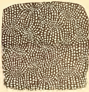
FIG. 59. — Thamnaestrea Defranciana , quelques calices bien conservés, grandis (d'après Edwards et Haime). — Bajocien de Dundry.
