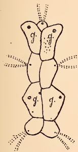
FIG. 80. — Hyboclypus gibberulus (d'après M. Cotteau). — Bathonien.
