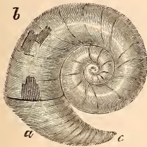
FIG. 150. — Caprina adversa , à \frac{1}{5} de grandeur; a , valve droite fixée par son sommet c ; b , valve libre ou gauche. (M. Fischer, d'après d'Orbigny.) — Cénomaniens de l'île d'Aix 4 .
