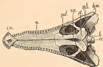
FIG. 566. — Tête du Gompholis crassidens , vue en dessous, à 1/12 de grandeur (d'après M. Hulke). — Wealdien du sud de l'Angleterre.
