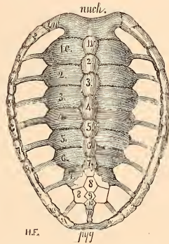
FIG. 555. — Restauration de la carapace de la Chelone Hoffmanni , vue sur le dos, au 1/24 de grandeur. 1 v. à 11 pièces vertébrales; 1 c. à 8 pièces costales; 1 m. à 11 pièces marginales; nuch. pièce nuchale; pyg. pièce pygale (d'après M. Winkler). — Craie de Maestricht.
