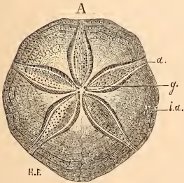
FIG. 85. — Pygurus rostratus , à \frac{1}{2} grandeur. A. vu en dessus; B. vu en dessous; p.p. périprocte; p.s. péristome; a. ambulacres; i.a. inter-ambulacres; fl. rosace appelée floscelle, formée par les dilatations des ambulacres appelées phylloides; g. trous génitaux. — Néocomien de Sainte-Croix. Coll. d'Orbigny.
