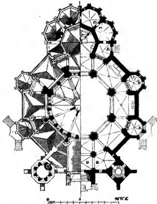
Grundriß der neuen Kirche zu Hünfhaus. AA Vorhalle. B Kapelle. CC Sakristei. DE Orgelbühne.
