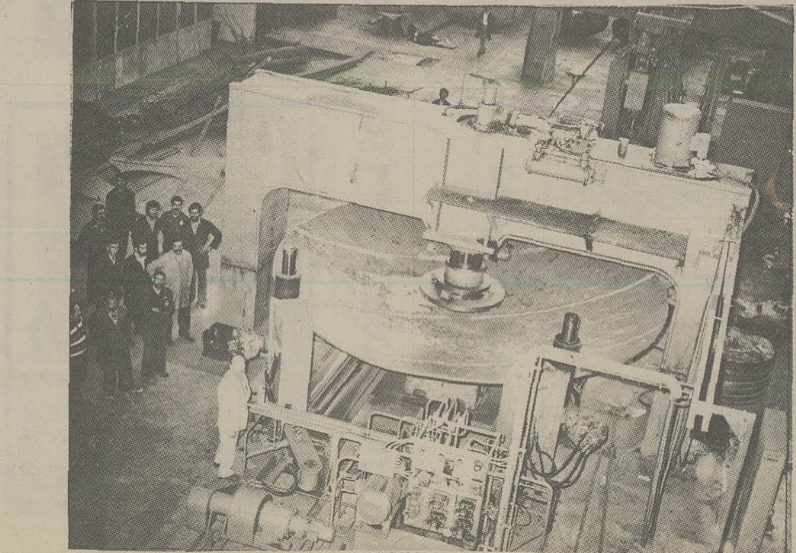
اینجا سالن پر عظمت کارخانجات ماشین سازی اراک مخصوص تولید مخازن بزرگ می باشد در عکس بزرگترین دستگاه ساخت سروه مخازن تحت فشار که در ایران منحصر فرد است دیده میشود. با این دستگاه غول پیکر بدنه و همچنین سروه مخازن از قطر ۸۰۰ تا ۲۹۰۰ میلیمتر و از ورقهای آهن و فولاد ضخامت ۳ تا ۳۲ میلیمتر تولید میشود.
