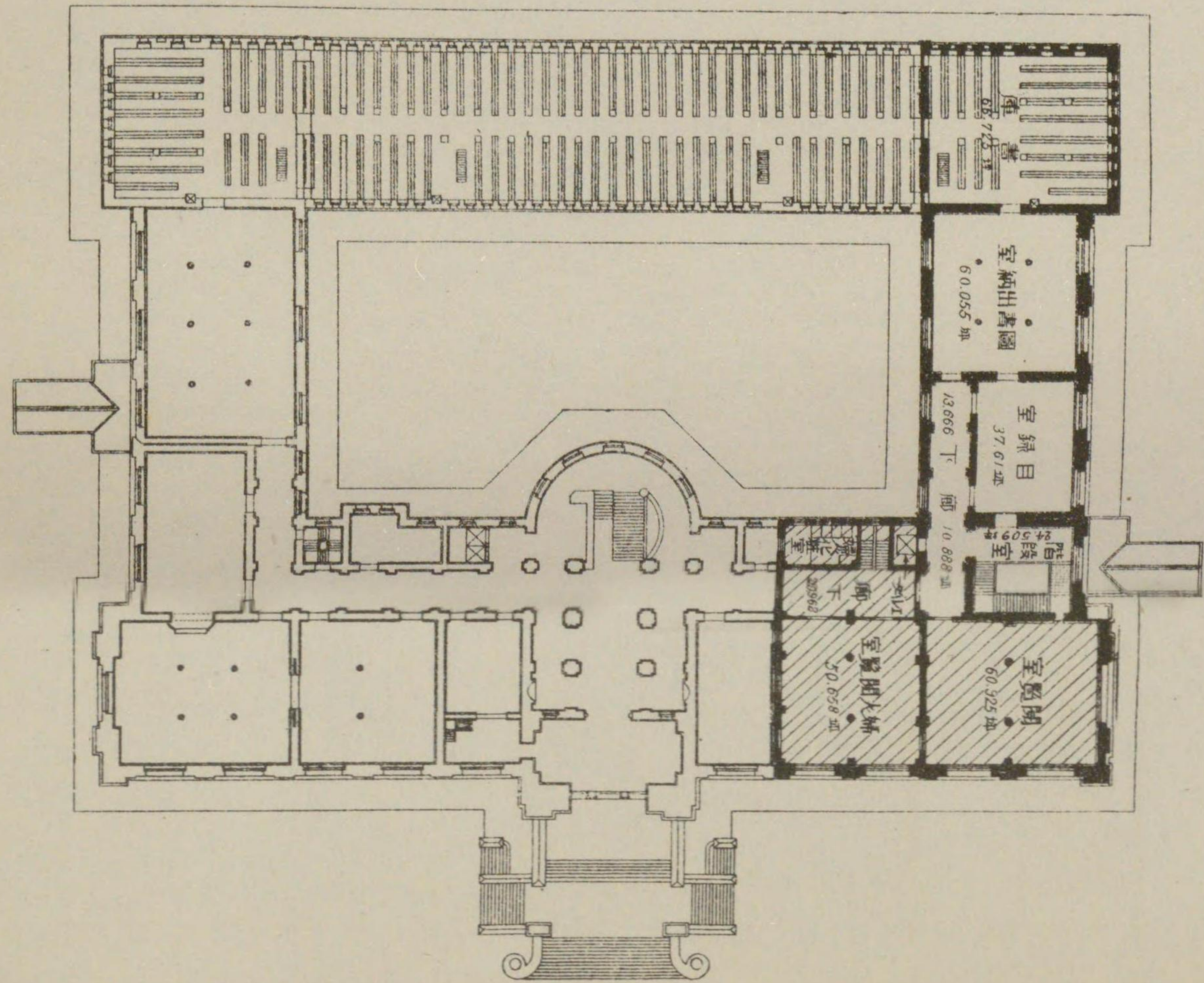
圖面平階二
