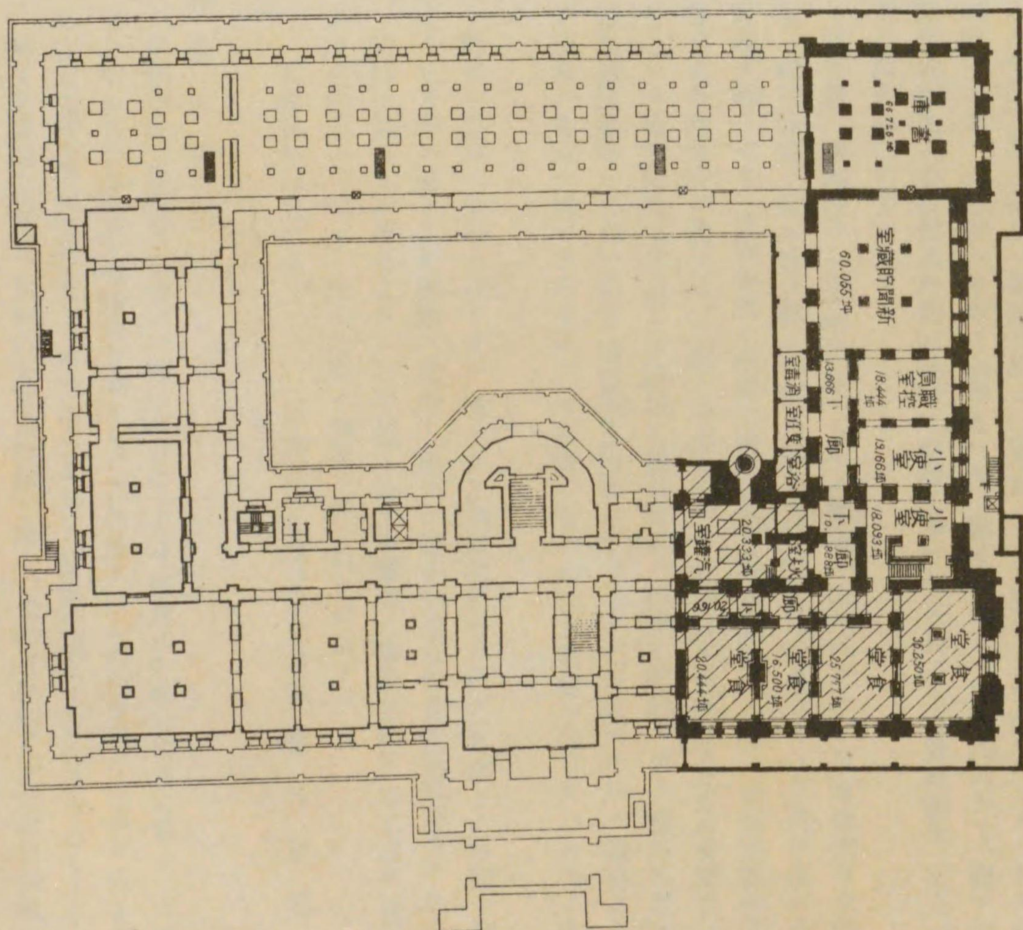
圖面平階地
