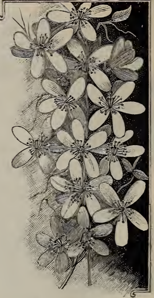
CLEMATIS PANICULATA.
