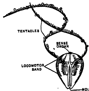
Fig. 588.—Cydippe
