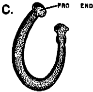
Fig. 766.— Chætoderma
