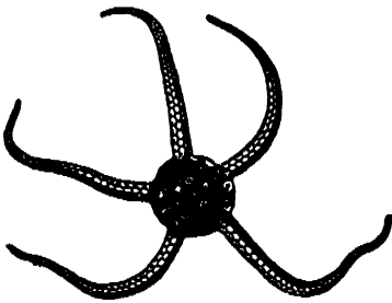
Fig. 669.—A Brittle-Star
