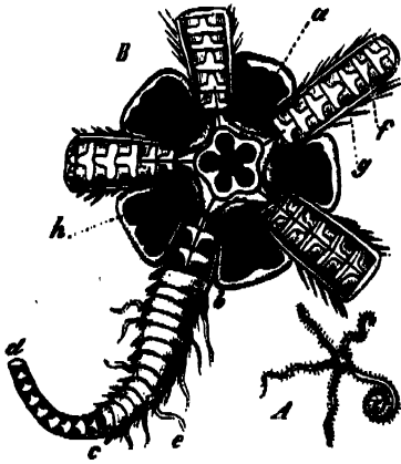
Fig. 820.—Brittle-Star
