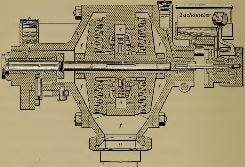
FIG. 43.—Dow TURBINE.
