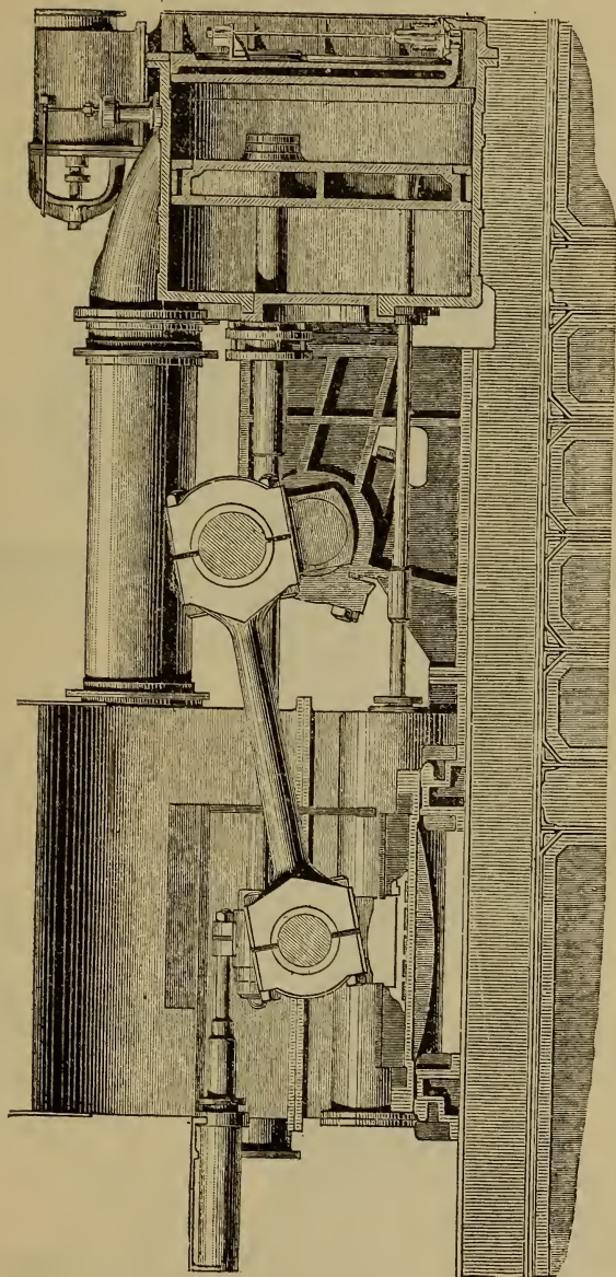
FIG. 12.—ENGINE OF H. M. S. AGINCOURT.
