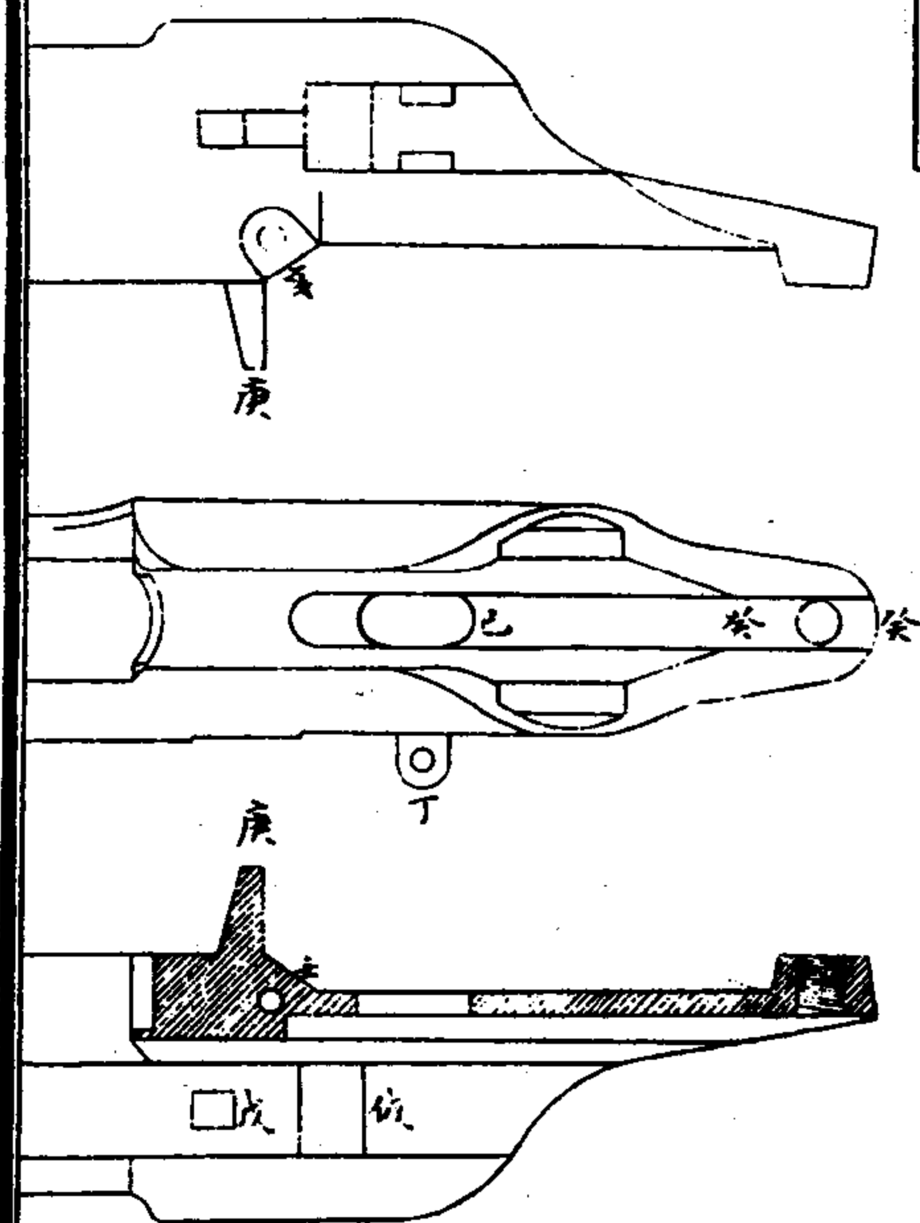
槍圖一機槍
