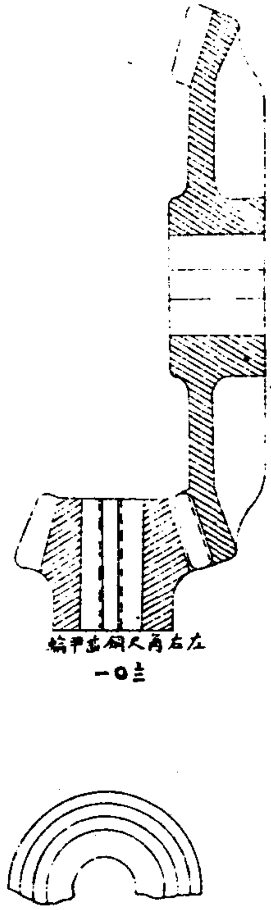
鐵圖三十二
