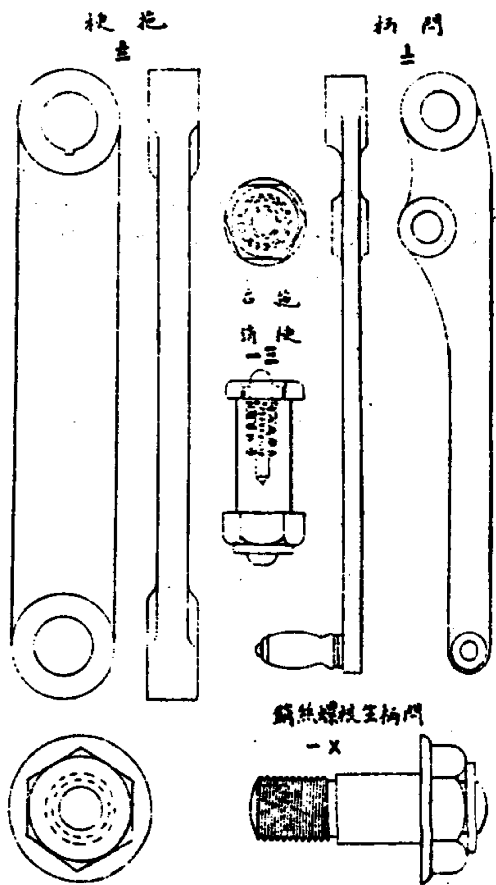
鐵圖六
