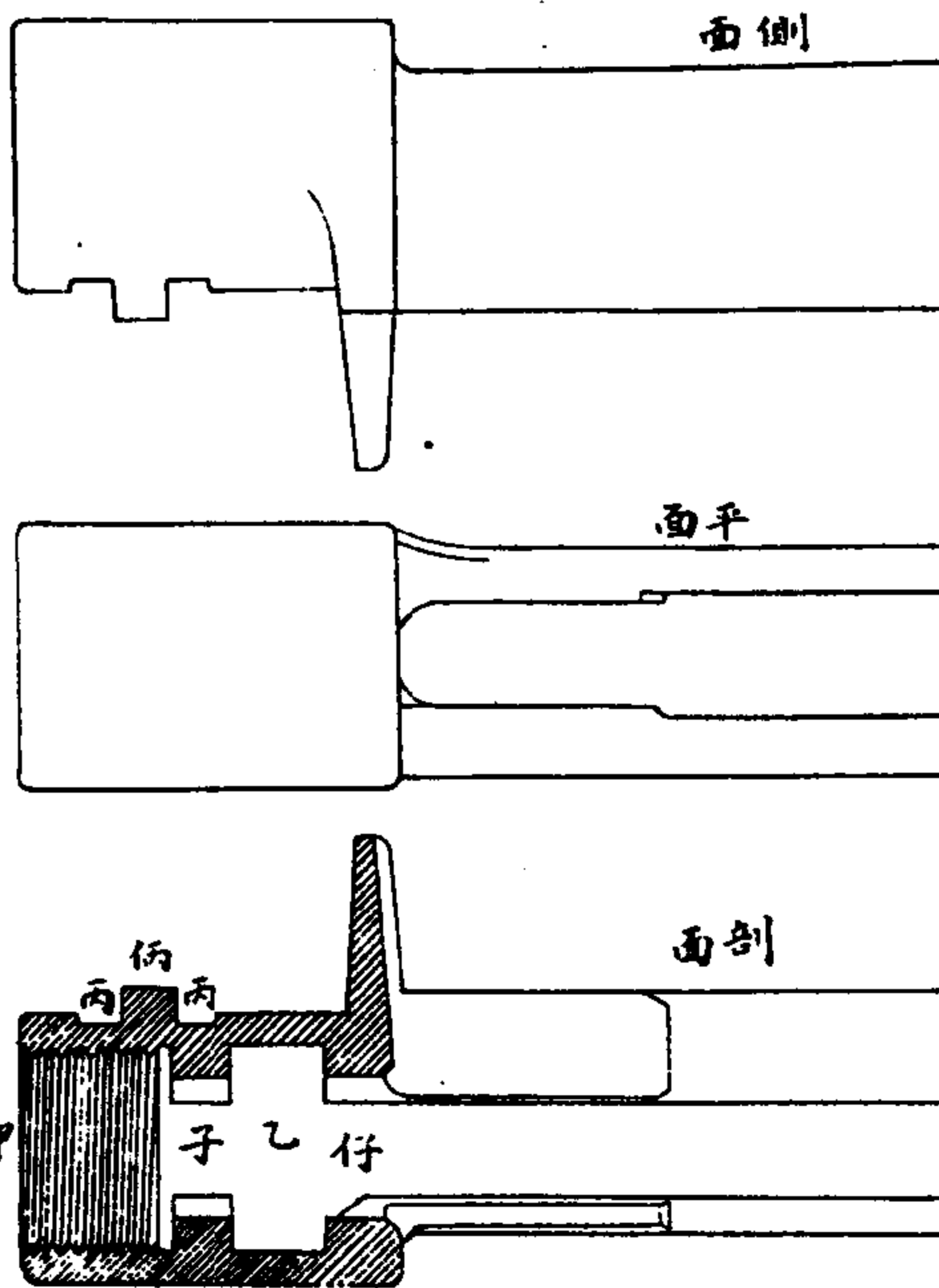
槍機二圖槍
