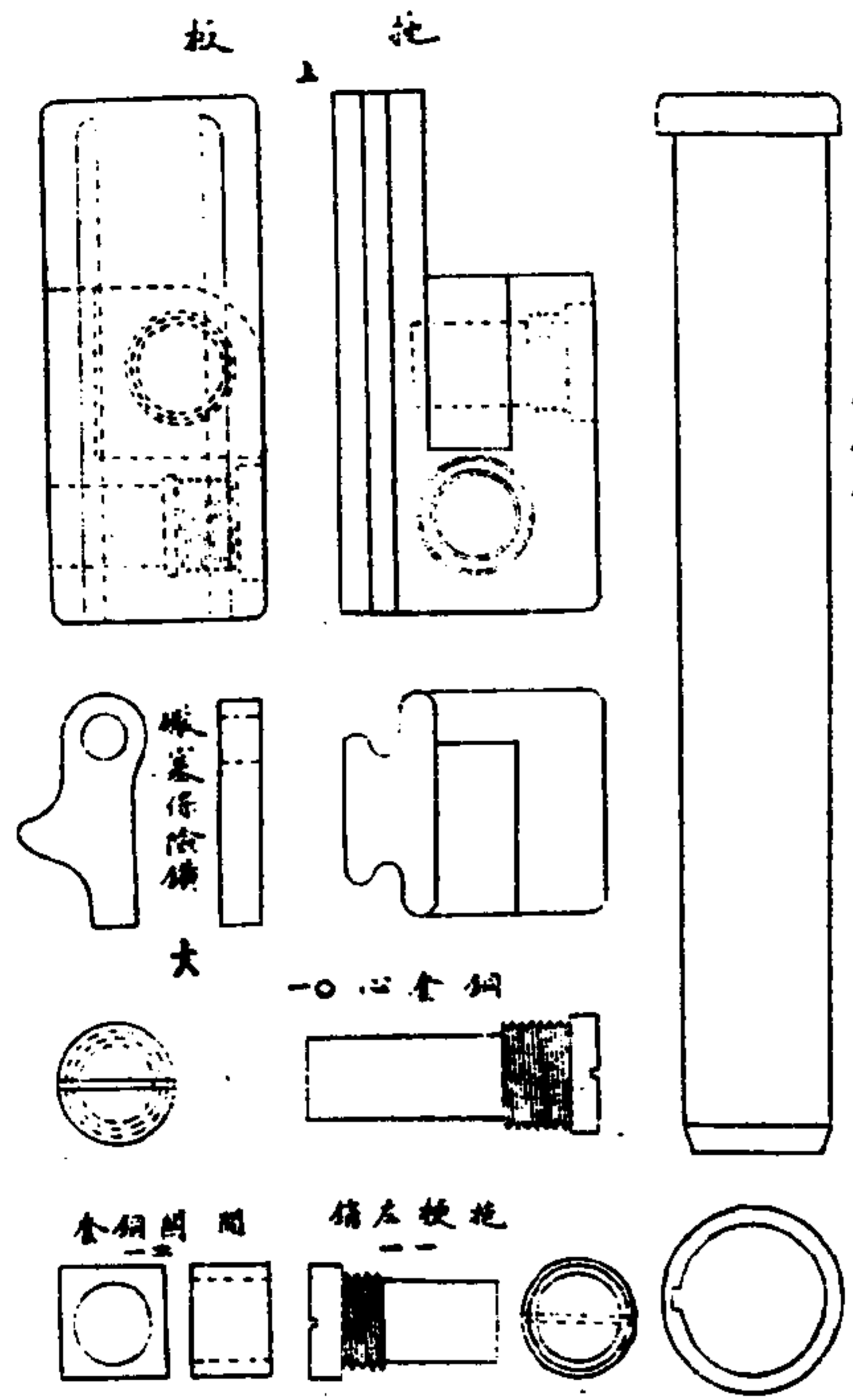
鐵圖五
