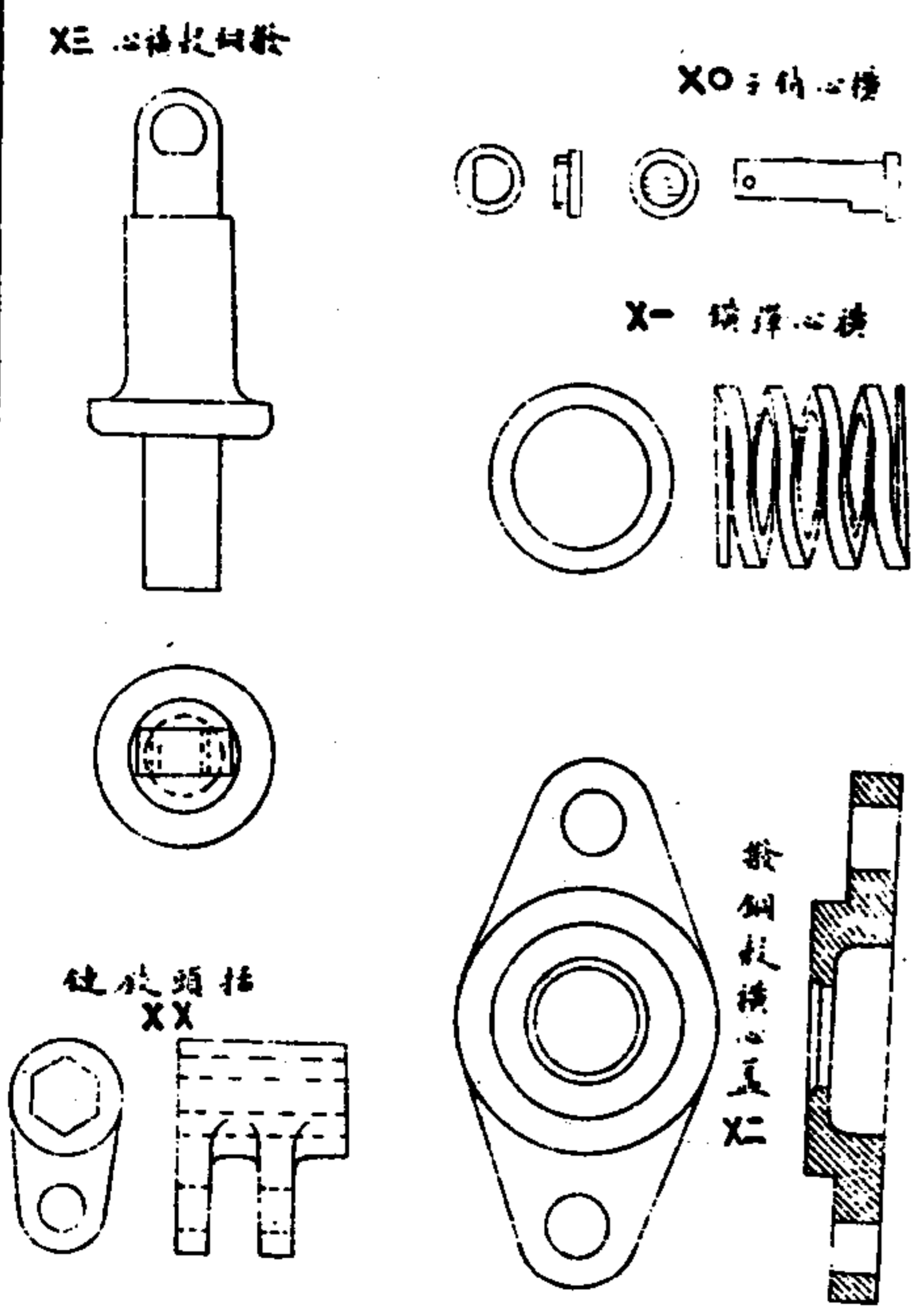
破圖十一
