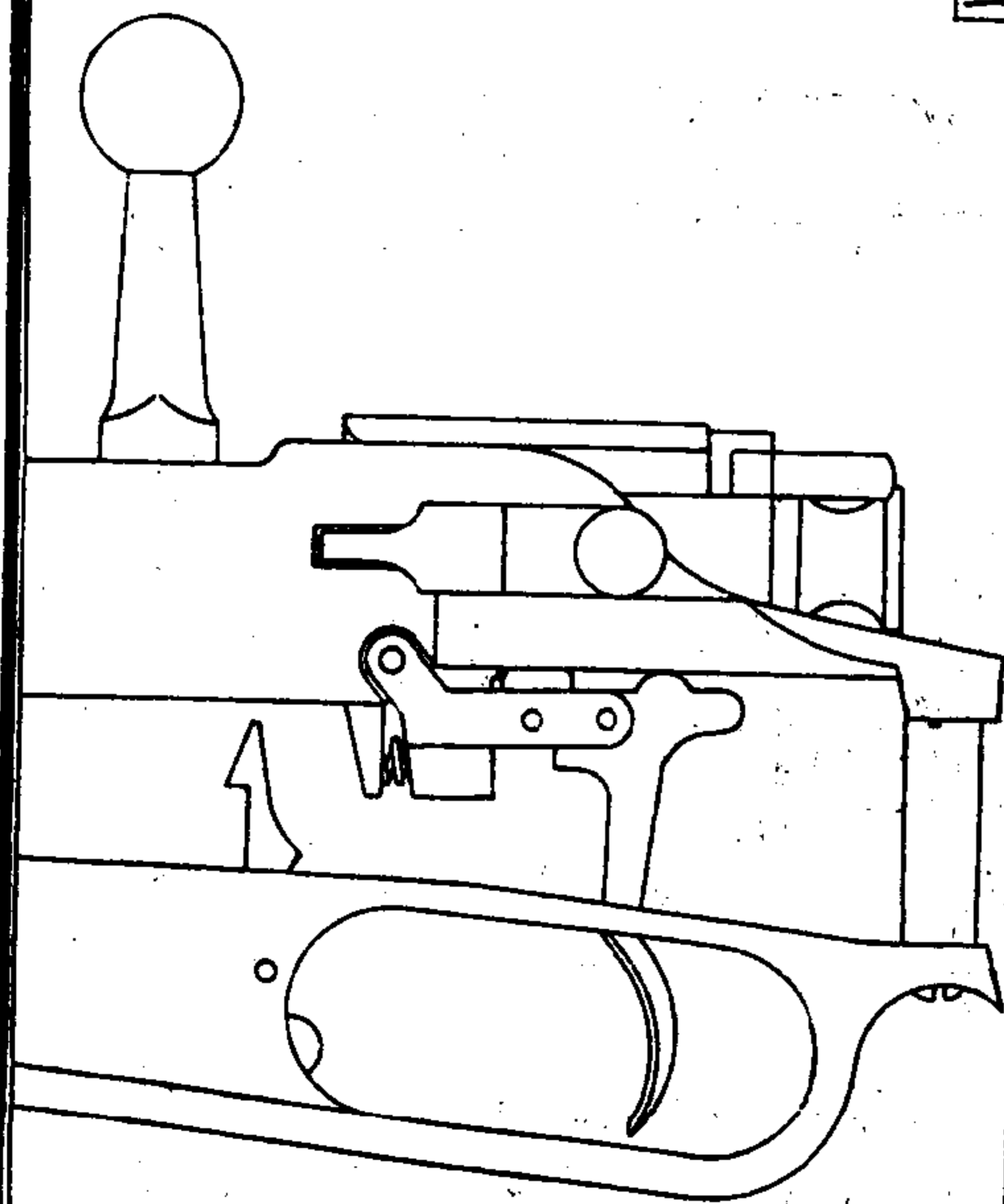
槍圖十一
