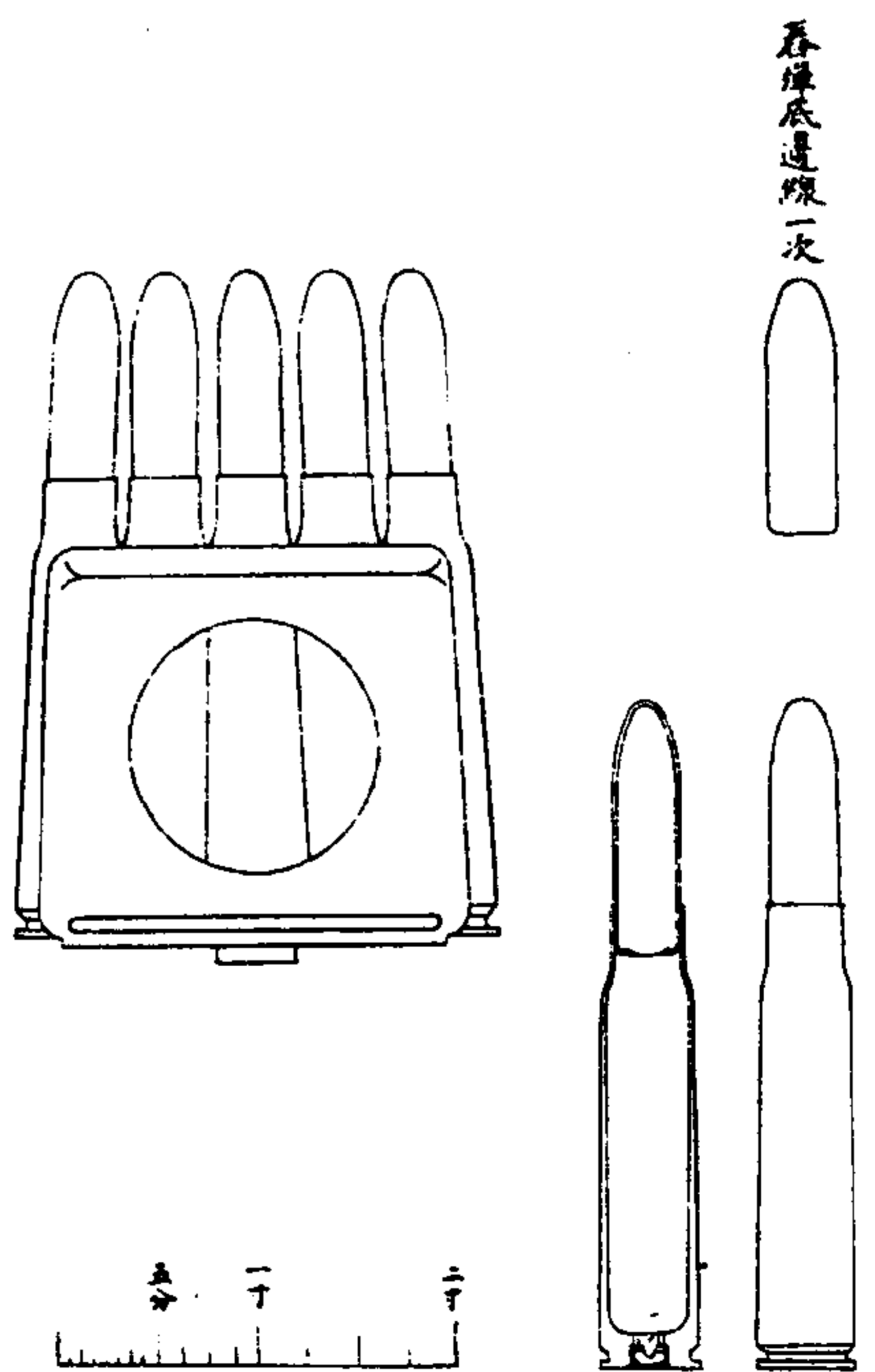
槍子圖四
