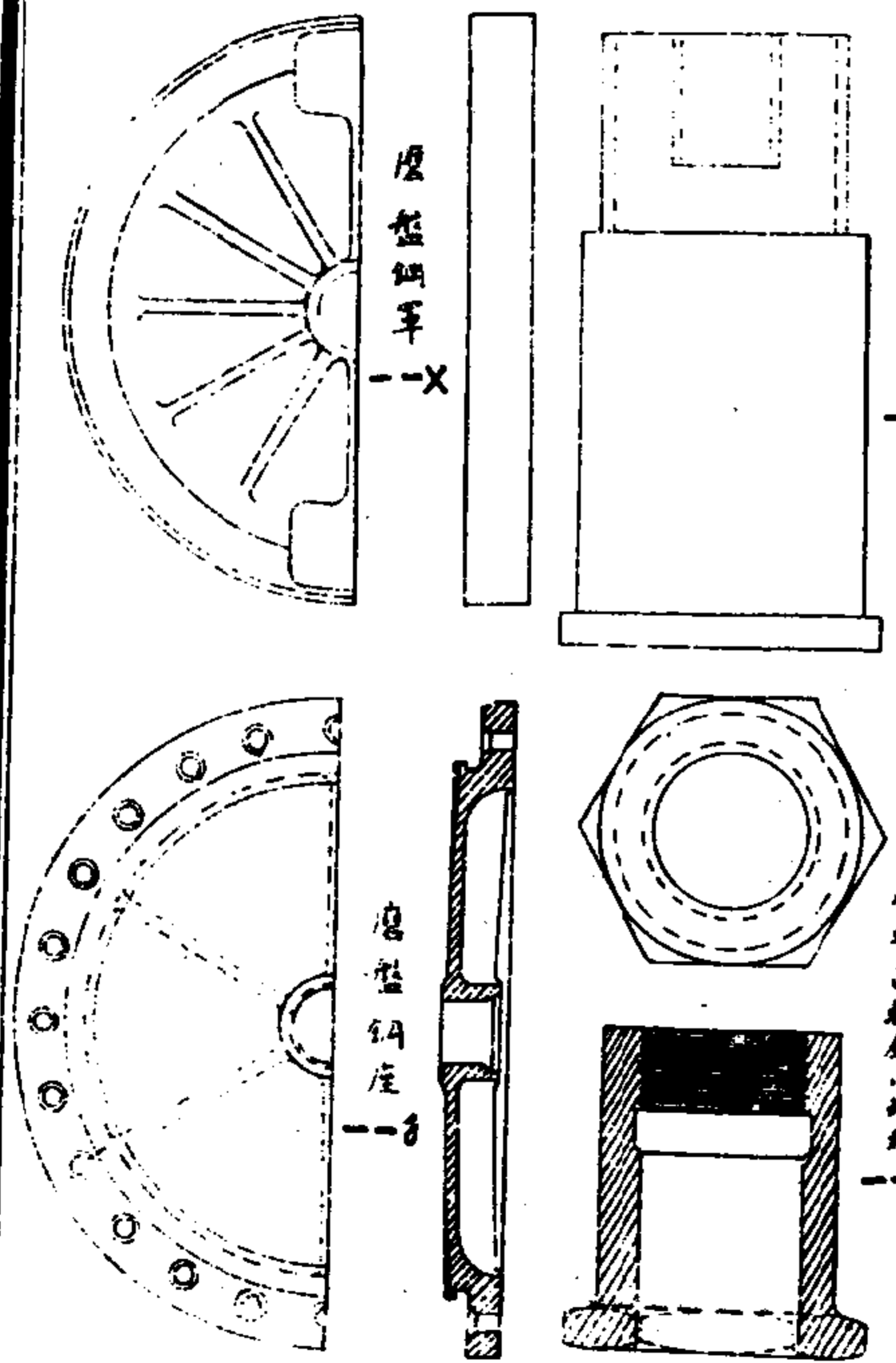
鐵圖三十五
