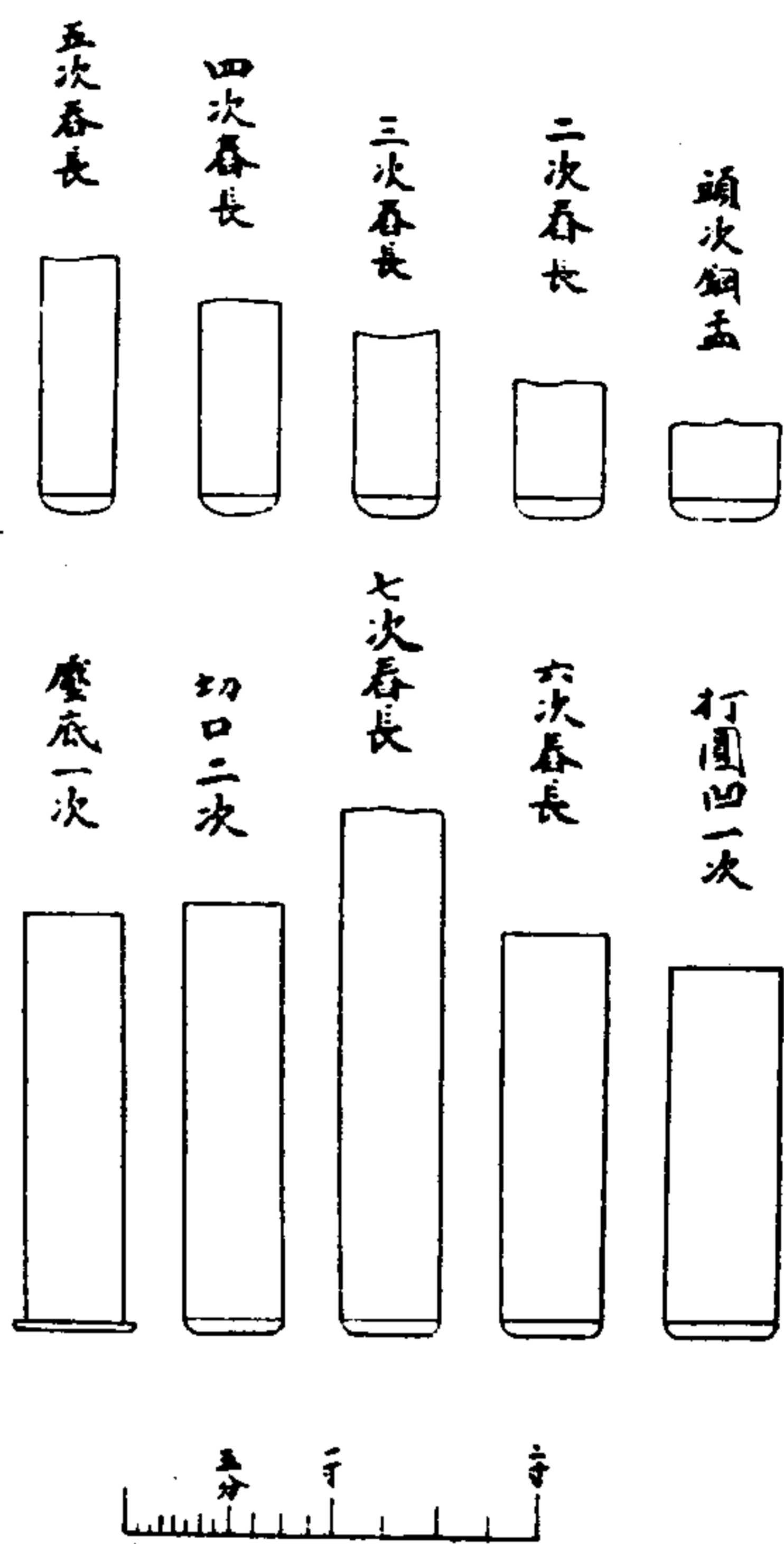
槍子圖六
