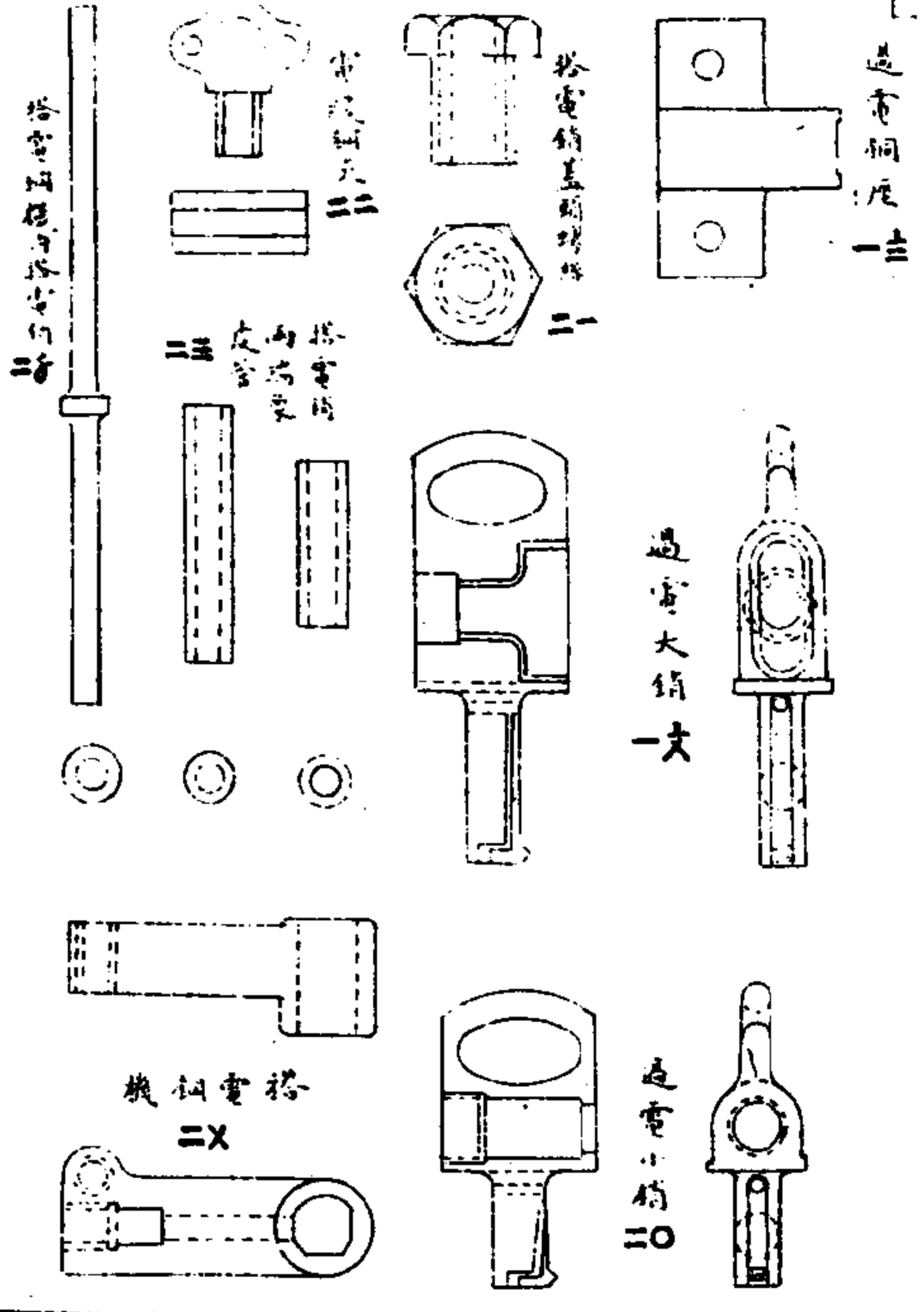
破圖八
